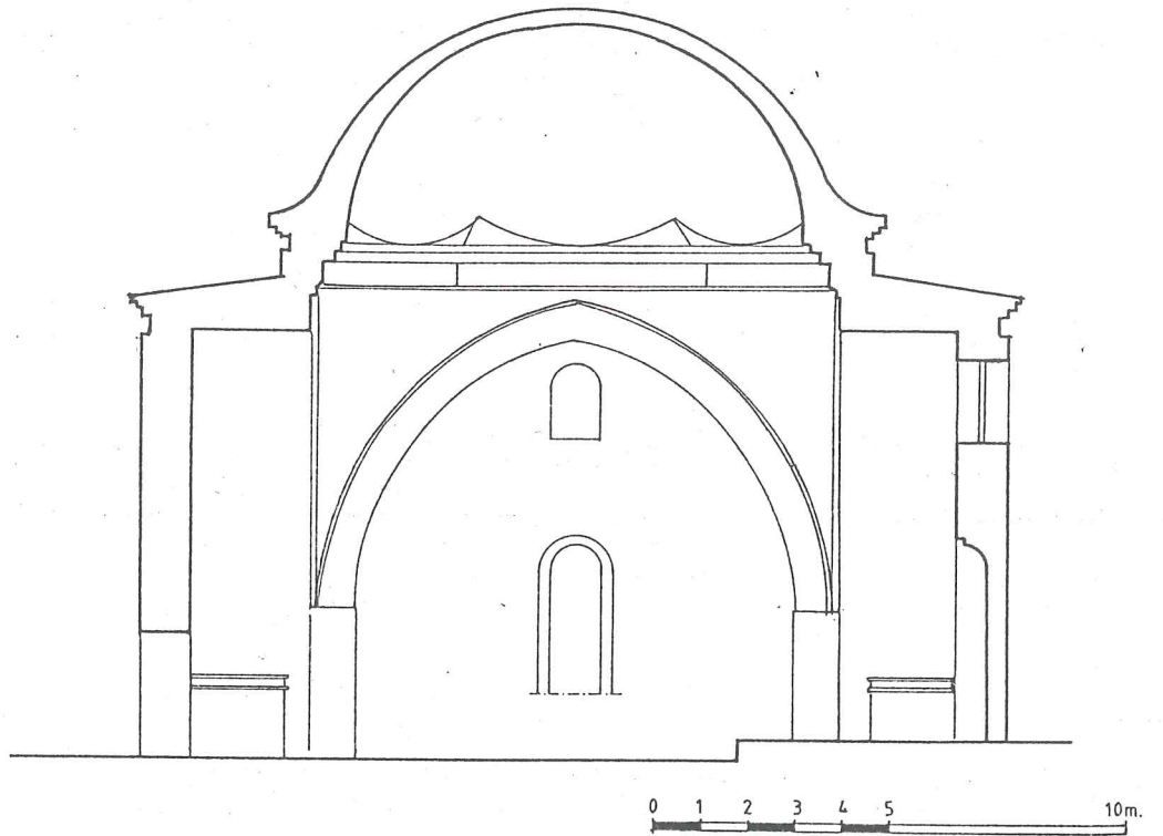
Resim 11- Orhan Gazi Camii Kesiti.
