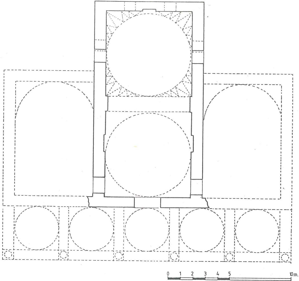
Resim 23- Orhan gazi İmareti Planı
