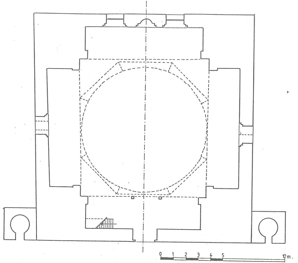
Resim 10- Orhan Gazi Camii Planı.
