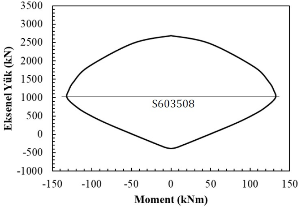
Şekil 3.25 S603508 için kapasite eğrisi
