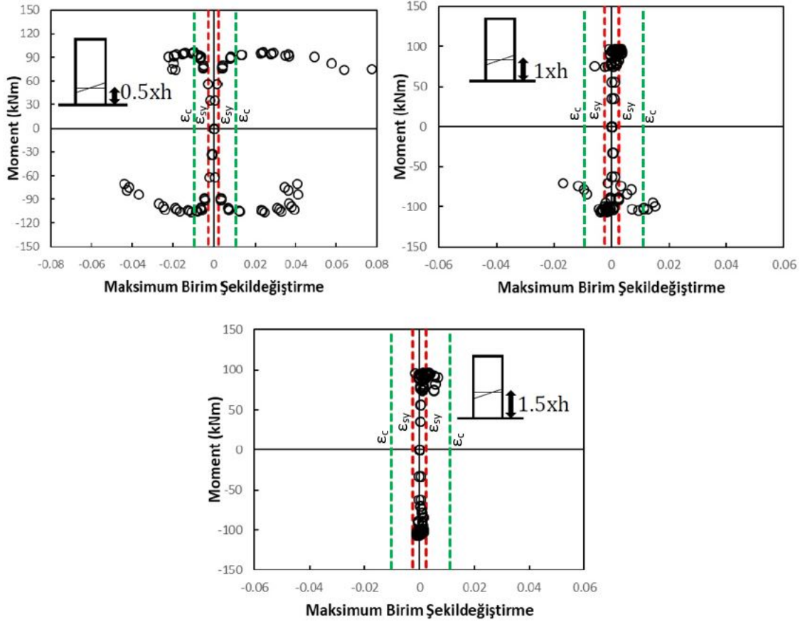
Şekil 4.40 S451006 için farklı seviyelere ait maksimum birim şekil değiştirme diyagramı
