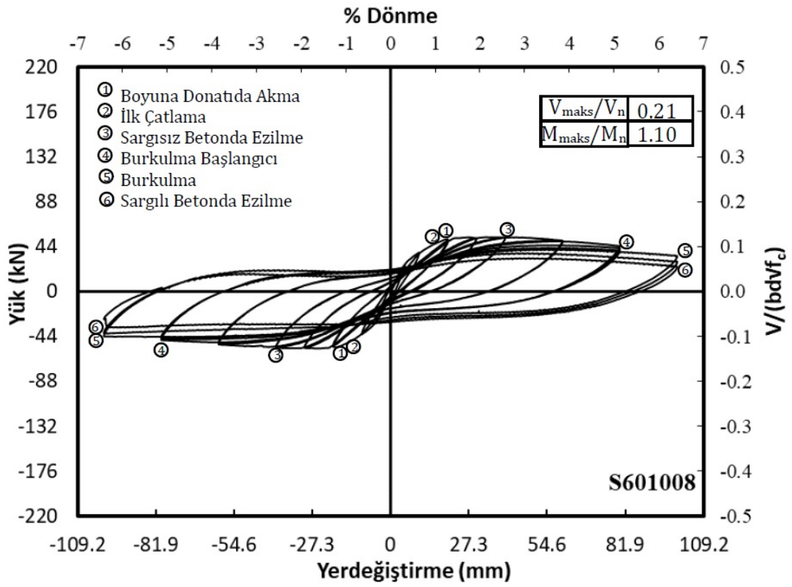
Şekil 3.36 S601008 için yük-yerdeğiştirme ilişkisi
