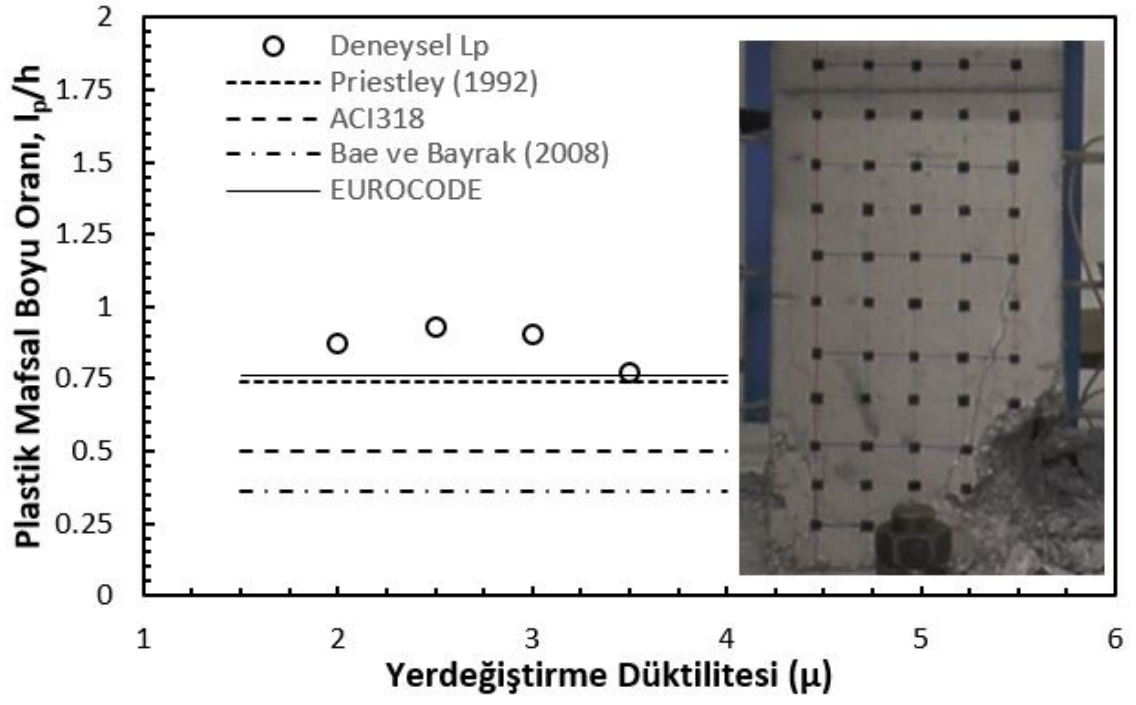
Şekil 4.29 S353508 kolonu için plastik mafsall boyu
