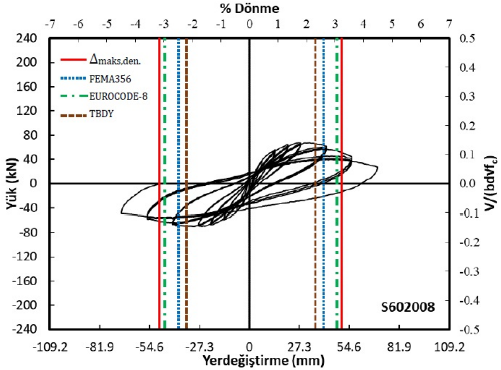
Şekil 5.7 S602008 kolonu için yönetmeliklere göre yerdeğiştirme kapasitesi
