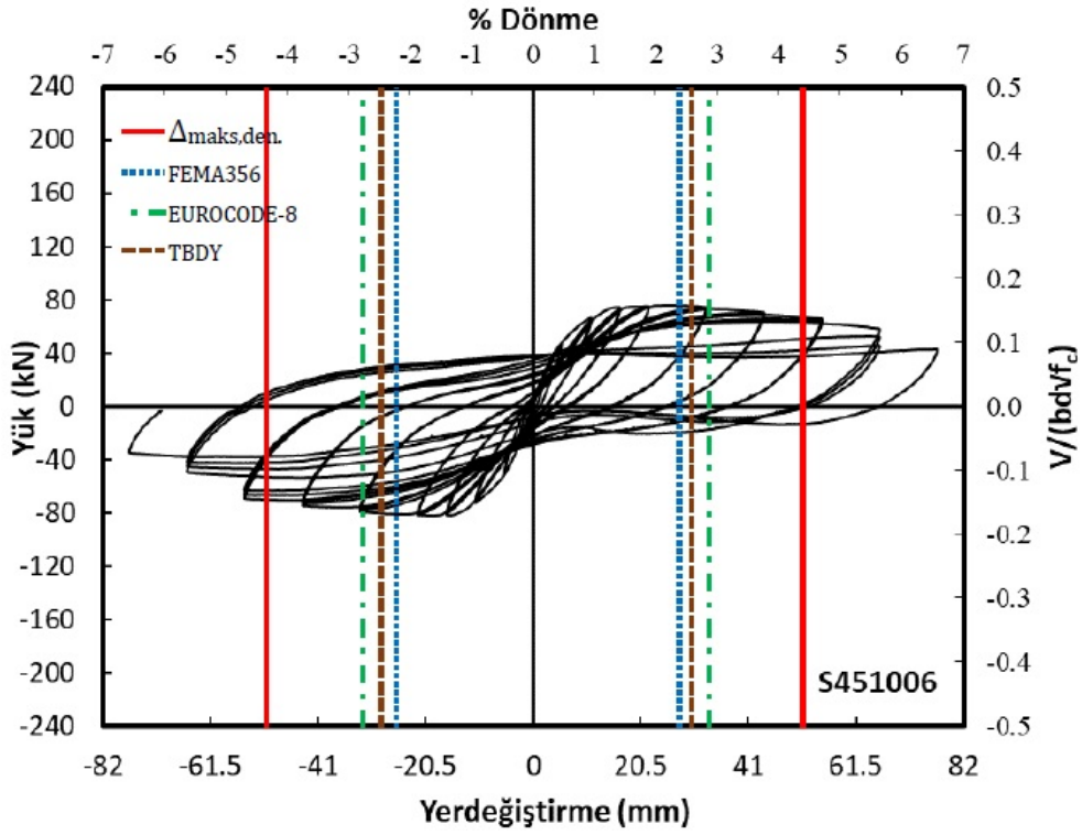
Şekil 5.11 S451006 kolonu için yönetmeliklere göre yerdeğiştirme kapasitesi
