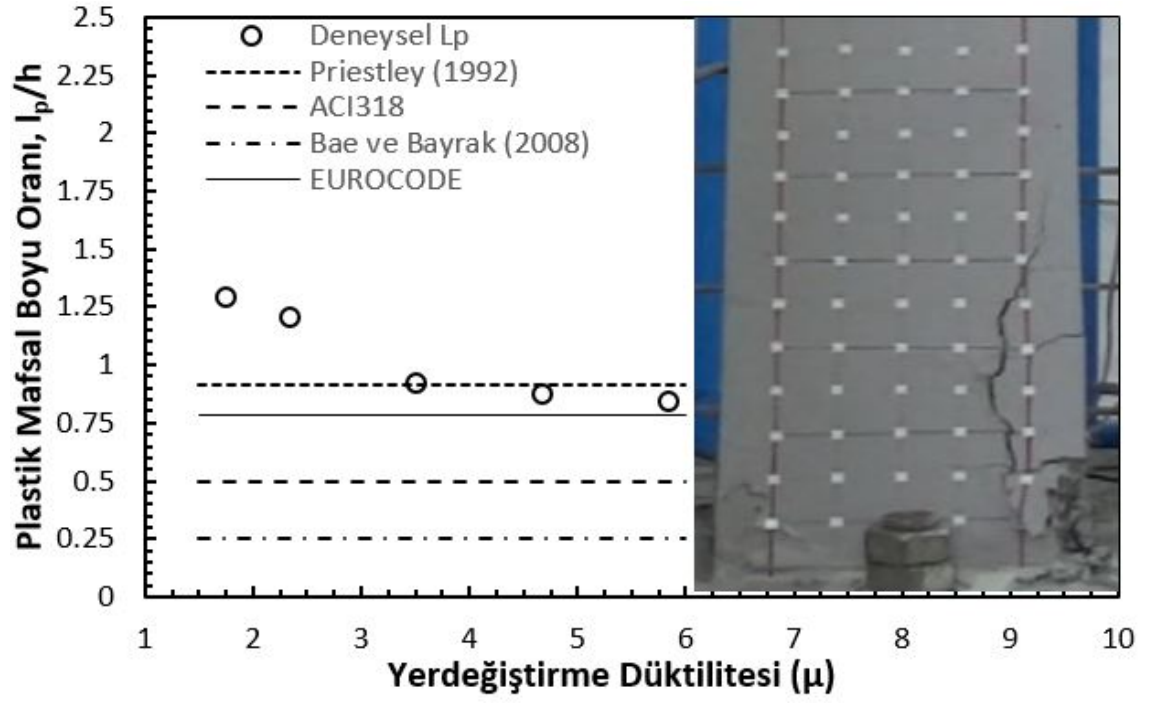
Şekil 4.25 S452008 kolonu için plastik mafsal boyu
