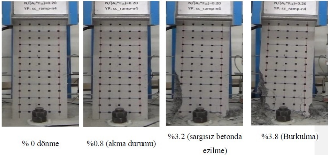
Şekil 3.11 S352008 için deney sırasında gözlemlenen hasar durumları
