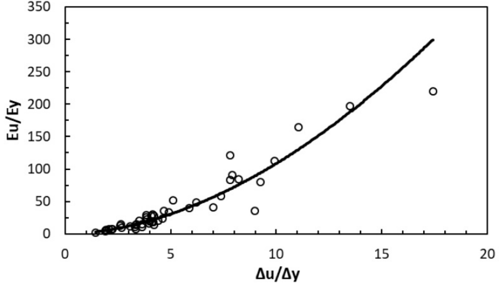
Şekil 6.3 Göçme durumuna ait normalize edilmiş kümülatif sönümleme enerjisi ile düktilite ilişkisi
