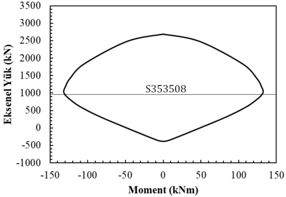
Şekil 3.19 S353508 için kapasite eğrisi
