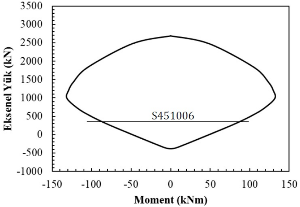
Şekil 3.28 S451006 için kapasite eğrisi
