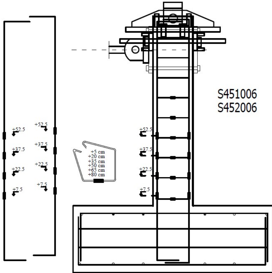
Şekil 2.13 Şekildeğiştirme ölçerlerin konumları
