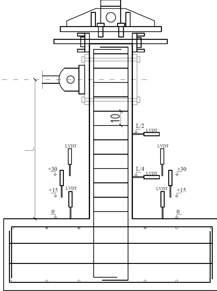
řekil 2.14 Kolon boyunca yerleřtirilen LVDT'lerin konumu
