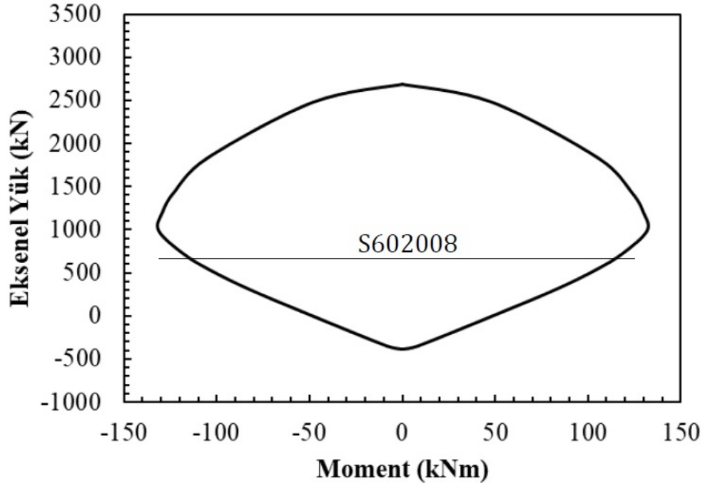
Şekil 3.16 S602008 için kapasite eğrisi
