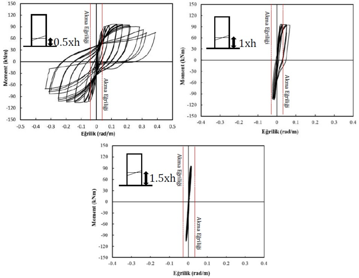
Şekil 4.39 S451006 için üç farklı seviyede moment-eğrilik diyagramı
