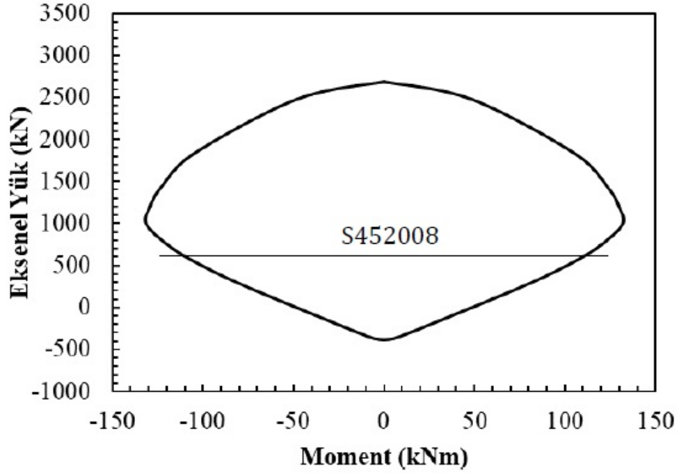
Şekil 3.13 S452008 için kapasite eğrisi
