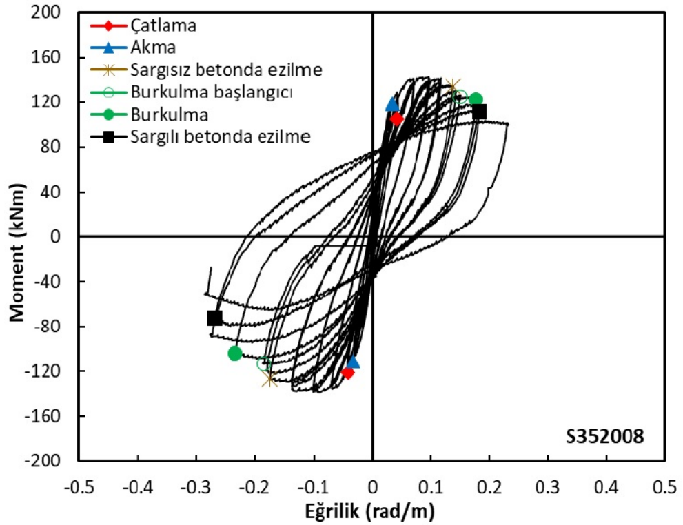
Şekil 3.49 S352008 için deneysel maksimum moment-eğrilik ilişkisi
