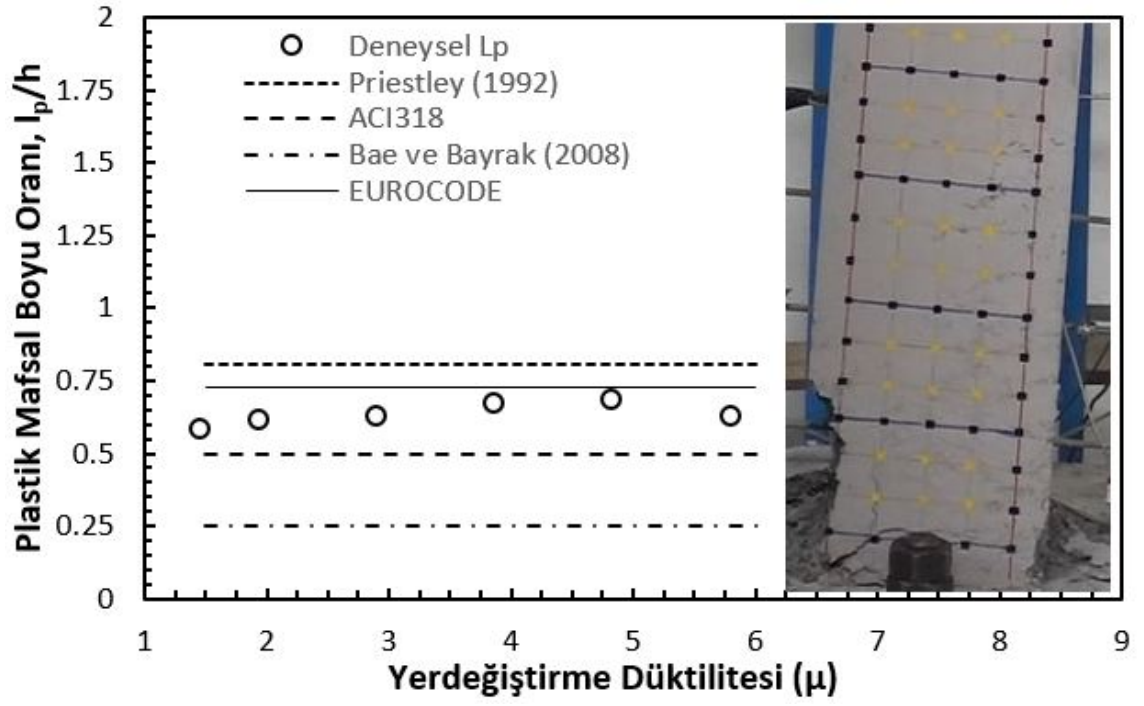
Şekil 4.41 S451006 kolonu için plastik mafsalları
