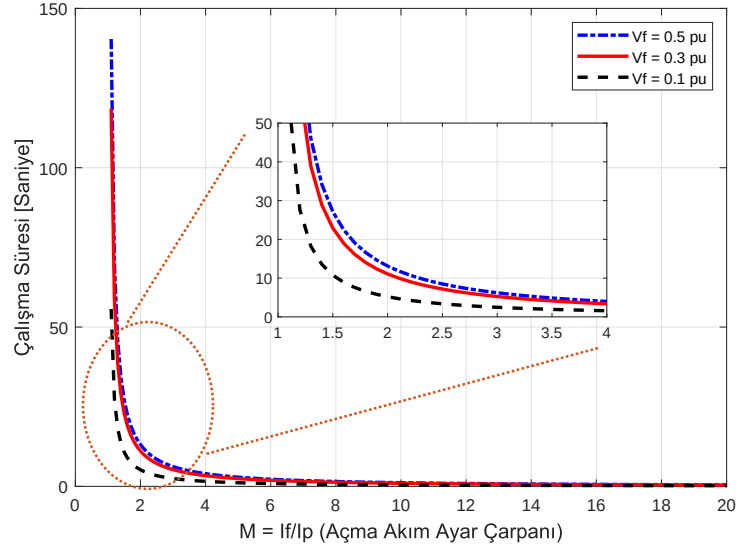
Şekil 2.7 Gerilim değişiminin denklem (2.6)'da A = 80 , B = 2 , k = 1,71 ve TDS = 1 olduğu düşünümlere oluşturulan standart dışı karakteristik üzerindeki etkisi
