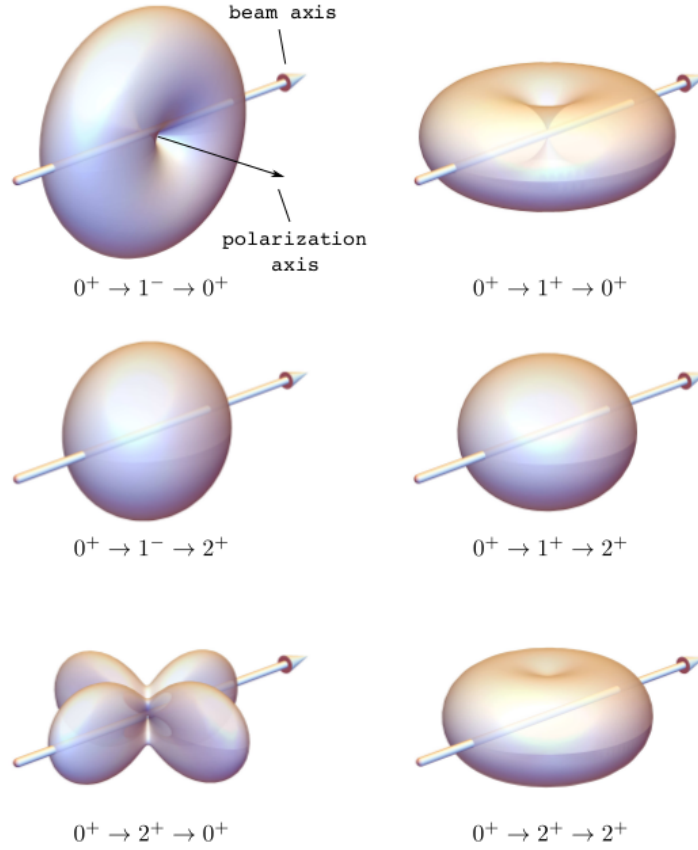
Şekil 2.5 Linear polarize foton ışınları kullanarak ^{156}\text{Gd} gibi çift-çift çekirdekler için NRF ölçümleri ile ilgili spin dizileri için açısıl dağılımlar[54]
