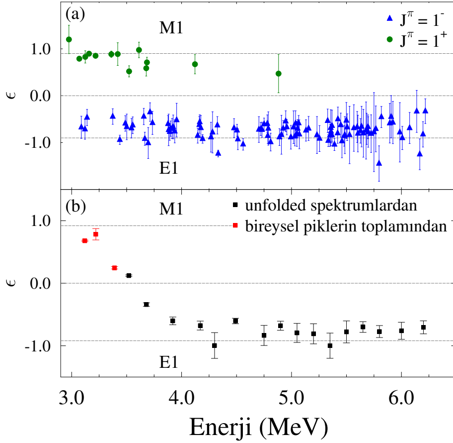
Şekil 5.1 Gözlemlenen bireysel durumlar için asimetriler (a) ve düzeltilmiş (unfolded) spektrumları (b) kullanarak her bir ışın enerjisi için ortalama asimetri dağılımı (Her iki durumda da sadece temel seviyeye geçişler ele alınmıştır. Noktalı yatay çizgiler, sırasıyla E1 ve M1 geçişleri için beklenen değerleri işaret eder.)
