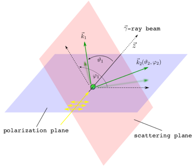
Şekil 2.4 İki fotonun \gamma - \gamma korelasyonu için koordinat sisteminin gösterimi, nükleer seviyenin bozunumunda yayılan foton ışınları (yeşil oklar), lineer olarak polarize edilmiş bir foton ışınıyla (sarı ok) uyarılan nükleer seviyenin bozunumunda yayılan foton ışınları (yeşil oklar) (Metinde daha ayrıntılı bir açıklama verilmiştir[54].)
