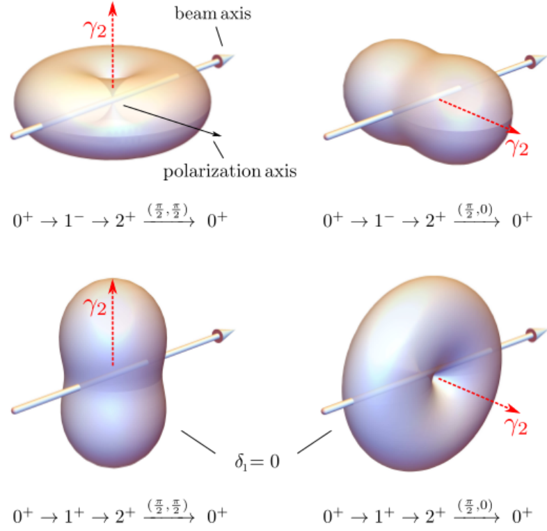
Şekil 2.7 ( 0^+ \xrightarrow{1^-} 2^+ \xrightarrow{\gamma_2} 0^+ ) ve ( 0^+ \xrightarrow{1^+} 2^+ \xrightarrow{\gamma_2} 0^+ ) örnekleri için ardışık iki foton \gamma_1 ve \gamma_2 arasındaki açılal ilişki ( \gamma_1 'in yönlü açılal ilişkisi, \gamma_2 'nin gözlem yönüne ( \vartheta, \varphi ) bağılı olarak değişir (kırmızı kesikli ok).)
