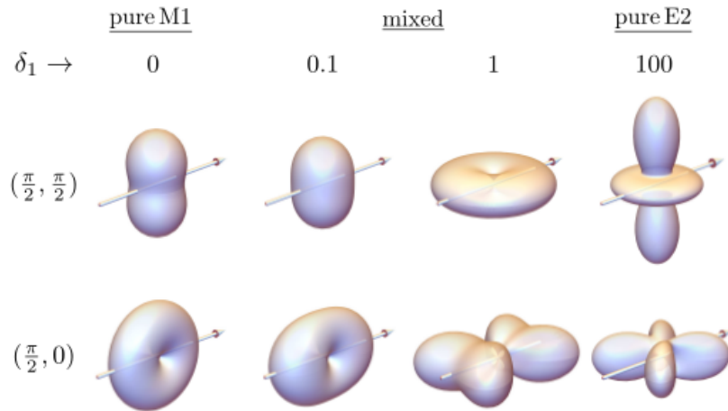
Şekil 2.8 ( 0^+ \xrightarrow{1^-} 2^+ \xrightarrow{(\vartheta, \varphi)} 0^+ ) spin düzeninde karışım oranı \delta_1 'in fonksiyonu olarak \gamma_2 'nin gözlem yönüne göre \gamma_1 'in açılal yönelim ilişkisi (Sadece M1 geçişleri (Pure M1), sadece E1 geçişleri (Pure E1) ve karışım oranları (mixed) gösterilmiştir.)
