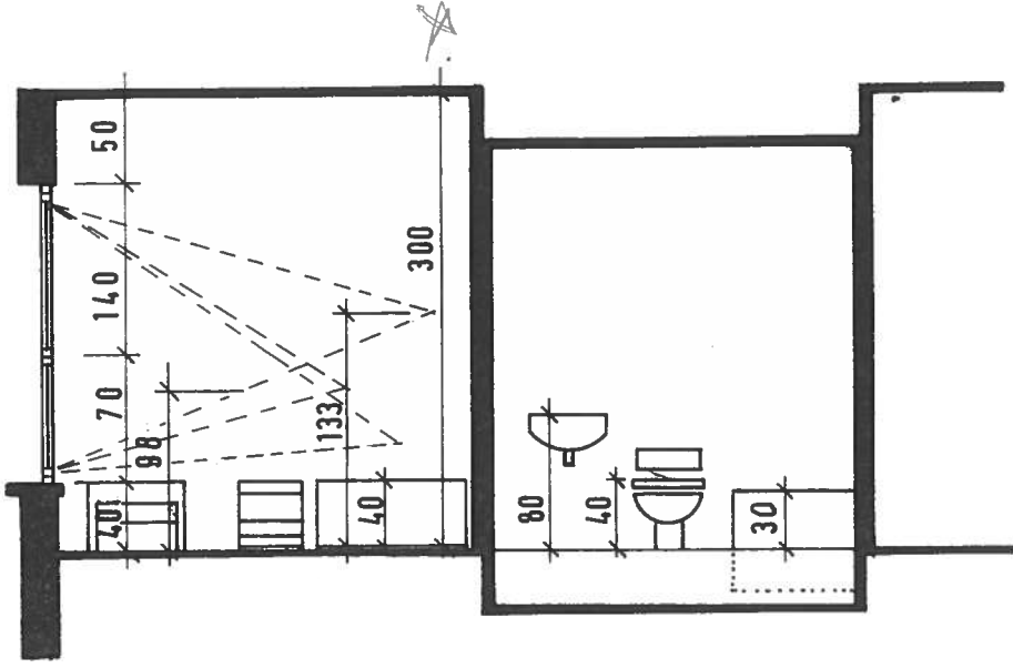
ŞEKİL 38. Yatak Odası Kesiti Ö:1/50
