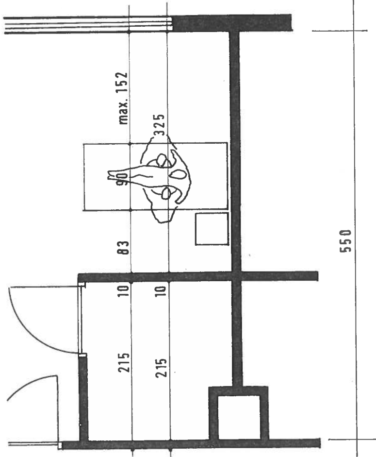
Şekil 39. Pencere Yatak Uzaklığı Ö:1/50
