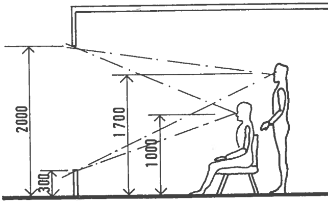
Şekil 7. Oturma Salonu Pencere Yüksekliği
