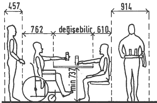
Sekil 4. Yemek Salonu Kullanım Ölçüleri
