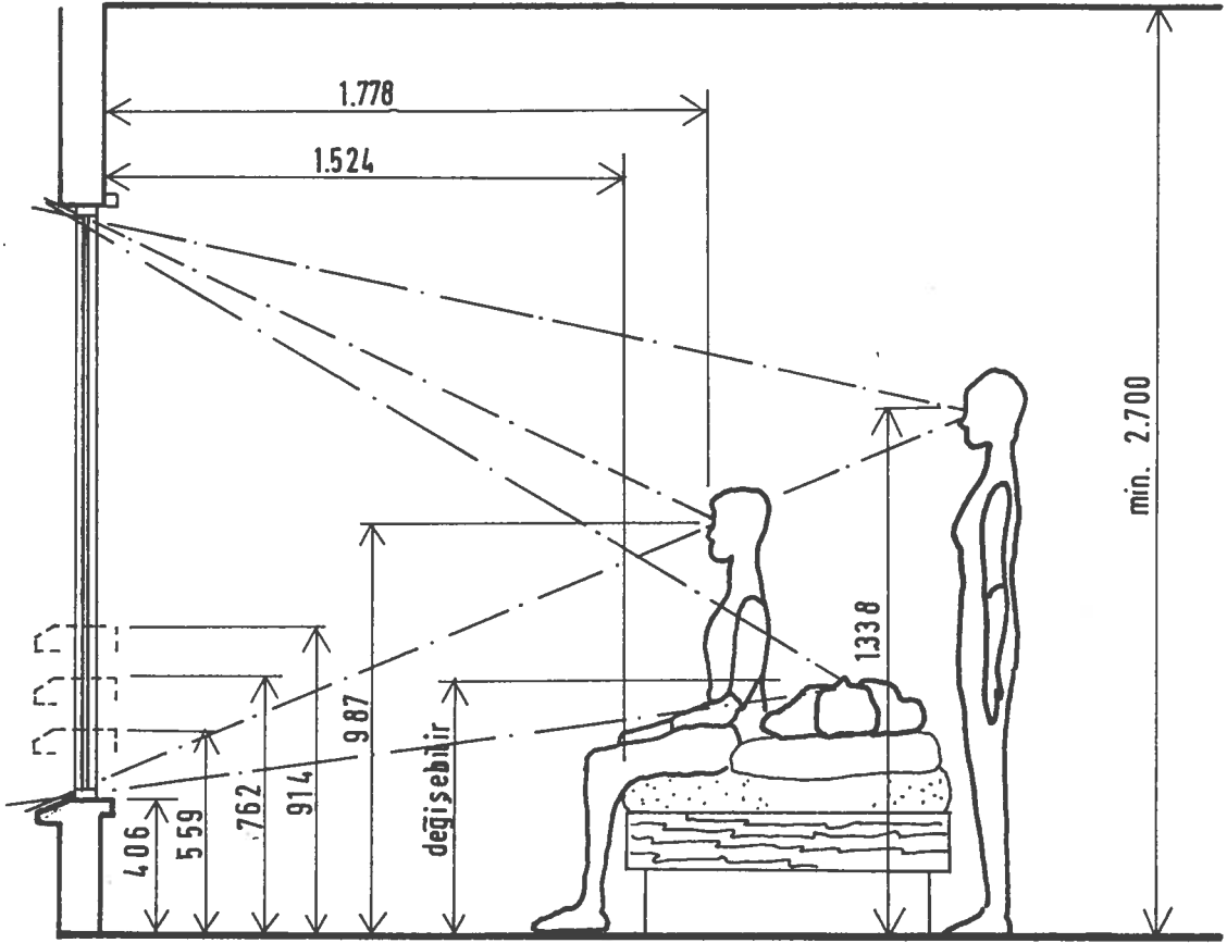
Şekil 2. Yatak Odalarında Pencere ve Kat Yüksekliği
