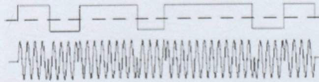
Şekil 5.21 BPSK işareti
