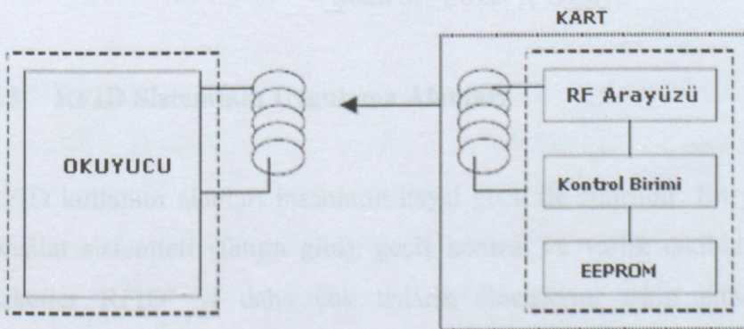
Şekil 3.6 Okunabilir yazılabilir RF etiketler
