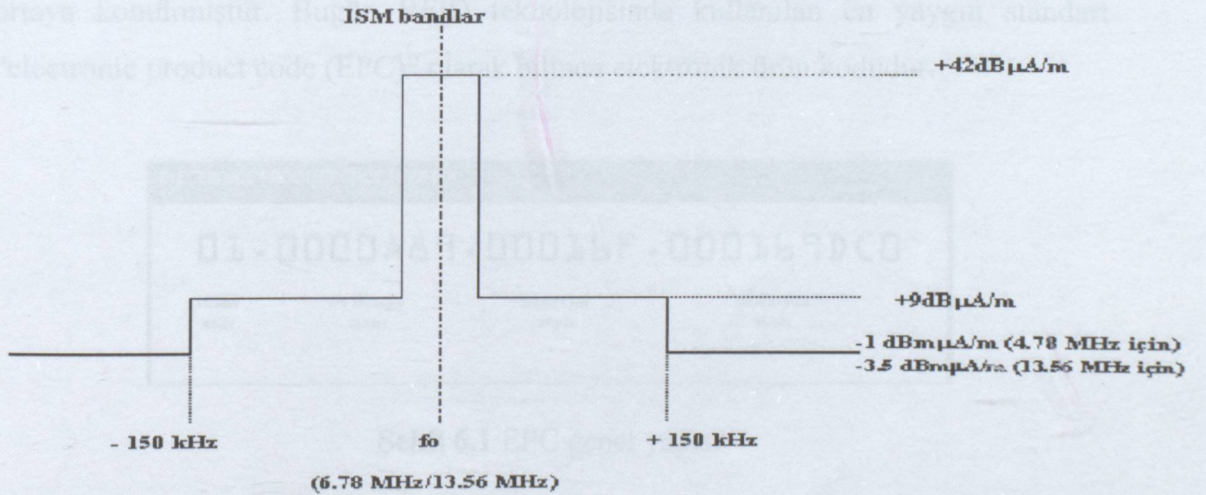
Şekil 5.24 6.78 MHz ve 13.56 MHz bandlarında 10 metrede ölçülen manyetik alan sınır değerleri
