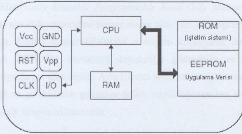
Şekil 2.10 Tipik Mikroişlemcili Kart Yapısı
