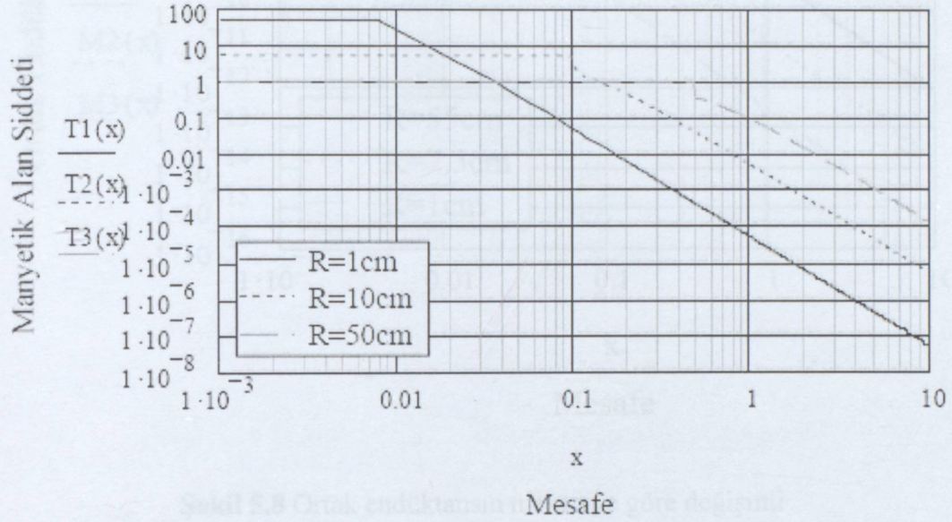
Şekil 5.6 Manyetik alan şiddetinin mesafeye göre değişimi
