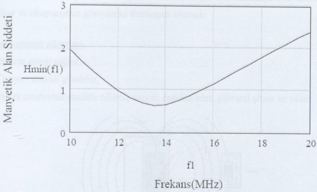
Şekil 5.10 Manyetik alan şiddetinin frekansa göre değişimi
