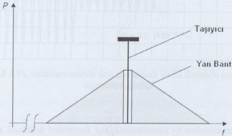
Şekil 5.13 Sinüzoidal sinyal modülasyonu (taşıyıcı ve yan bantlar)
