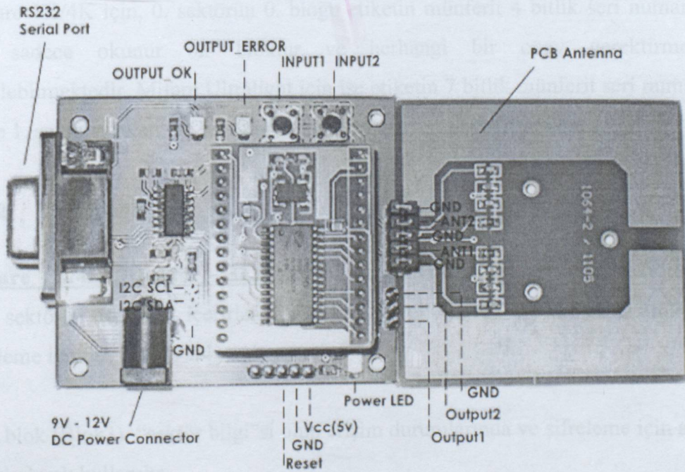
Şekil 7.1 SM 1013 Uygulama Geliştirme Kitinin Üstten Görünümü
