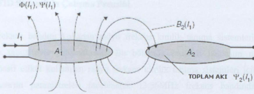
Şekil 5.5 İki bobinin oluşturduğu karşılıklı endüktans
