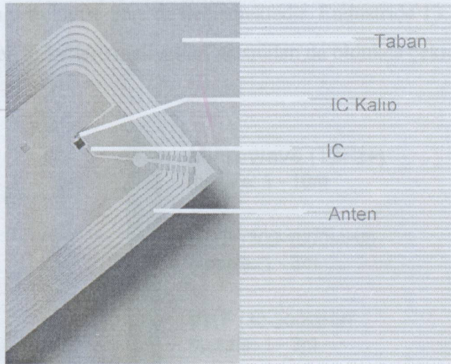
Şekil 3.3 RFID Etiket yapısı
