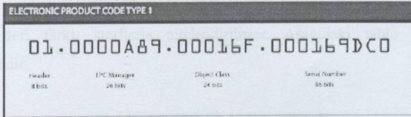
Şekil 6.1 EPC genel yapısı
