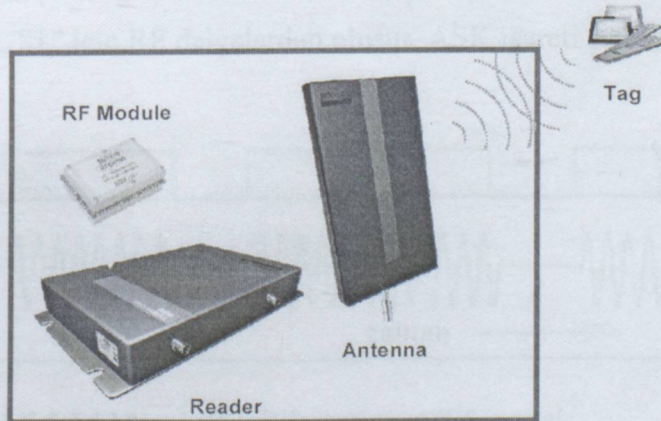
Şekil 5.12 RFID Haberleşme Yapısı
