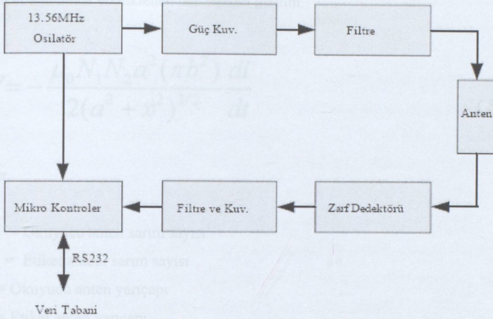
Şekil 5.2 RFID Okuyucu devre yapısı
