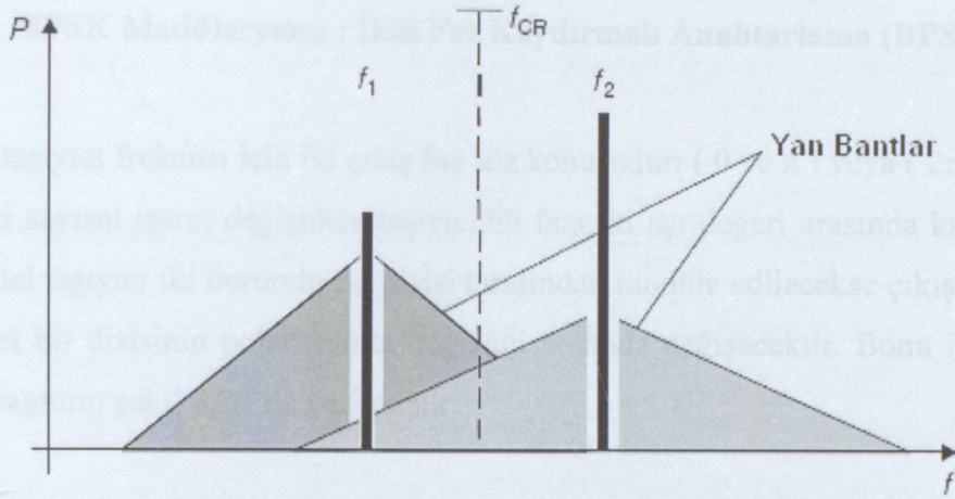
Şekil 5.18 FSK modülasyonu
