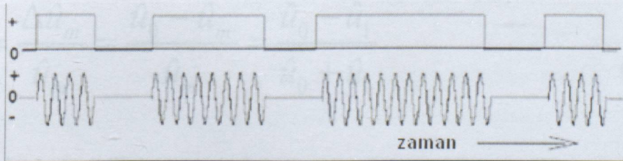
Şekil 5.14 Mesaj (Bilgi) işareti ve ASK işareti
