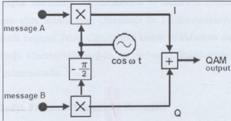
Şekil 5.22 QAM modülatörü (QPSK modülatörü)
