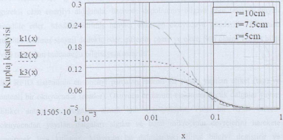
Şekil 5.9 Kuplaj katsayısının mesafeye göre değişimi
