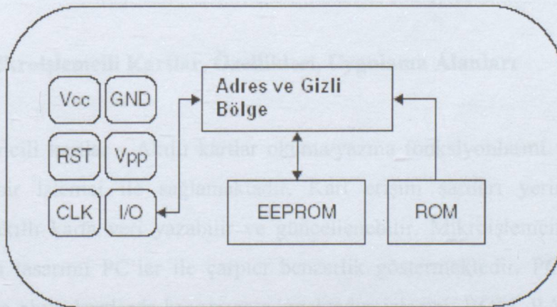
Şekil 2.9 Tipik Bellekli Kart Yapısı
