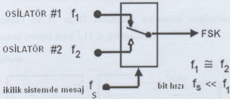
Şekil 5.17 FSK üretimi
