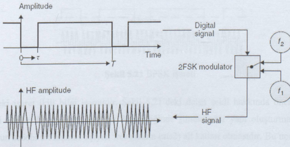
Şekil 5.19 2 FSK modülasyonunun üretimi
