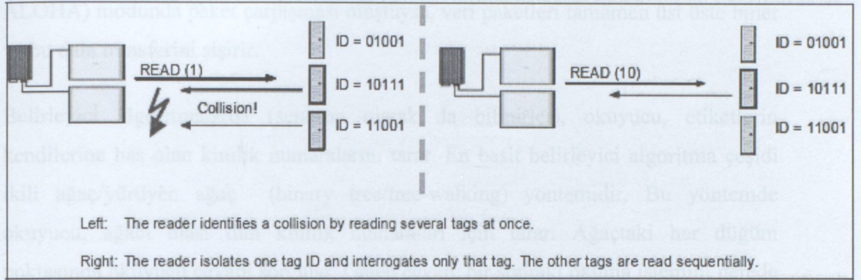
Şekil 6.2 RFID Okuyucu Çarpışması Protokolü
