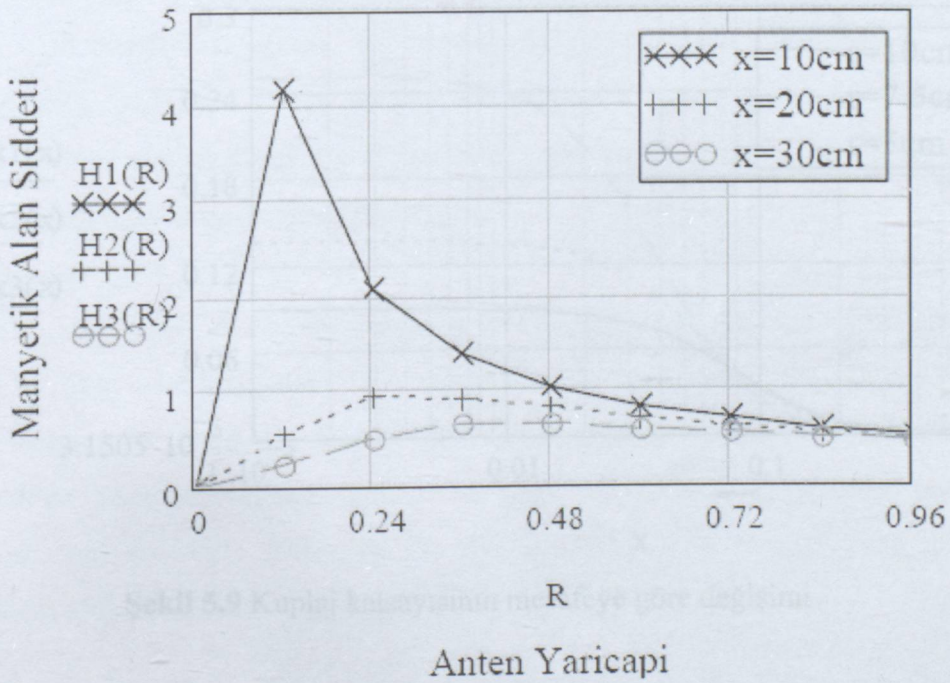
Şekil 5.7 Manyetik alan şiddetinin anten yarıçapına göre değişimi
