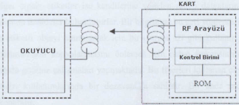
Şekil 3.5 Yalnız okunabilir RF etiket
