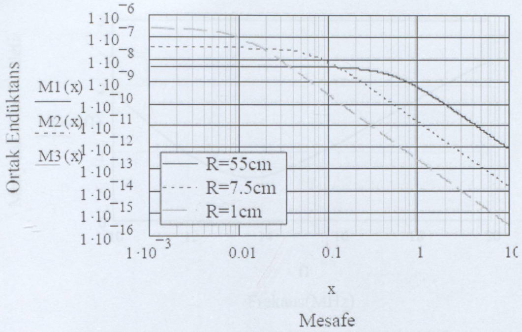
Şekil 5.8 Ortak endüktansın mesafeye göre değişimi
