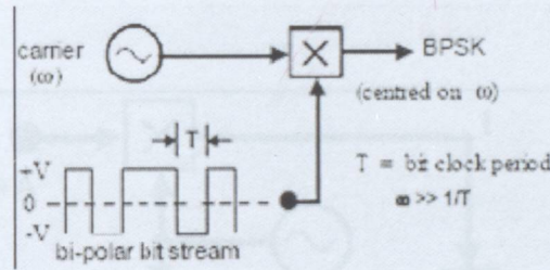
Şekil 5.20 BPSK işaretinin üretilmesi
