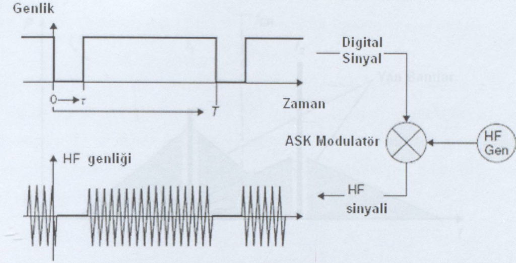
Şekil 5.16 ASK modülasyonunun üretilmesi
