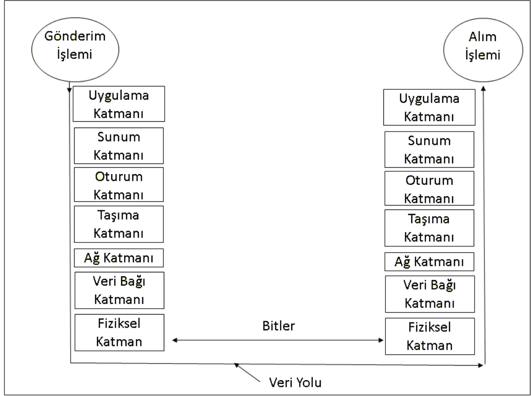
Şekil 6.3 OSI Katmanları
