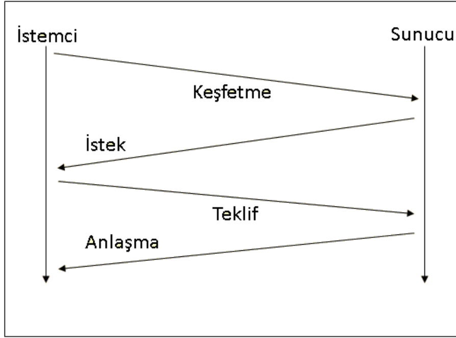
Şekil 6.4 DHCP Protokol Akışı
