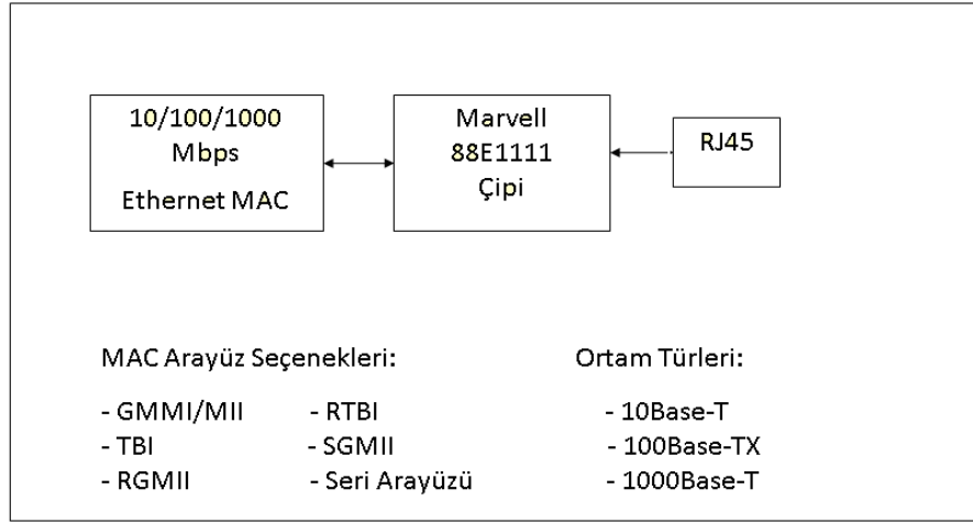
Şekil 6.2 88E1111 Çipinin Uygulamalardaki Kullanımı[39]
