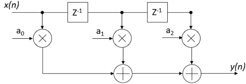
Şekil 4.2 FIR Filtre
