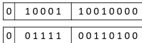
Şekil 2.3 Kayan-Nokta Toplama Örneği
