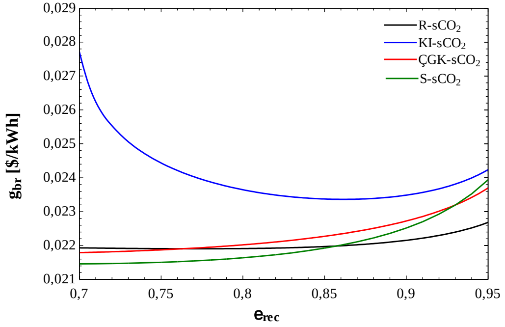
Şekil 3.35 Çevrimlerin reküperatör etkinliği-birim elektrik üretim maliyeti
