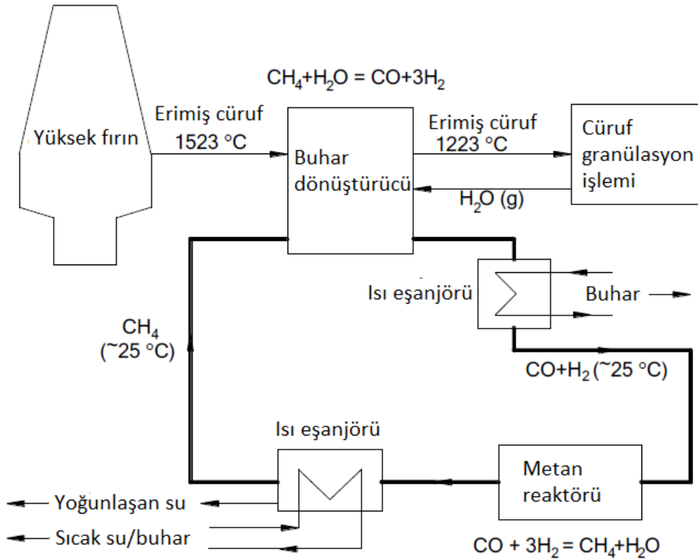
Şekil 1.19 Metanın su ile reformasyonu [24]
