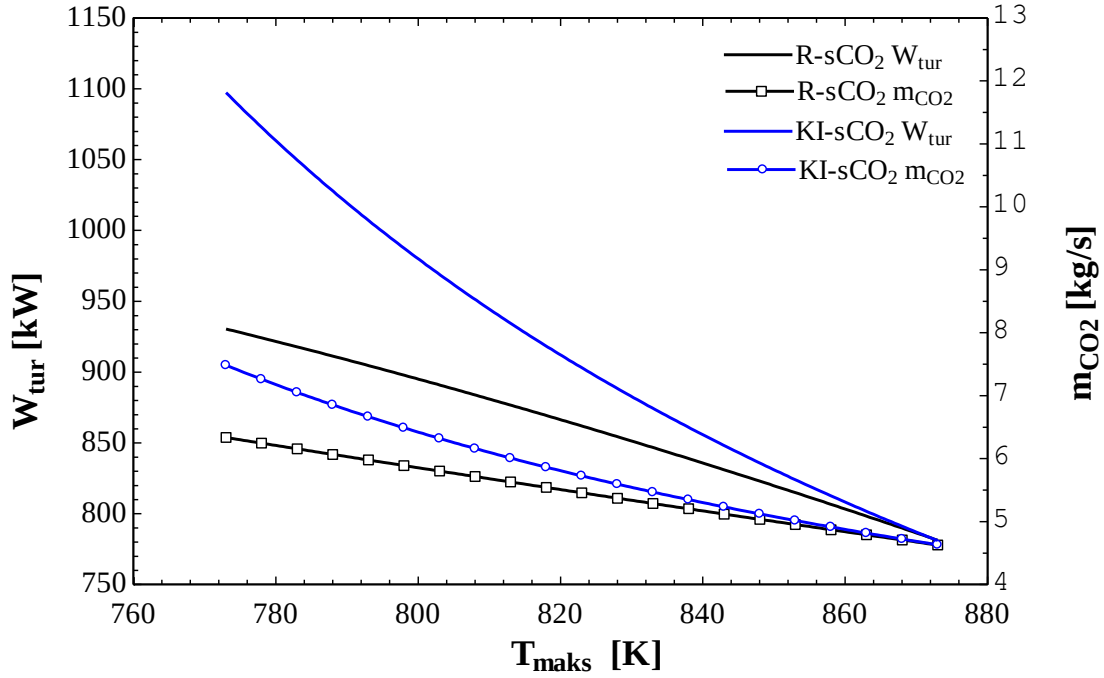
Şekil 3.18 R-sCO 2 ve KI-sCO 2 'de maksimum çalışma sıcaklığı ve türbinin ürettiği güç
