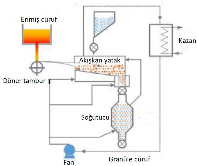
Şekil 1.9 Tek döner tamburlu yöntemin şematik gösterimi [26]
