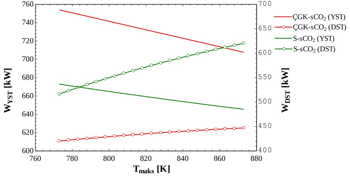
Şekil 3.19 S-sCO 2 ve ÇGK-sCO 2 'de maksimum sıcaklık ve türbinlerin ürettiği güç Maksimum çalışma sıcaklığı artışı ile birlikte tüm sCO 2 çevrimlerinde tanımlanan \eta_{1,çevrim} verim eğrileri, çevrimlerin net güç üretim eğrileri ile benzerlik göstermektedir. Şekil 3.20'de maksimum sıcaklığın \eta_{1,çevrim} etkisi gösterilmiştir.
