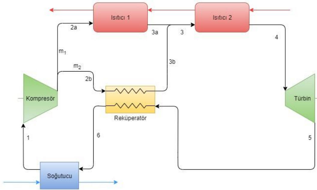
Şekil 3.3 KI- \text{sCO}_2 çevriminin şematik gösterimi
