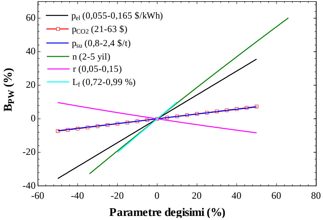
Şekil 4.2 ÇGK-sCO 2 çevriminin entegre olduğu sistemde, ekonomik giriş parametre değişimleri durumunda toplam gelirin ( B_{PW} ) duyarlılık analizi
