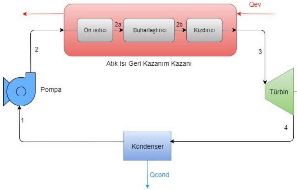
Şekil 3.10 Buhar Rankine çevriminin şematik gösterimi
