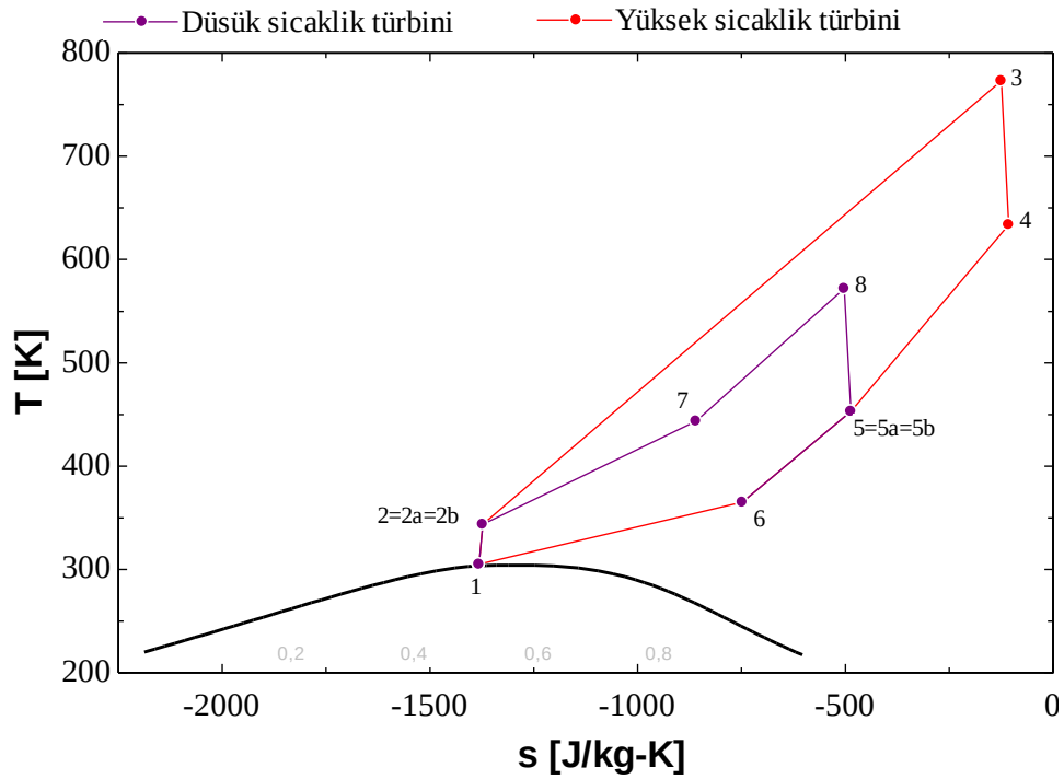
Şekil 3.6 S-sCO 2 çevriminin T-s grafiği
