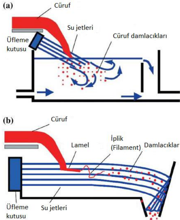
Şekil 1.4 (a) Soğuk yolluk tankı ve (b) Yüksek basınçlı su püskürtmesine sahip ıslak granülasyon işlemi şeması [14]
