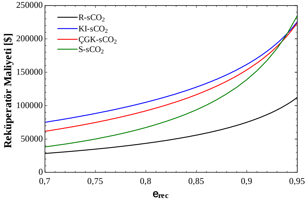
Şekil 3.36 Reküperatör etkinliğinin maliyetine etkisi
