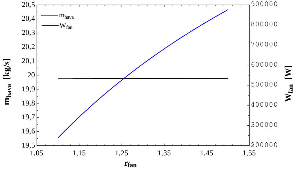
Şekil 2.6 Fan özel oranının güç tüketimine etkisi
