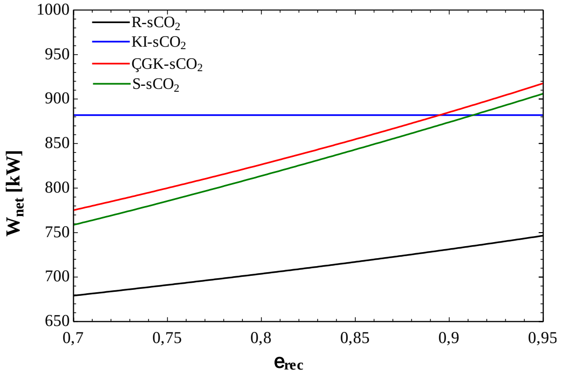
Şekil 3.24 sCO 2 çevrimlerinin net güç çıkışı-rekuperatör etkinliği
