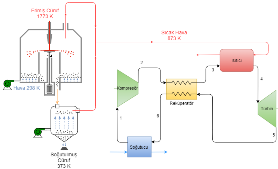
Şekil 4.1 Santrifüj granülasyon yöntemine entegre R- \text{sCO}_2 çevrimi
