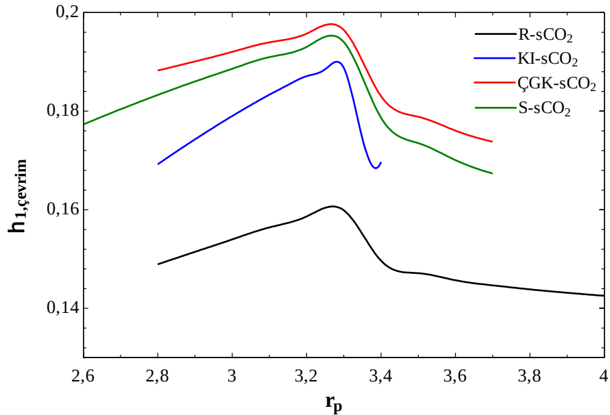
Şekil 3.15 25 MPa maksimum basınçta basınç oranının çevrimin \eta_{1,çevrim} değerine etkisi
