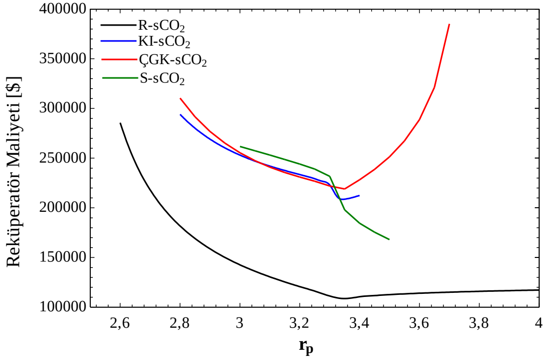
Şekil 3.30 Çevrim basınç oranının reküperatör maliyetine etkisi
