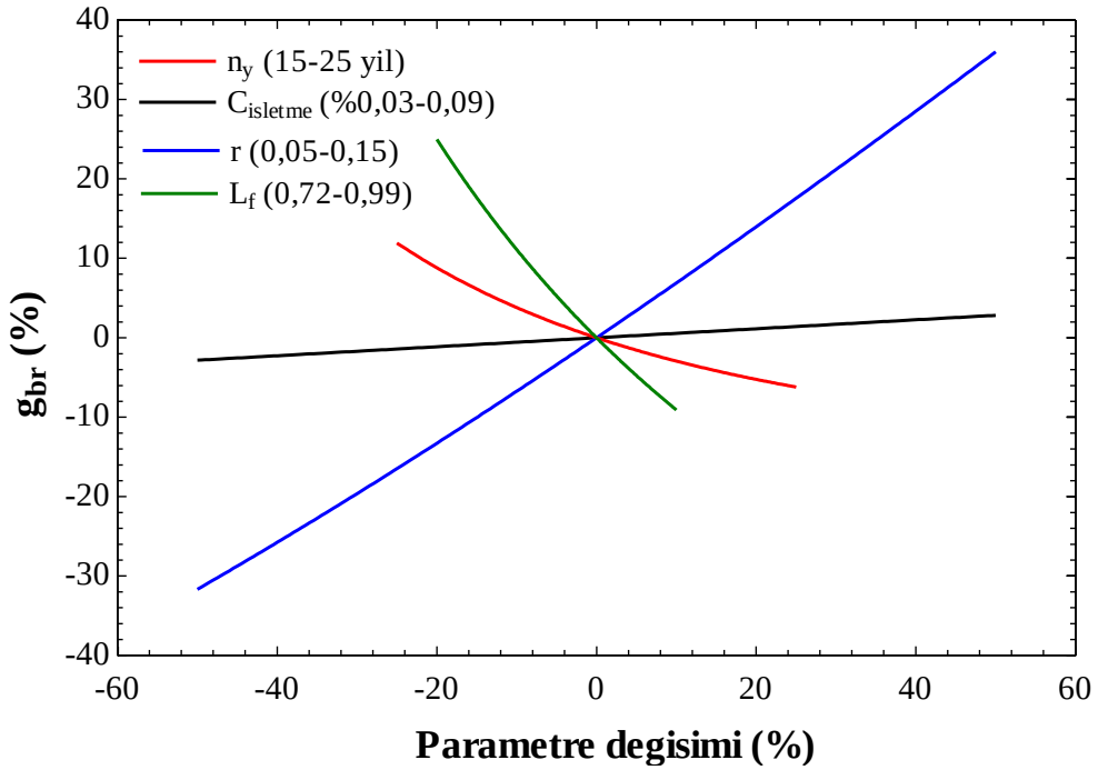
Şekil 3.41 S-sCO 2 çevriminde ekonomik giriş parametre değışimleri durumunda g_{br} 'nin duyarlılık analizi
