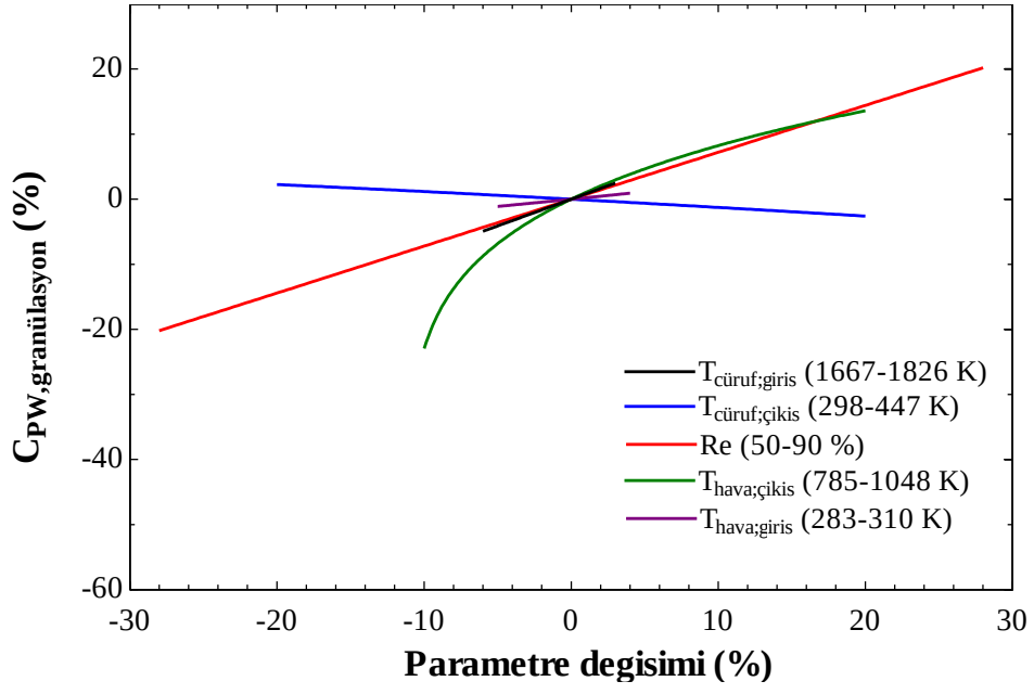
Şekil 4.4 S-sCO 2 çevriminin entegre olduęu sistemde, granülasyon giriř parametre deęişimleri durumda C_{PW,granülasyon} 'nın duyarlılık analizi
