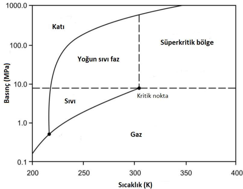
Şekil 1.22 CO 2 faz değişim grafiği [33]
