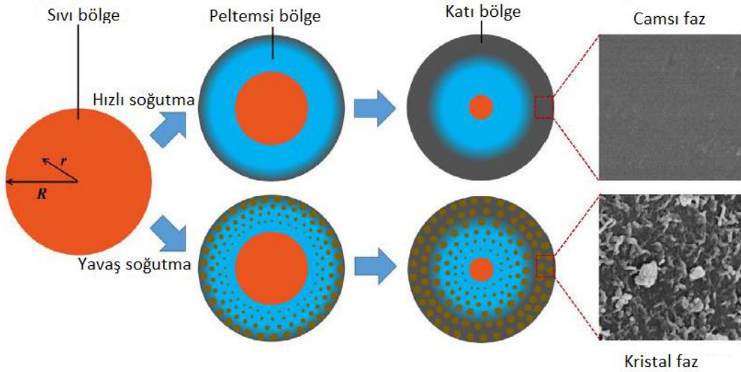
Şekil 1.7 YFC'nun soğutma hızına bağlı yapısal değişimi [23]
