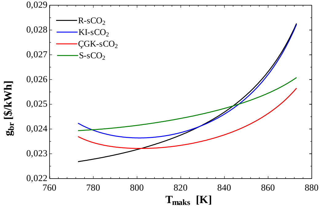
Şekil 3.31 Maksimum çalışma sıcaklığının birim elektrik üretim maliyetine etkisi sCO 2 çevrimlerindeki birim elektrik üretim maliyetinin artmasının en önemli sebebi, ısıtıcıda çalışma sıvısının daha yüksek sıcaklıklara ulaşmak zorunda olmasıdır. Bu durum ısıtıcı maliyetlerini etkilemektedir. Şekil 3.32’de maksimum sıcaklıkla değişen ısıtıcı maliyetleri gösterilmiştir.
