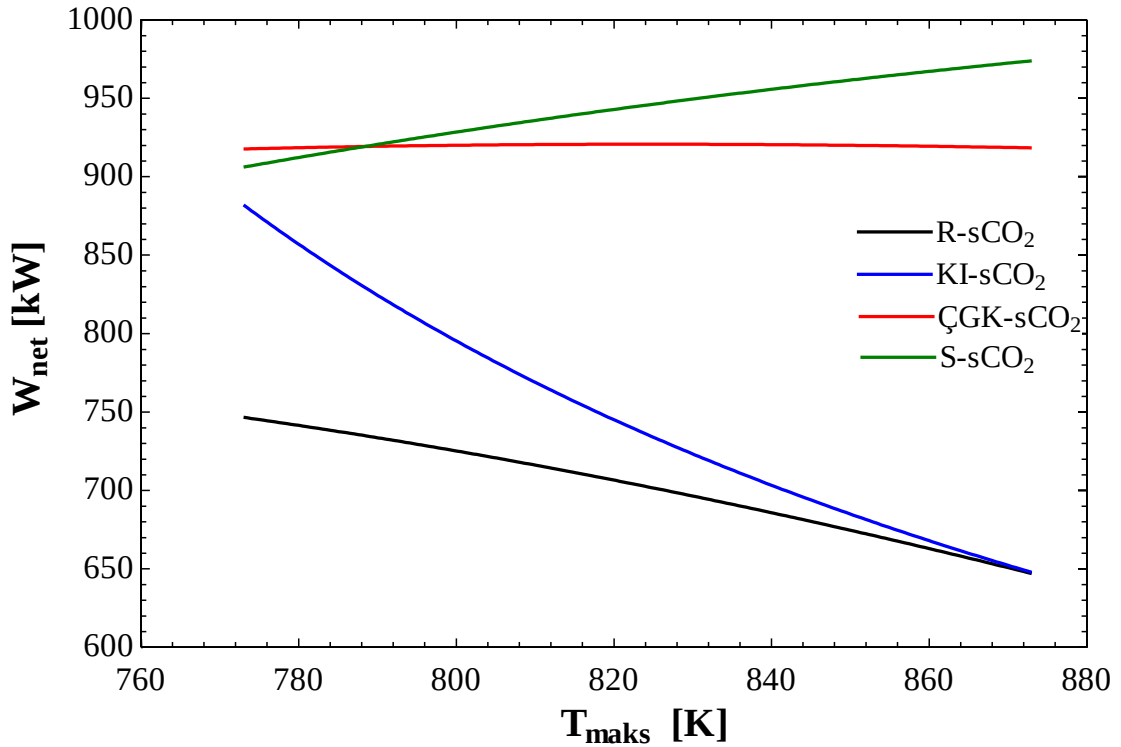
Şekil 3.17 Maksimum çalışma sıcaklığı-net güç üretimi
