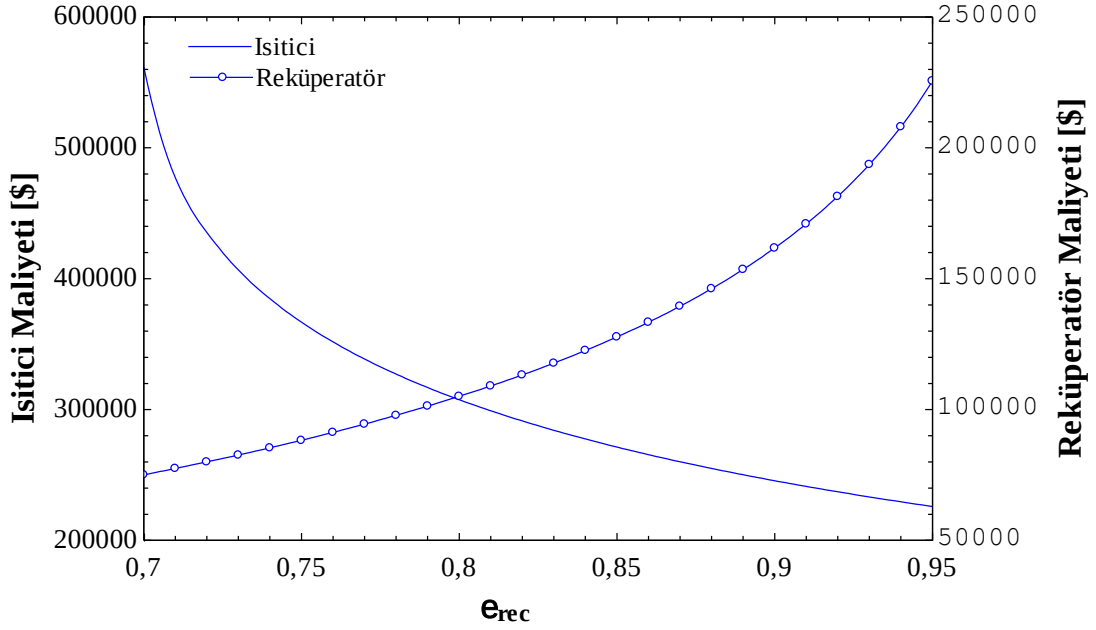
Şekil 3.37 KI-sCO 2 çevriminde reküperatör etkinliğinin ısıtıcı ve reküperatör maliyetine etkisi
