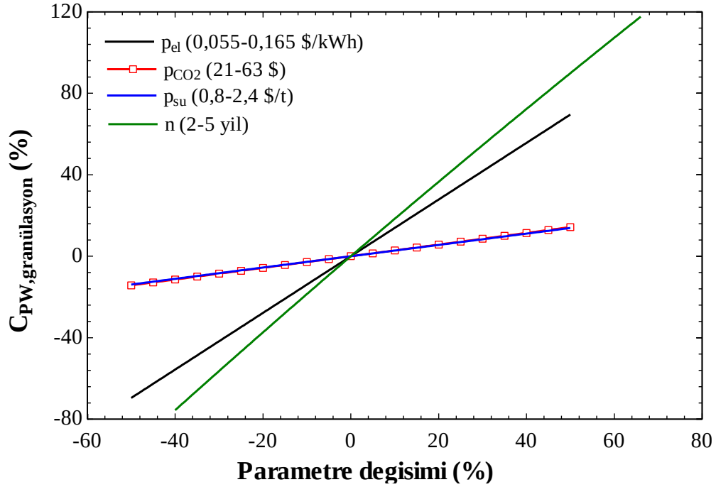
Şekil 4. 3 ÇGK-sCO 2 çevriminin entegre olduğu sistemde, ekonomik giriş parametre değişimleri durumunda C_{PW,granülasyon} 'nin duyarlılık analizi
