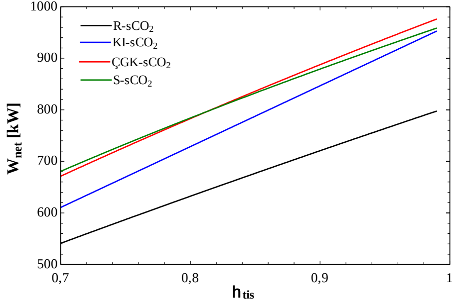
Şekil 3.22 Türbin izantropik veriminin net güç çıkışına etkisi
