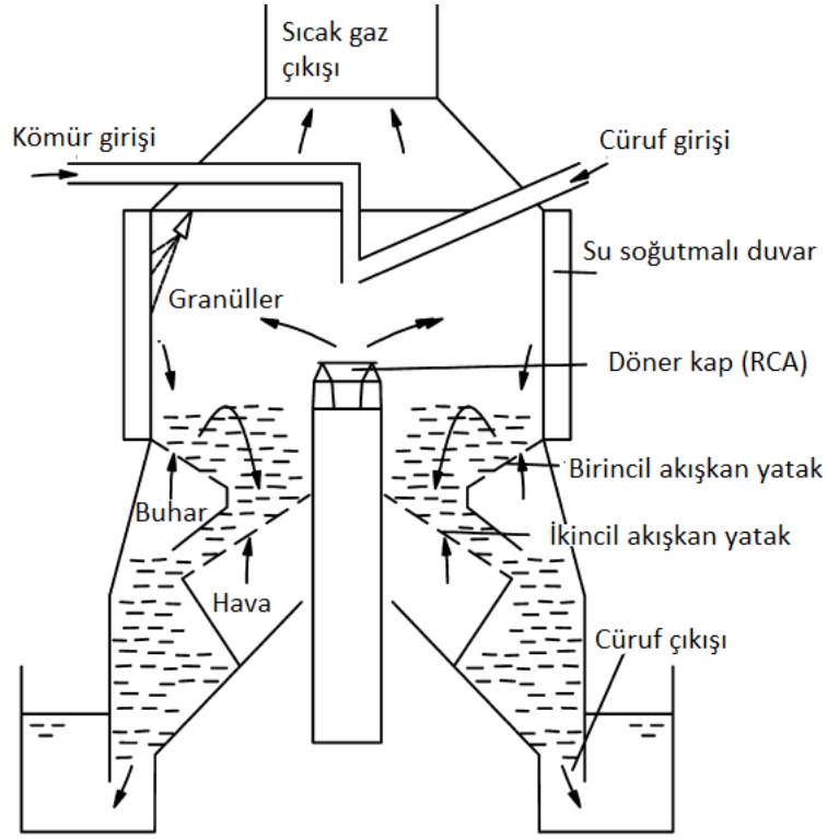
Şekil 1.21 Kömür gazı üretiminde YFC'nun kullanımı [7]
