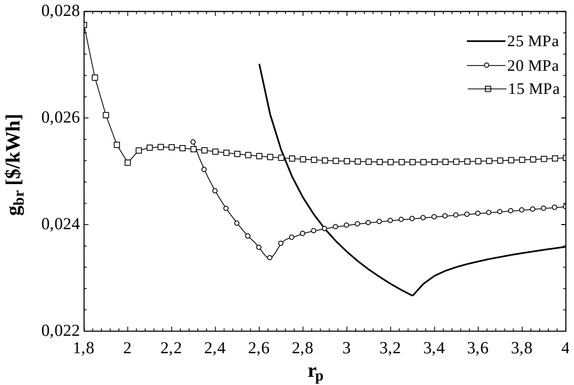
Şekil 3.28 R-sCO 2 'de maksimum basıncın ve basınç oranının, birim elektrik üretim maliyetine etkisi
