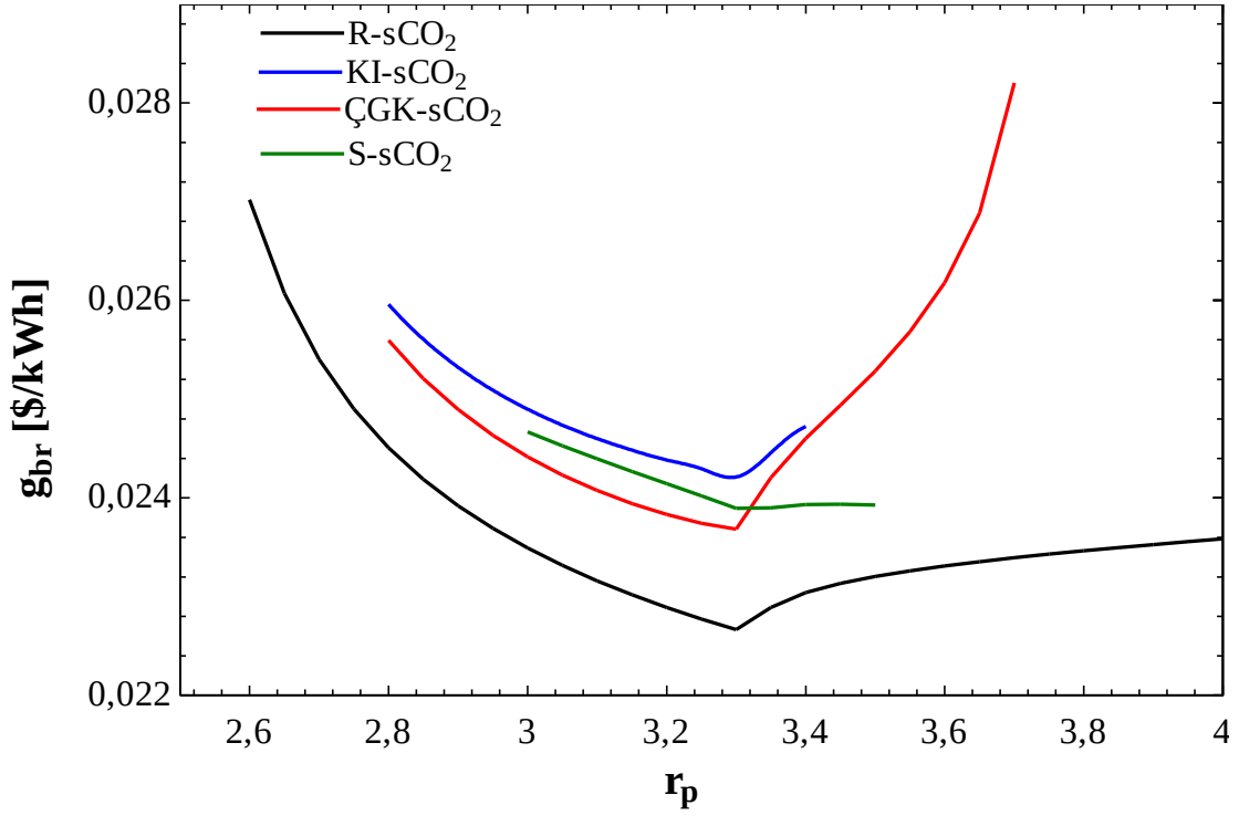
Şekil 3.29 Çevrim basınç oranının birim elektrik üretim maliyetine etkisi
