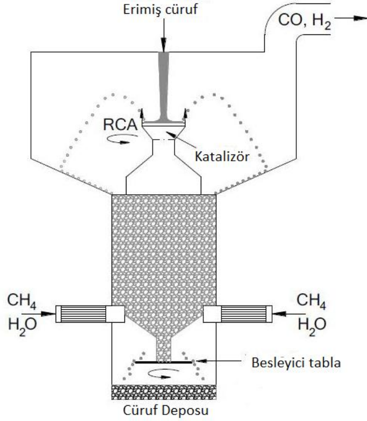
Şekil 1.20 Döner disk granülasyonu ve hidrojen üretimi [27]
