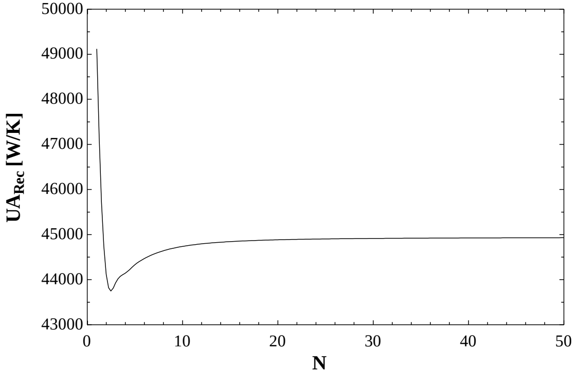
Şekil 3.12 Reküperatör iletkenliği-N grafiği
