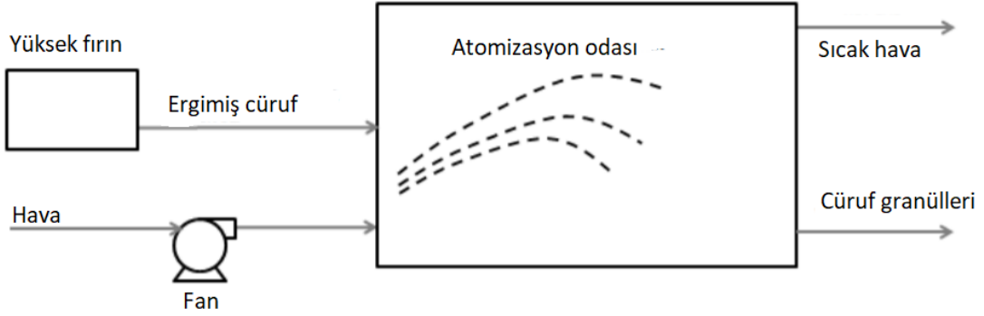
Şekil 1.11 Ecomaister ve Hatch hava püskürtmeli granülasyon yöntemi [11]
