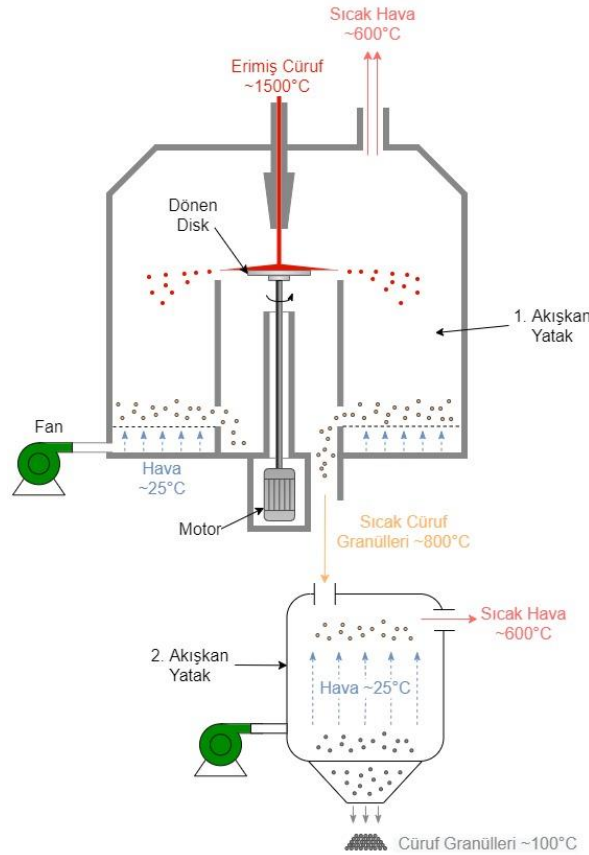
Şekil 2.1 Santrifüj kuru granülasyon sistemi şematiği
