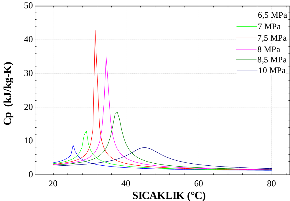
Şekil 1.23 CO 2 'in özgül ısı kapasitesinin sıcaklık ve basınca bağlı değişimi
