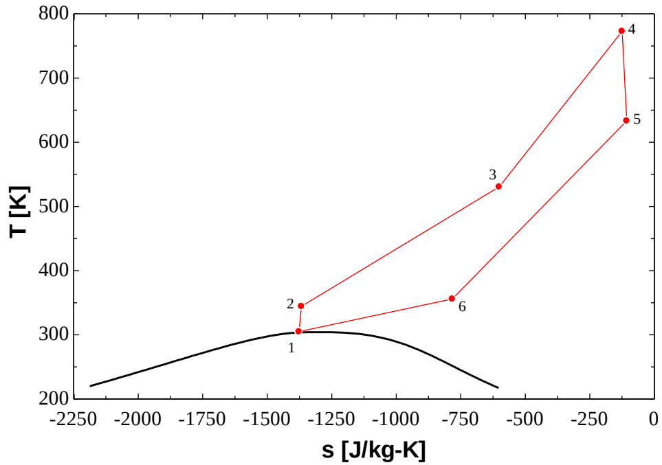
Şekil 3.2 R-sCO 2 çevriminin T-s grafiği
