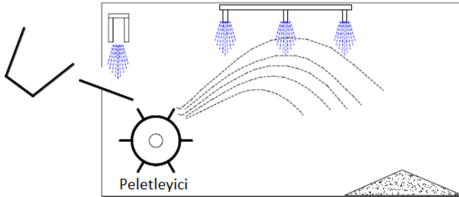
Şekil 1.5 Cüruf peletleme işleminin şematik gösterimi [11]
