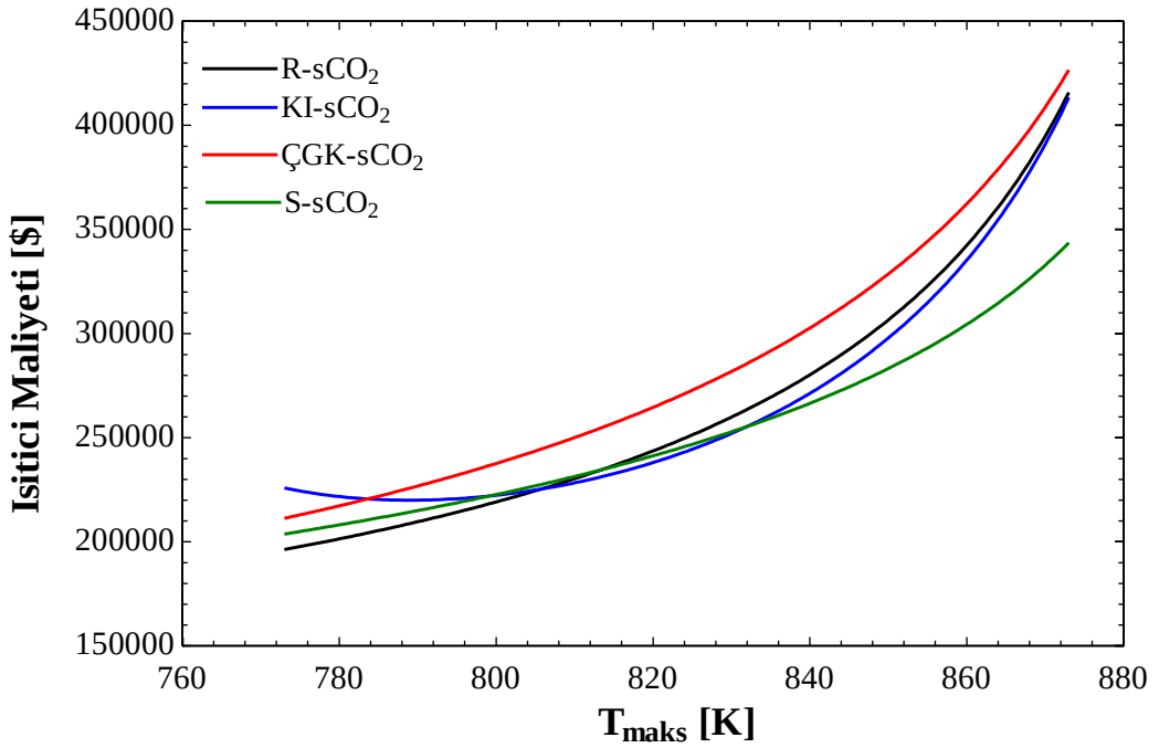
Şekil 3.32 Maksimum çalışma sıcaklığının ısıtıcı maliyetine etkisi
