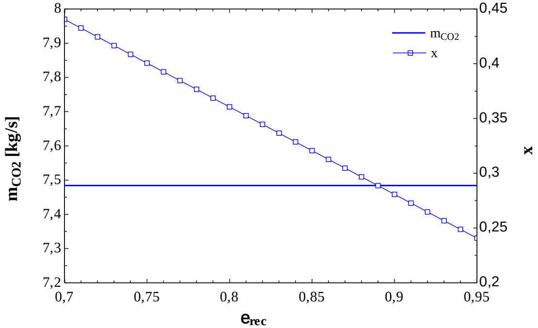
Şekil 3.25 KI-sCO 2 çevriminde rekuperatör etkinliğinin çalışma sıvısı üzerine etkisi (x:ayrışma oranı)
