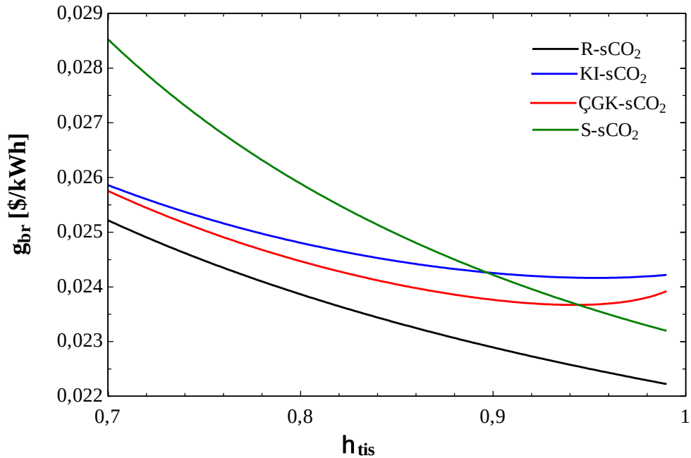
Şekil 3.33 Türbin izantropik veriminin birim elektrik üretim maliyetine etkisi
