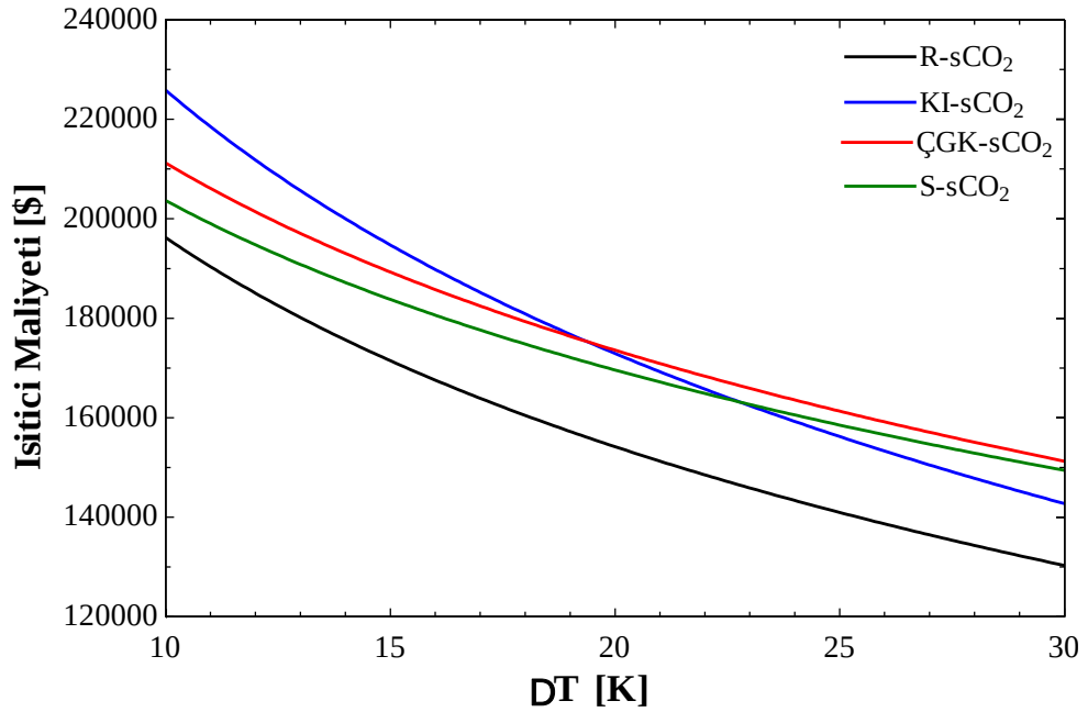
Şekil 3.39 Çevrimlerin \Delta T -ısıtıcı maliyeti
