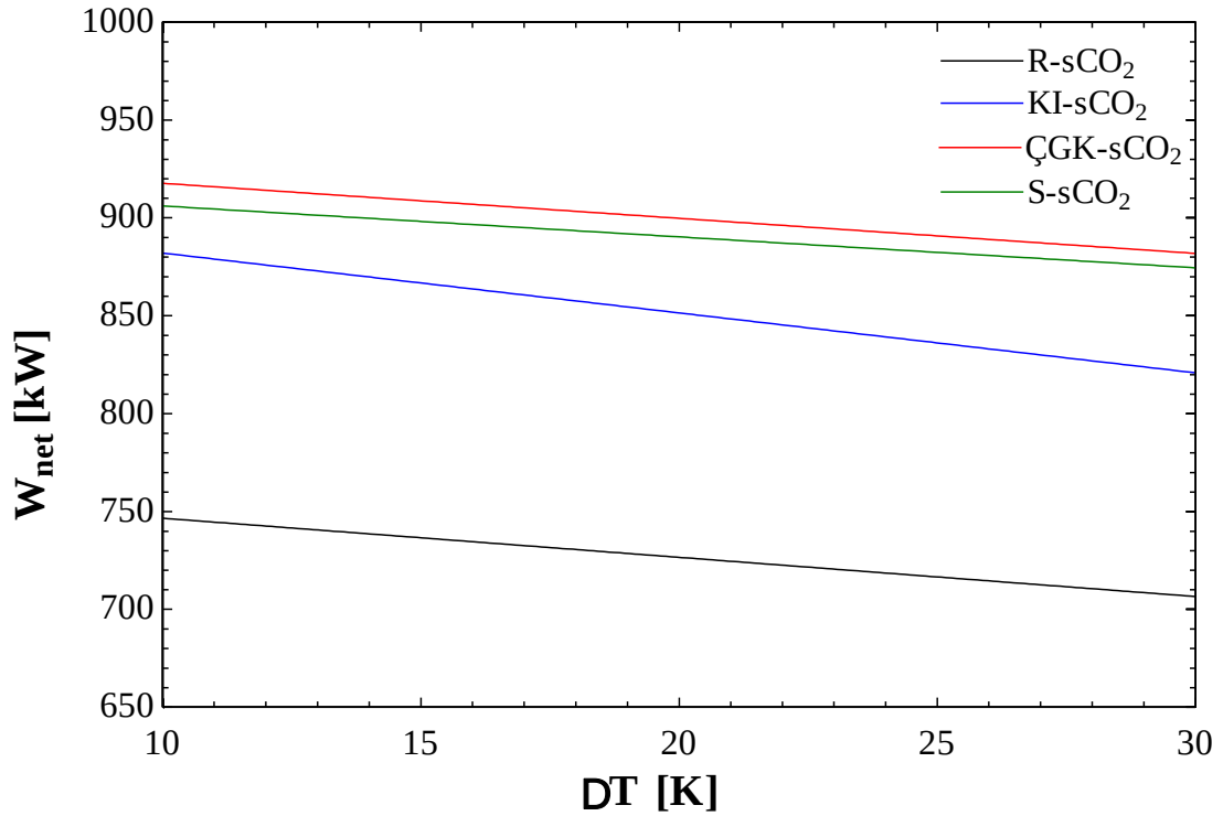
Şekil 3.26 sCO 2 çevrimlerin net güç çıkışı- \Delta T
