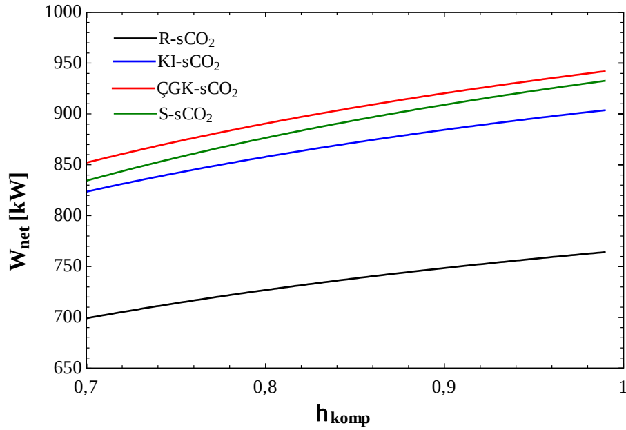
Şekil 3.23 Kompresör izantropik veriminin net güç çıkışına etkisi
