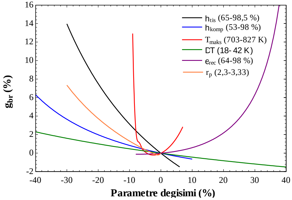
Şekil 3.40 S-sCO 2 çevriminde termodinamik giriş parametre değışimleri durumunda g_{br} 'nin duyarlılık analizi
