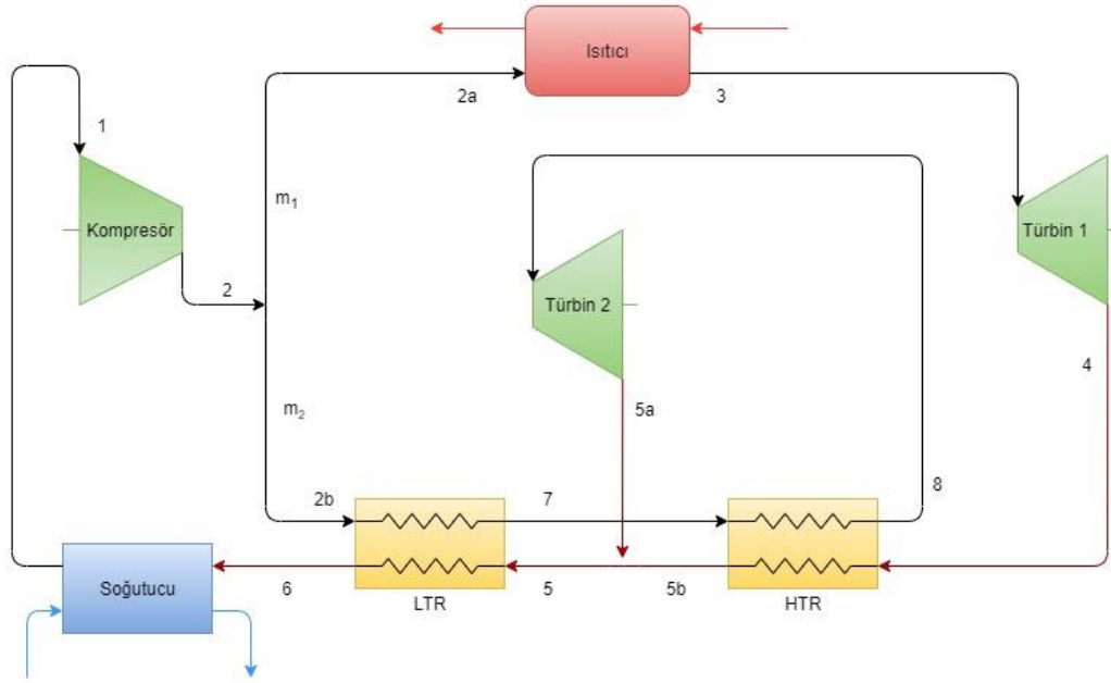
Şekil 3.5 S-sCO 2 çevriminin şematik gösterimi
