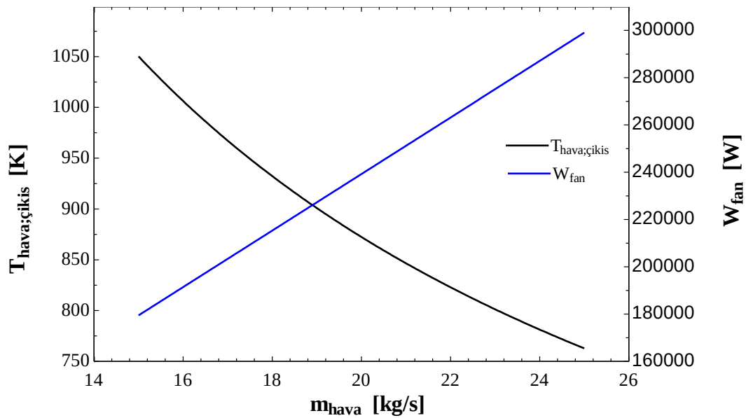
Şekil 2.4 Havanın kütlesel debi değişiminin, çıkış sıcaklığına ve fanın harcadığı güce etkisi
