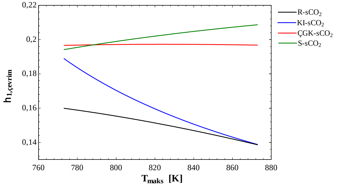
Şekil 3.20 sCO 2 çevrimlerinin \eta_{1,çevrim} -maksimum sıcaklık
