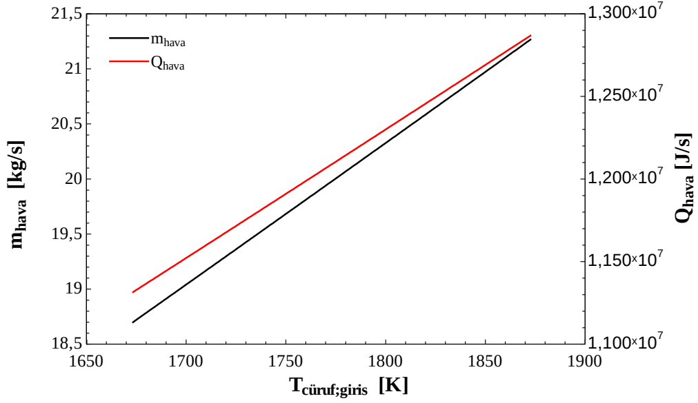
Şekil 2.2 YFC giriş sıcaklığının, havanın kütleli debisine ve kazandığı enerji miktarına etkisi
