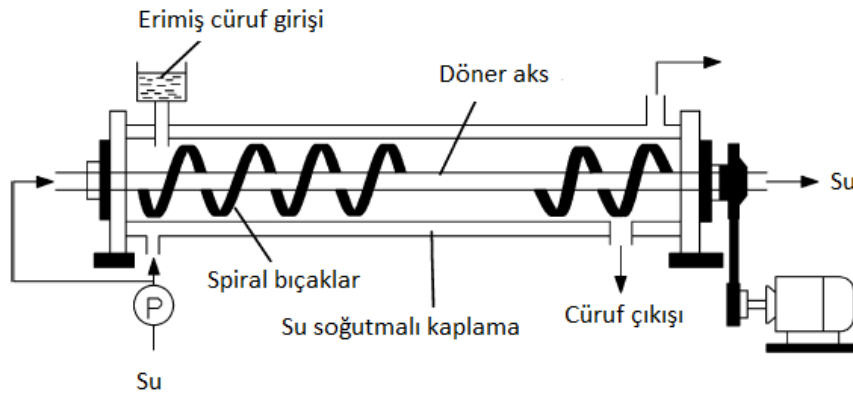
Şekil 1.13 Sumitomo Metal tarafından geliştirilen mekanik karıştırma işlemi [7]
