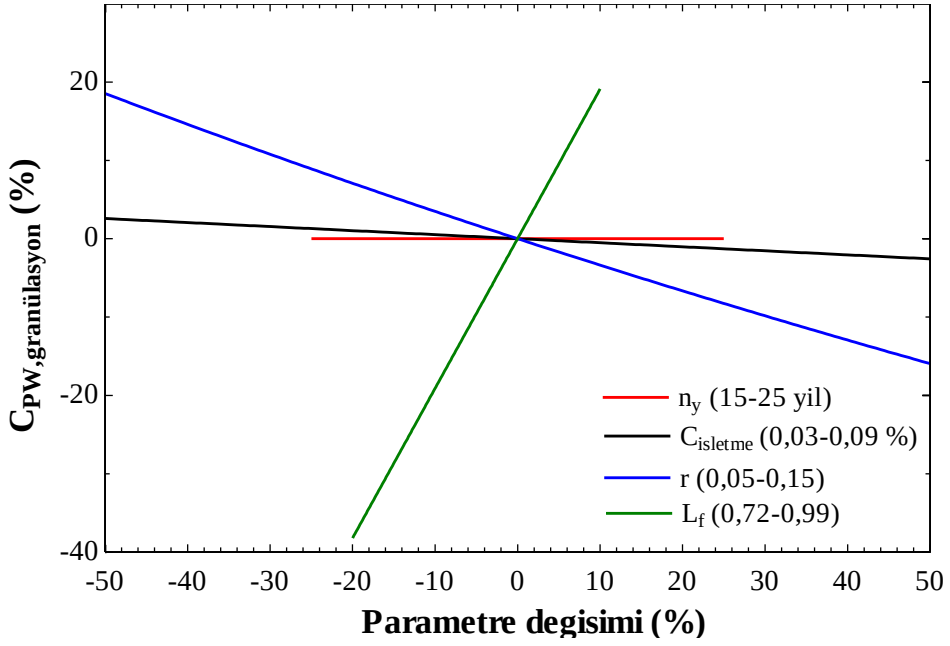
Şekil 4.5 S-sCO 2 çevriminin entegre olduęu sistemde, ekonomik giriř parametre deęişimleri durumda C_{PW,granülasyon} 'nın duyarlılık analizi
