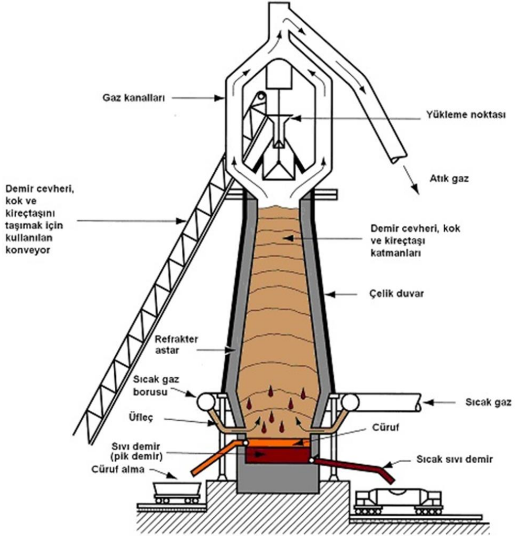
Şekil 1.1 Yüksek fırın řeması [5]
