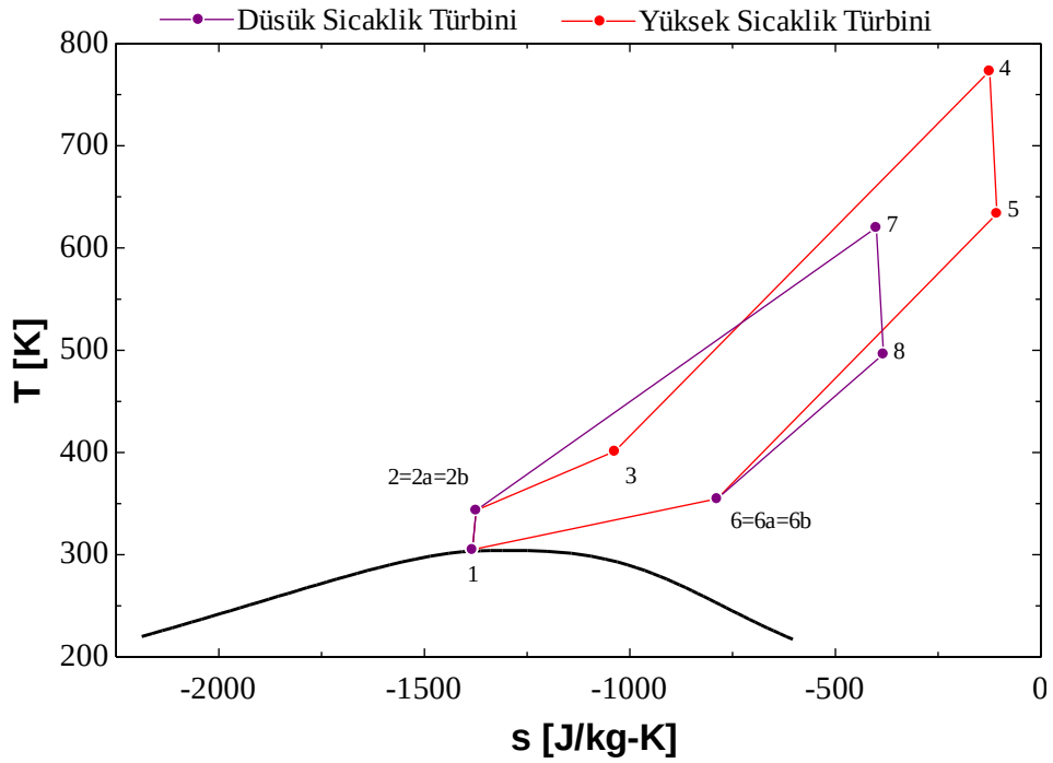
Şekil 3.8 ÇGK-sCO 2 çevriminin T-s grafiği
