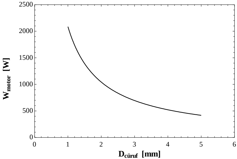
Şekil 2.5 Cüruf granül boyutunun motorun harcadığı güce etkisi
