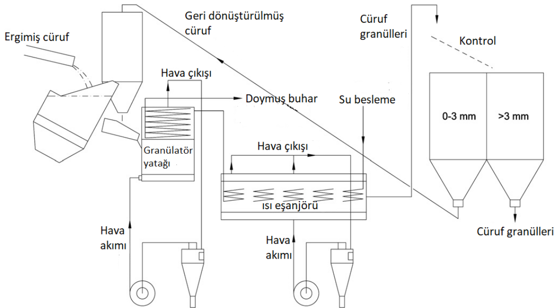
Şekil 1.12 Katı cüruf çarpması yöntemi [27]
