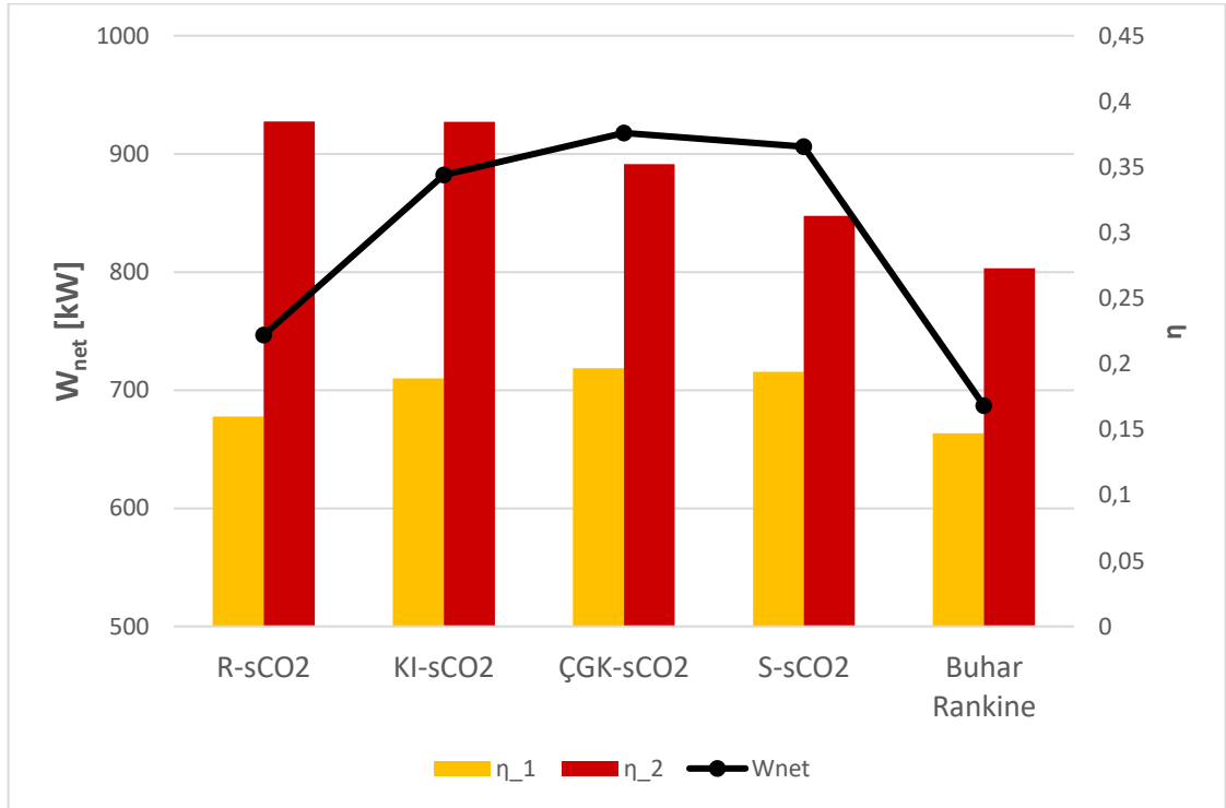
Şekil 3.27 Çevrimlerin verim ve güç çıktısına göre karşılaştırılması
