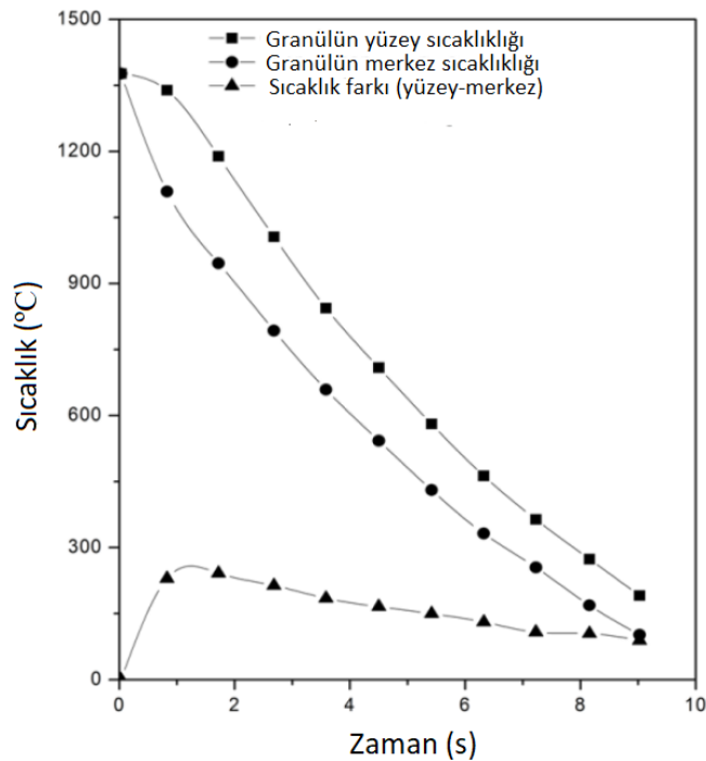
Şekil 1.6 5 mm çapındaki YFC granülünün zamana bađlı sıcaklık deđişim grafiđi [21]
