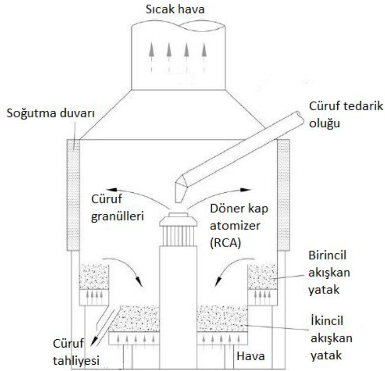
Şekil 1.15 Pickering tarafından geliştirilen döner kap atomizeri [27]
