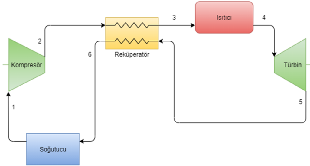
Şekil 1.24 Rejenerasyonlu sCO 2 Brayton çevrimi
