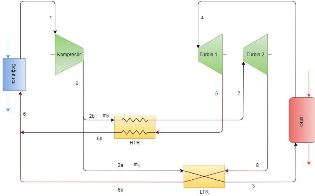
Şekil 3.7 ÇGK-sCO 2 çevriminin şematik gösterimi
