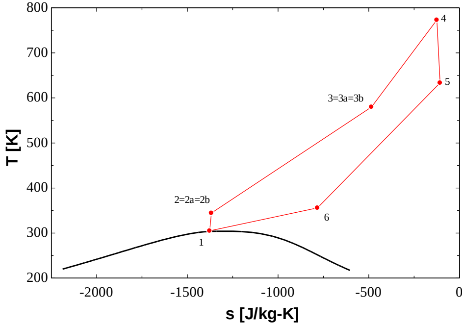
Şekil 3.4 KI-sCO 2 çevriminin T-s grafiği
