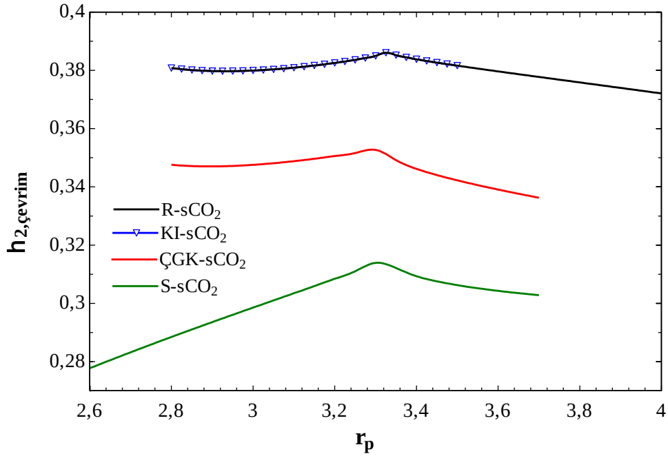
Şekil 3.16 25 MPa maksimum basınçta basınç oranının çevrimin \eta_{2,çevrim} değerine etkisi
