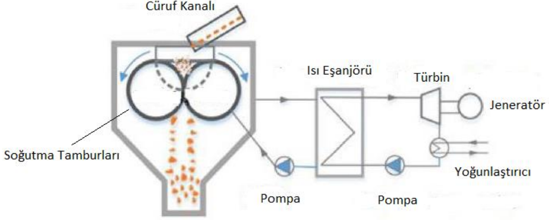
Şekil 1.10 İkiz tambur işleminin şematik gösterimi [26]
