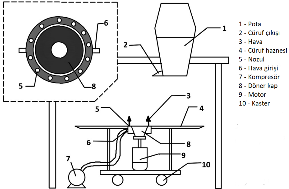
Şekil 1.16 Mizuochi tarafından geliştirilen RCA metodunun şematik gösterimi [7]
