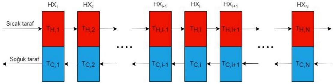
Şekil 3.9 Karşı akışlı ısı eşanjörünün alt bölümlere ayrılması
