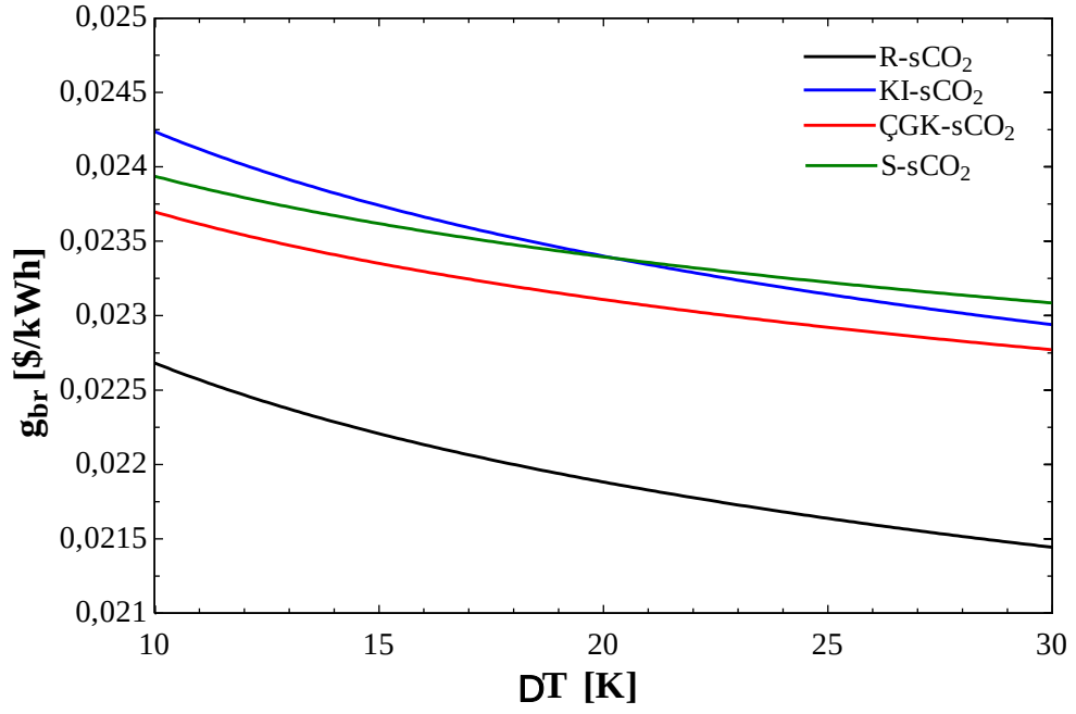
Şekil 3.38 Çevrimlerin \Delta T -birim elektrik üretim maliyeti
