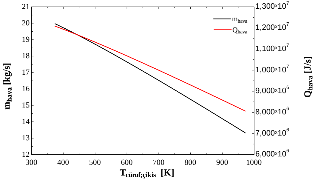
Şekil 2.3 YFC çıkış sıcaklığının, havanın kütleli debisine ve kazandığı enerji miktarına etkisi
