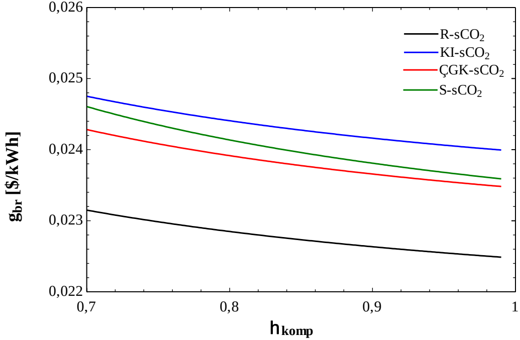
Şekil 3.34 Kompresör izantropik veriminin birim elektrik üretim maliyetine etkisi
