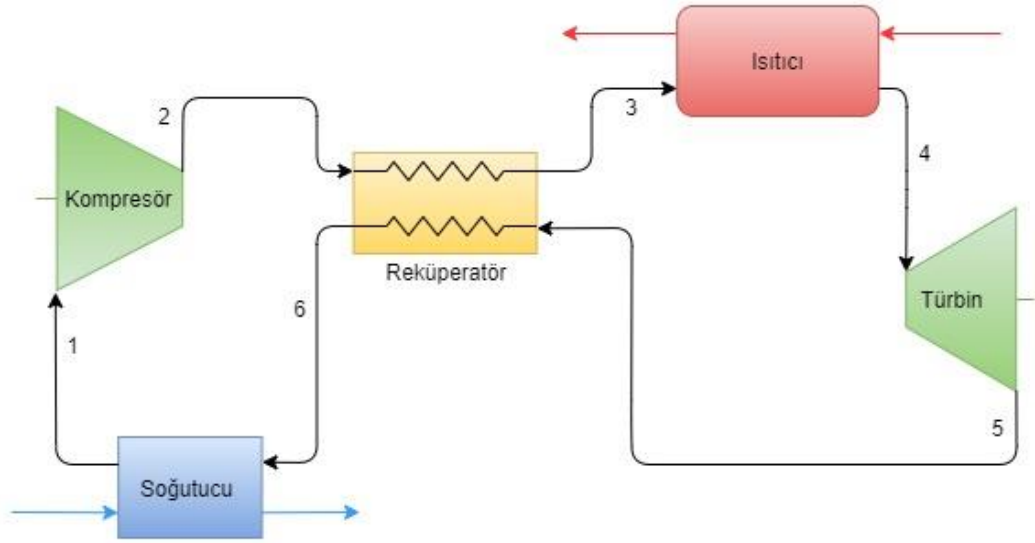
Şekil 3.1 R-sCO 2 çevriminin şematik gösterimi
