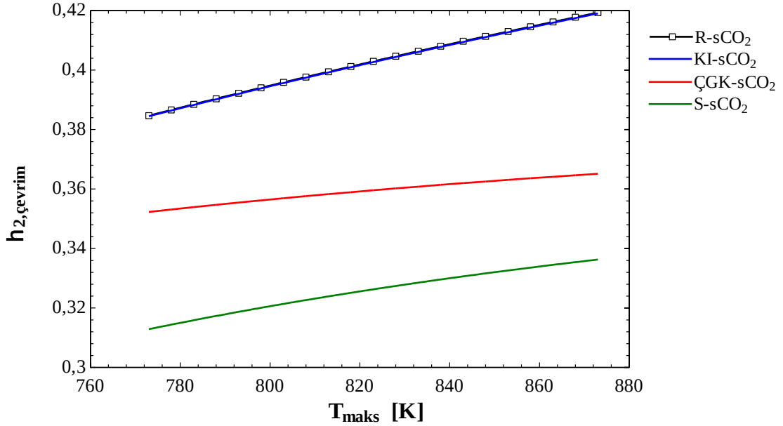
Şekil 3.21 sCO 2 çevrimlerinin \eta_{2,çevrim} -maksimum sıcaklık
