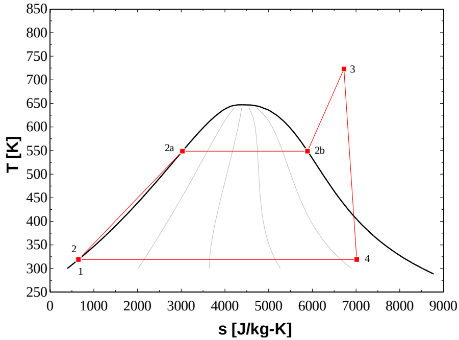
Şekil 3.11 Buhar Rankine çevriminin T-s grafiği
