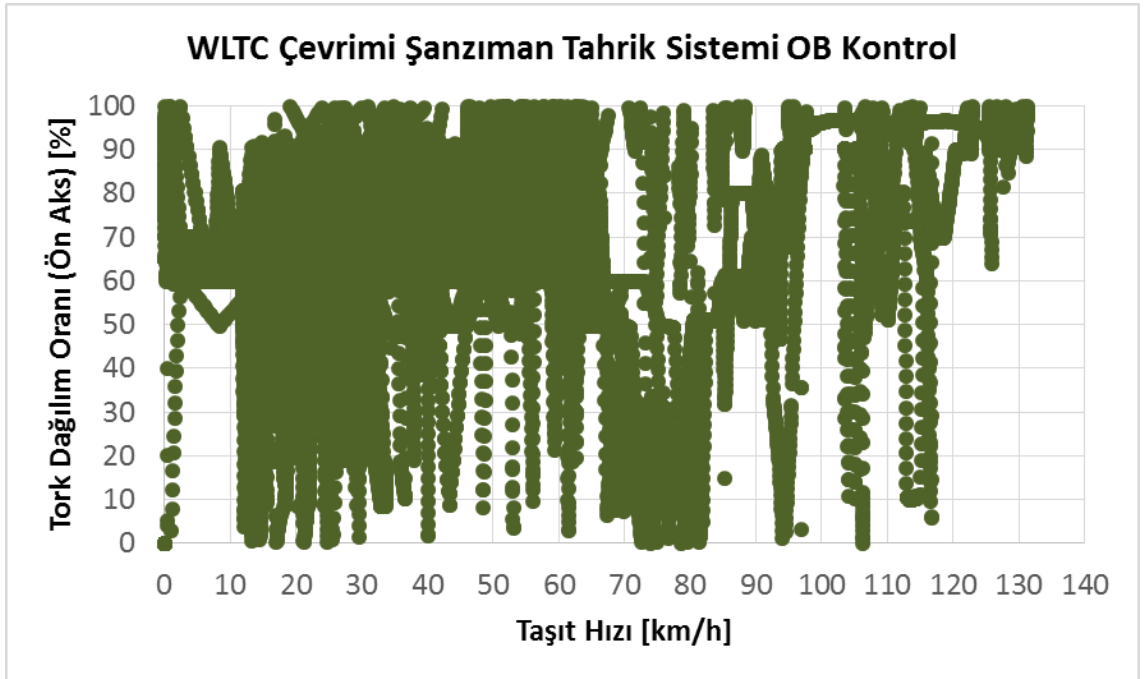
Şekil 4.32 WLTC çevriminde şanzımanlı tahrik sistemi optimizasyon bazlı kontrolde ön aks tork dağılım oranları
