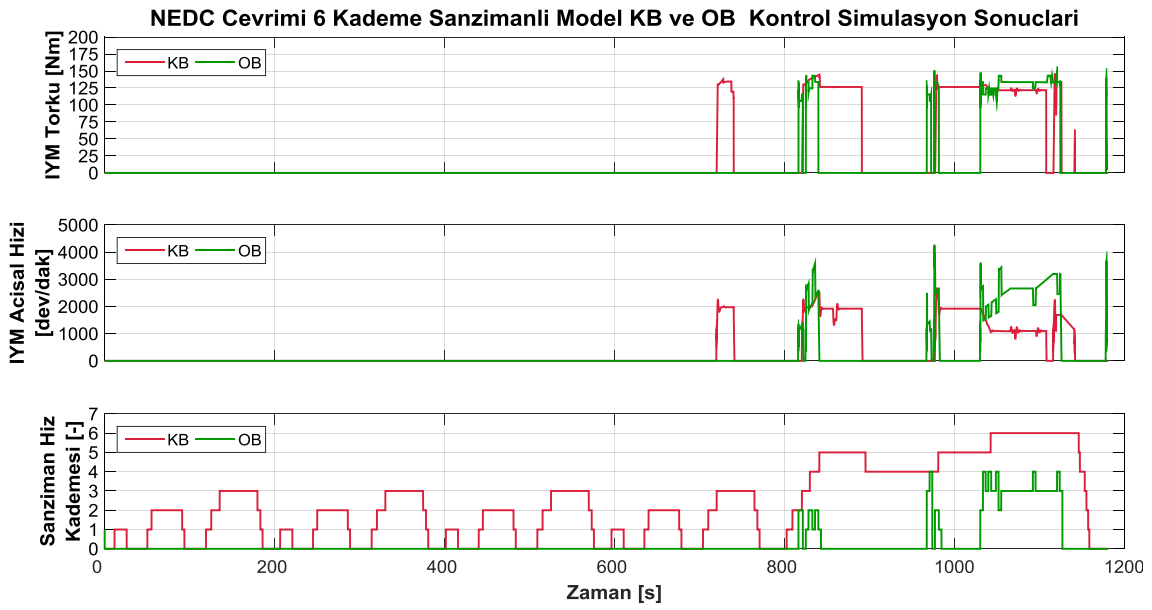
Şekil 4.10 NEDC çevriminde şanzımanlı tahrik sistemi şanzıman hız kademesi İYM açısal hızı ve torku
