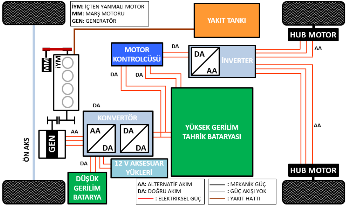
Şekil 1.10 Seri hibrit elektrikli taşıtlar için teker tipi (Wheel -Hub) elektrik motoru uygulaması
