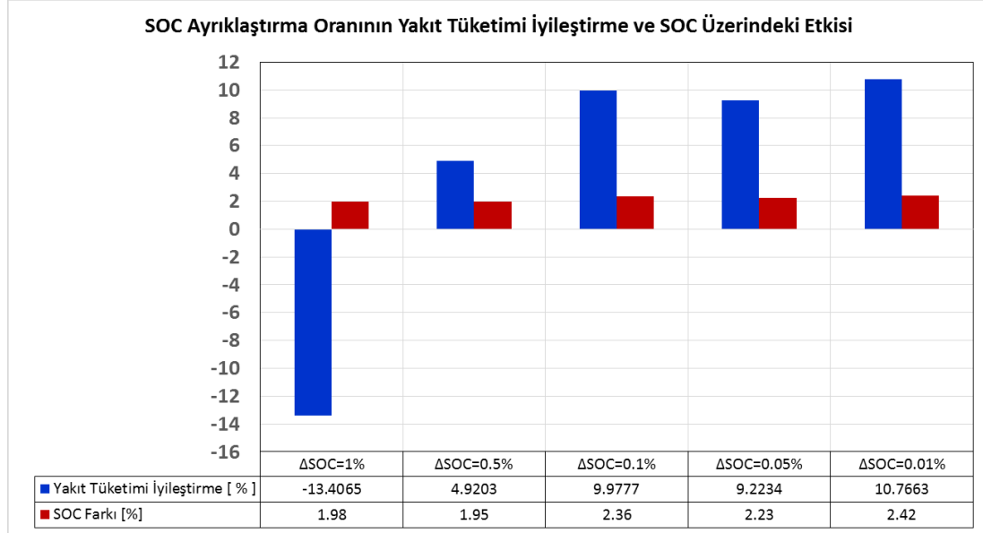
Şekil 4.54 FTP-72 çevriminde baz tahrik sistemi optimizasyon bazlı kontrolde SOC ayırıklaştırma oranının yakıt tüketimi ve son SOC üzerindeki etkisi
