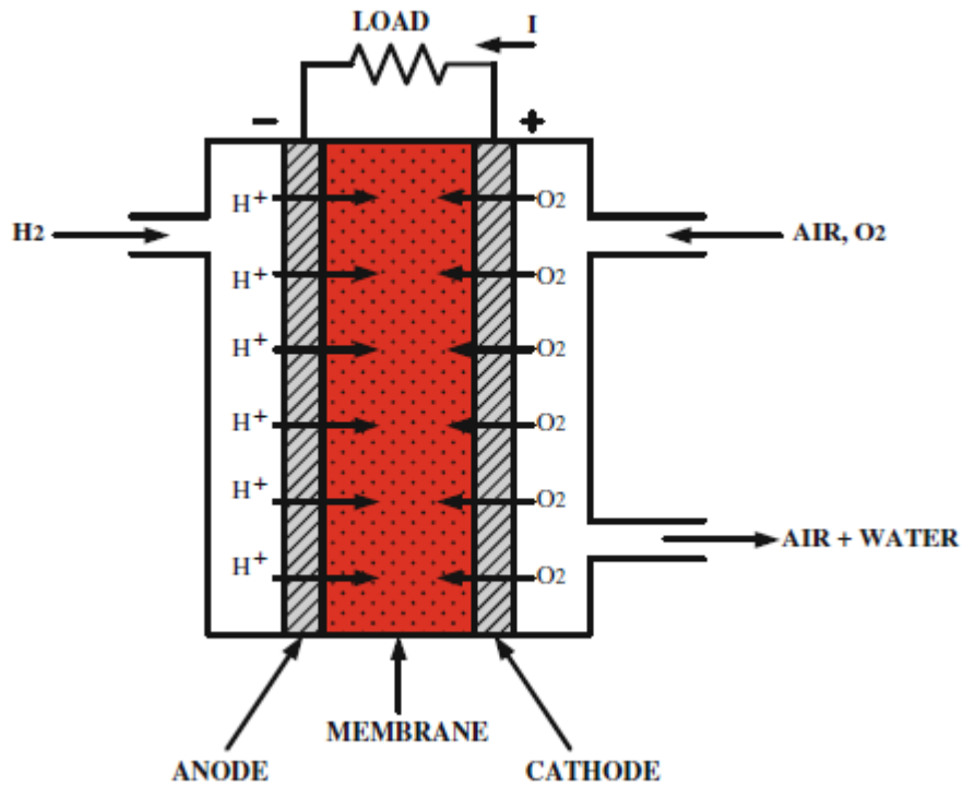
Şekil 1.7 PEM tipi yakıt hücresi çalışma prensibi [26]
