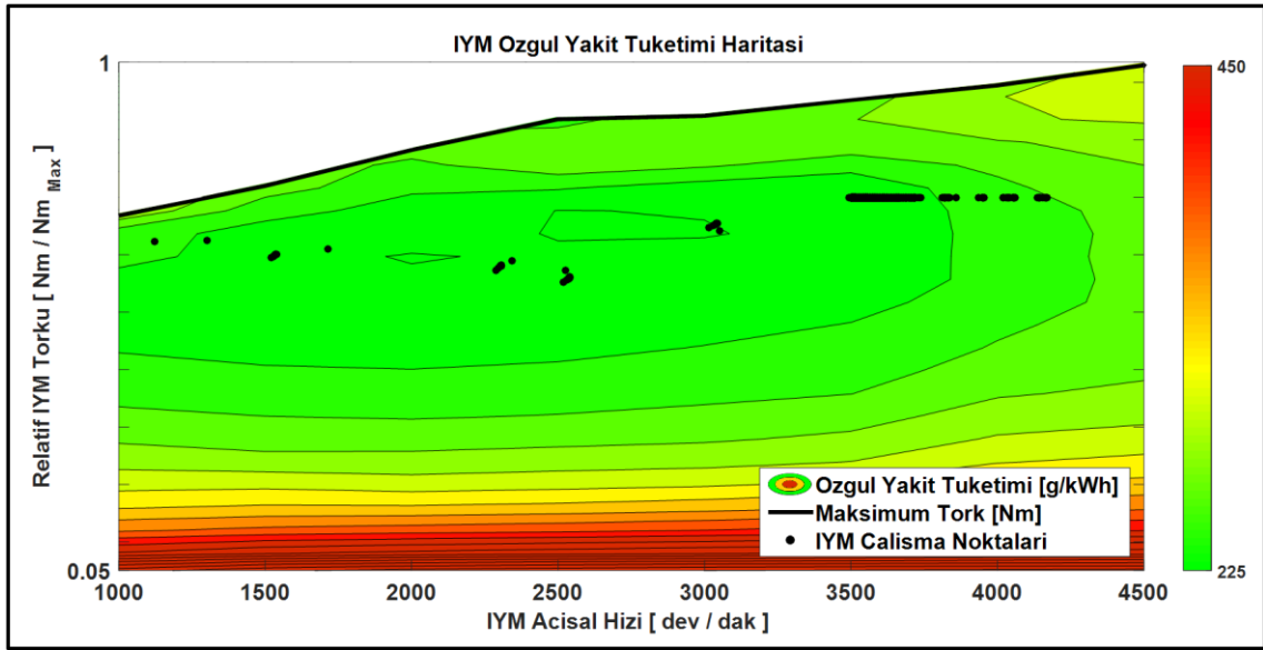
Şekil 4.41 FTP-72 çevriminde baz tahrik sistemi optimizasyon bazlı kontrolde İYM çalışma noktaları
