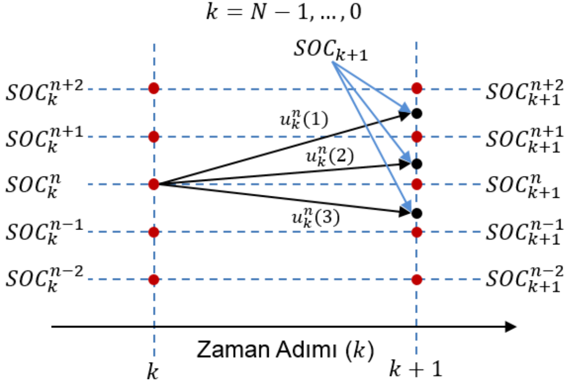
Şekil 3.5 Geriye dönük hesaplamada kullanılan interpolasyon
