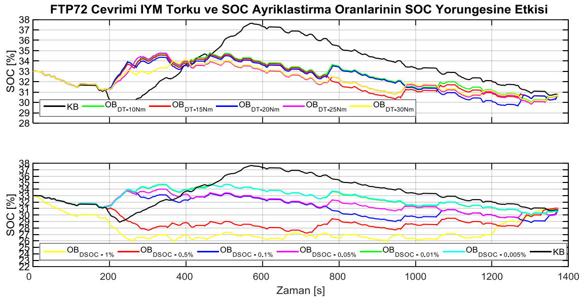
Şekil 4.52 FTP-72 çevriminde baz tahrik sistemi optimizasyon bazlı kontrolde İYM torku ve SOC ayırıklaştırma oranlarının SOC yörüngesine etkisi
