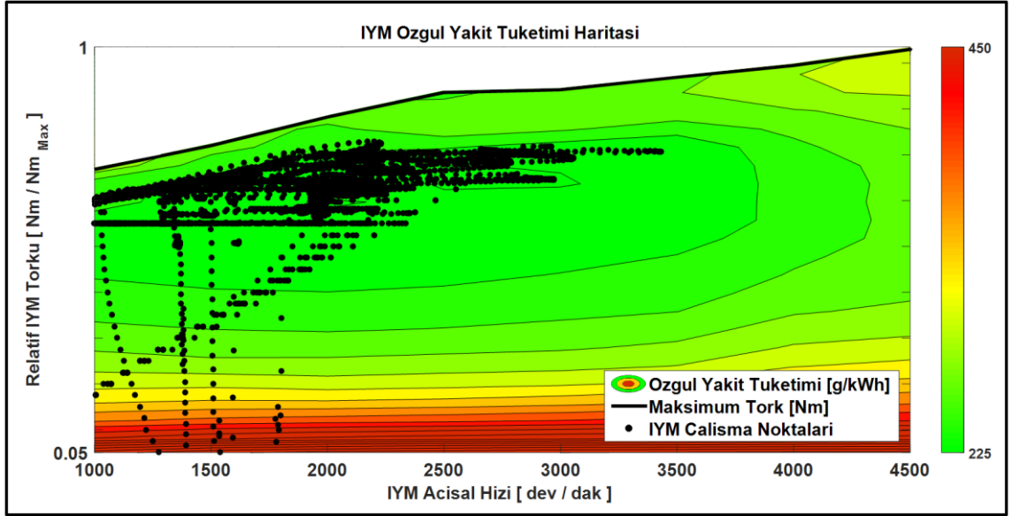
Şekil 4.30 WLTC çevriminde şanzımanlı tahrik sistemi kural bazlı kontrolde İYM çalışma noktaları
