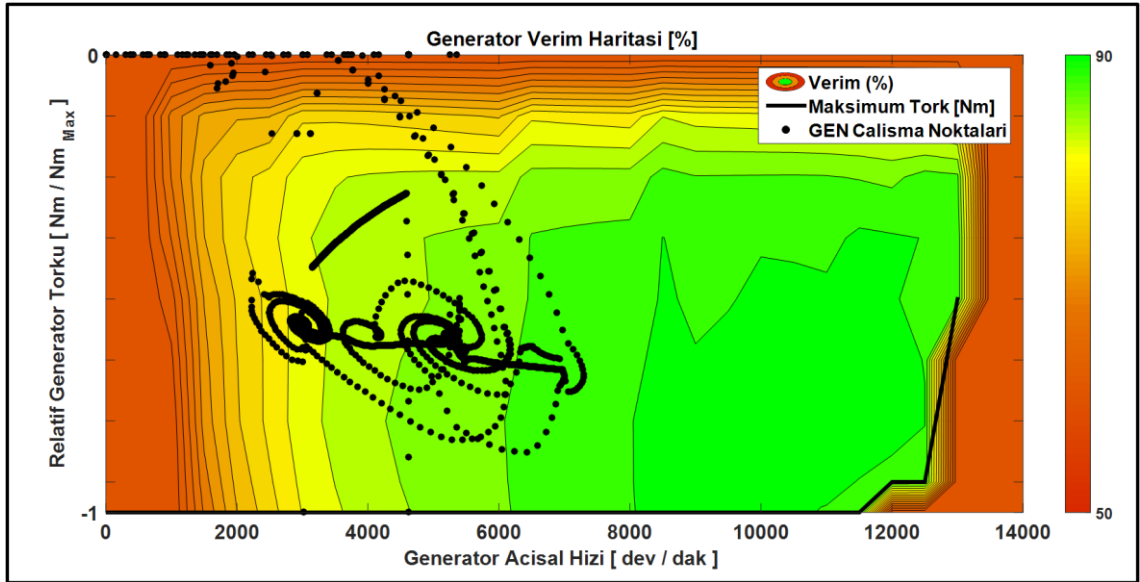
Şekil 4.14 NEDC çevriminde şanzımanlı tahrik sistemi kural bazlı kontrolde GEN çalışma noktaları
