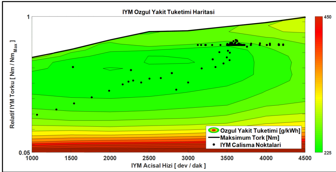
Şekil 4.7 NEDC çevriminde baz tahrik sistemi optimizasyon bazlı kontrolde İYM çalışma noktaları
