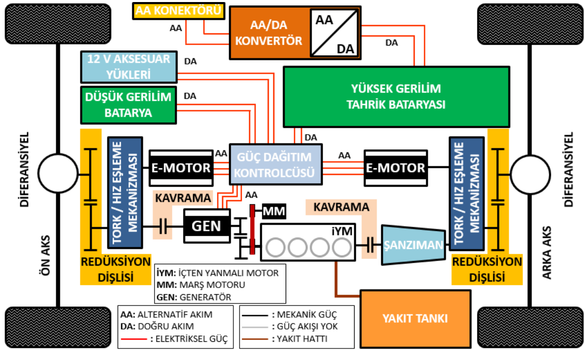
Şekil 1.15 Kompleks hibrit elektrikli taşıt mimarisi
