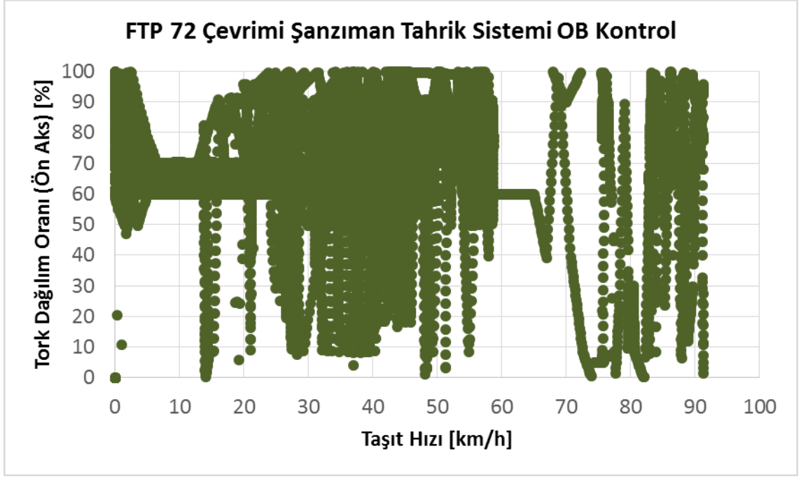
Şekil 4.49 FTP-72 çevriminde şanzımanlı tahrik sistemi optimizasyon bazlı kontrolde ön aks tork dağılım oranları
