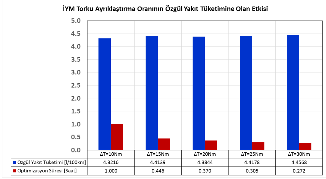
Şekil 4.55 FTP-72 çevriminde baz tahrik sistemi optimizasyon bazlı kontrolde İYM torku ayırıklaştırma oranının özgöl yakıt tüketimi ve optimizasyon süresi üzerindeki etkisi
