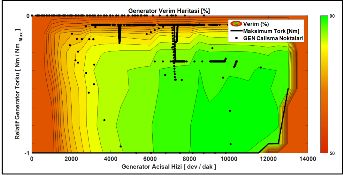
Şekil 4.17 NEDC çevriminde şanzımanlı tahrik sistemi optimizasyon bazlı kontrolde GEN çalışma noktaları
