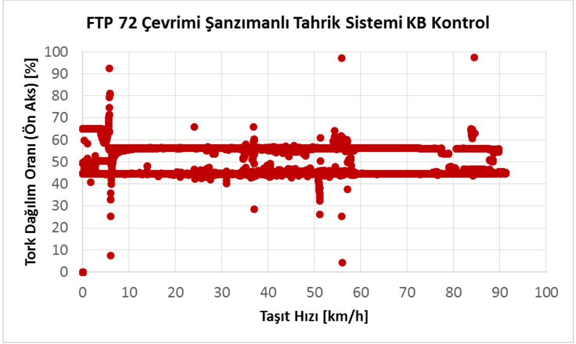
Şekil 4.46 FTP-72 çevriminde şanzımanlı tahrik sistemi kural bazlı kontrolde ön aks tork dağılım oranları
