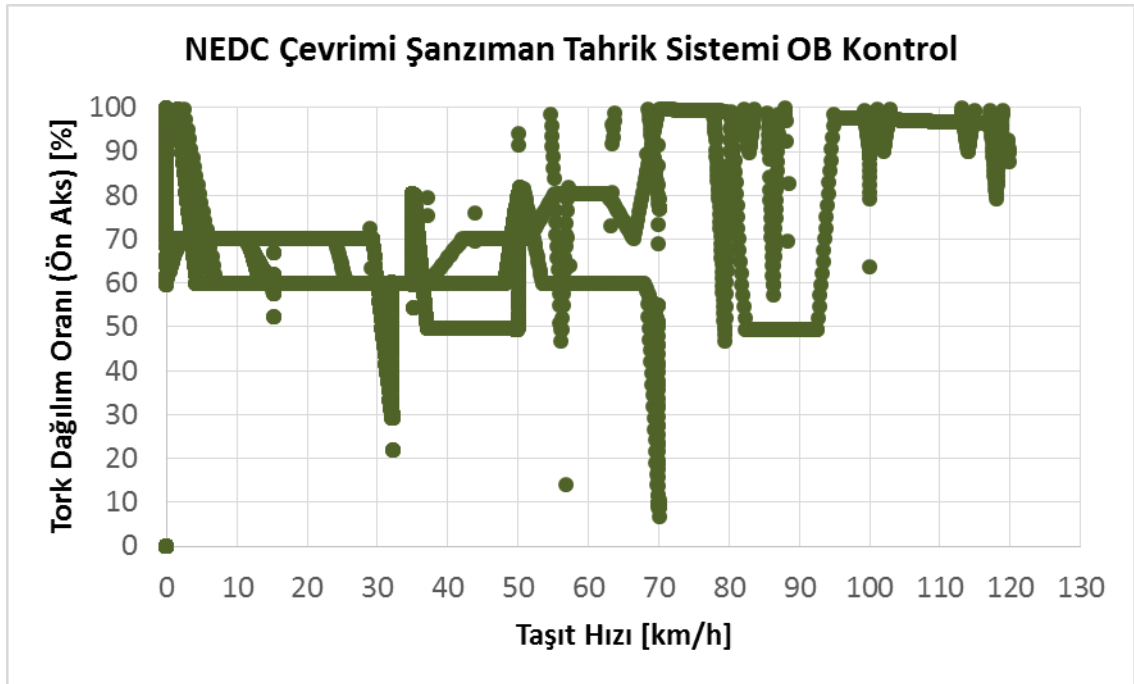
Şekil 4.15 NEDC çevriminde şanzımanlı tahrik sistemi optimizasyon bazlı kontrolde ön aks tork dağılım oranı
