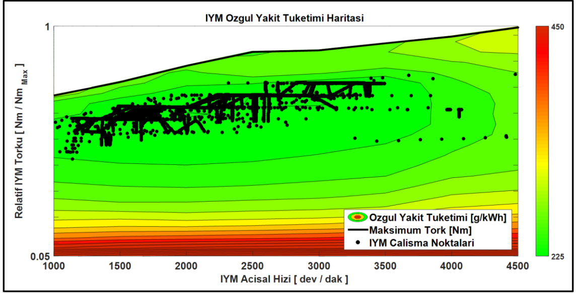
Şekil 4.33 WLTC çevriminde şanzımanlı tahrik sistemi optimizasyon bazlı kontrolde İYM çalışma noktaları
