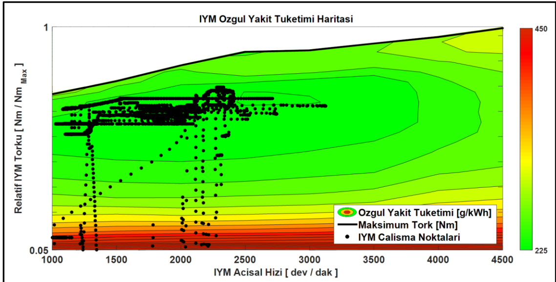
Şekil 4.38 FTP-72 çevriminde baz tahrik sistemi kural bazlı kontrolde İYM çalışma noktaları
