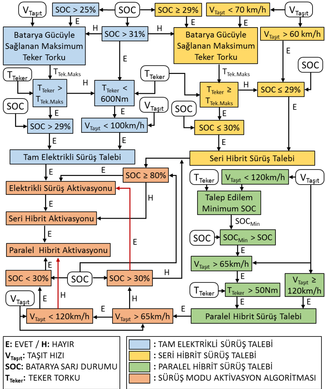
Şekil 2.7 Kontrol modeli temel algoritması
