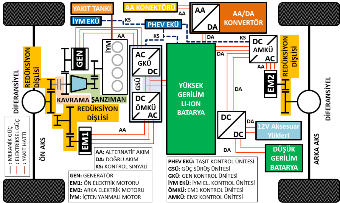
Şekil 3.9 6 ileri hız kademeli şanzımana sahip kompleks hibrit tahrik sistemi mimarisi
