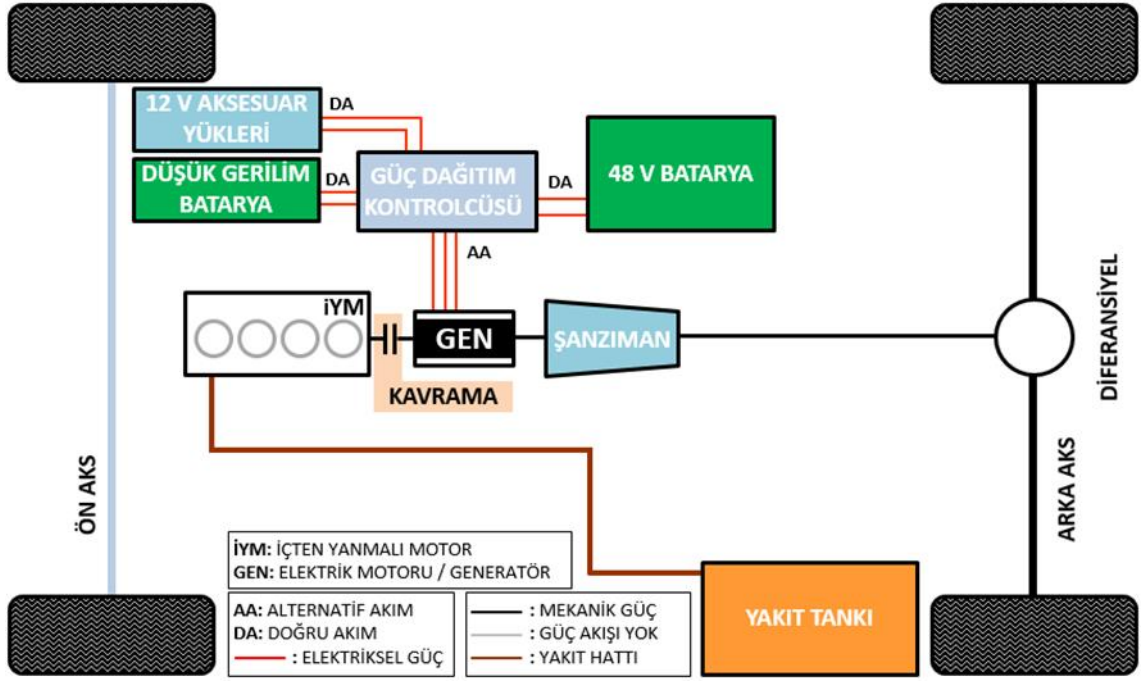
Şekil 1.13 Mild hibrit elektrikli taşıt mimarisi
