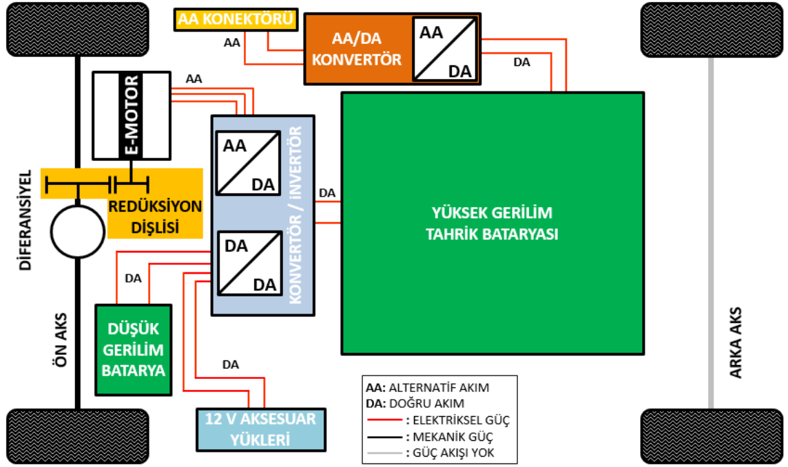
Şekil 1.6 Tam elektrikli taşıt (BEV) mimarisi
