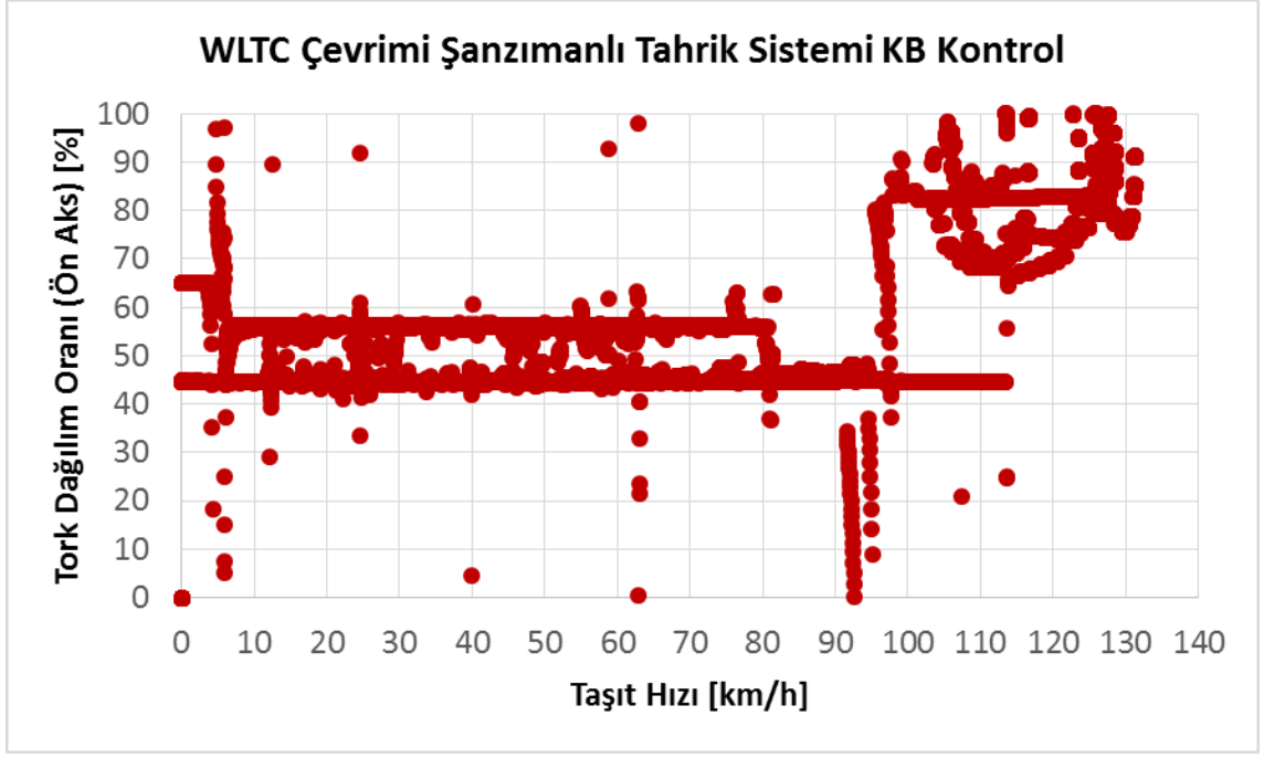
Şekil 4.29 WLTC çevriminde şanzımanlı tahrik sistemi kural bazlı kontrolde ön aks tork dağılım oranları
