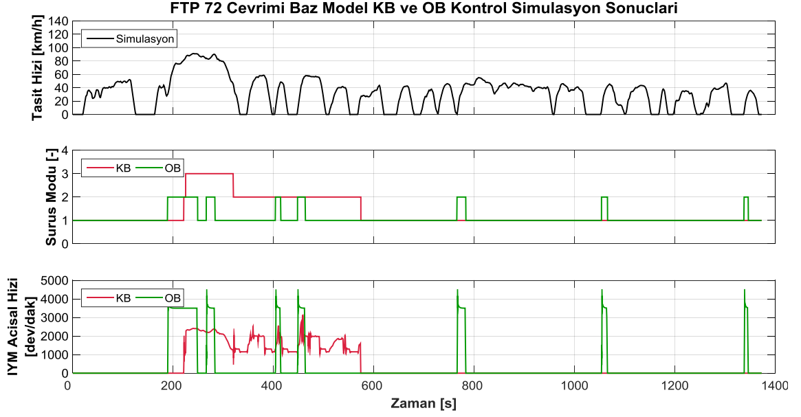
Şekil 4.35 FTP-72 çevriminde baz tahrik sistemi sürüş modu ve İYM açisal hızı
