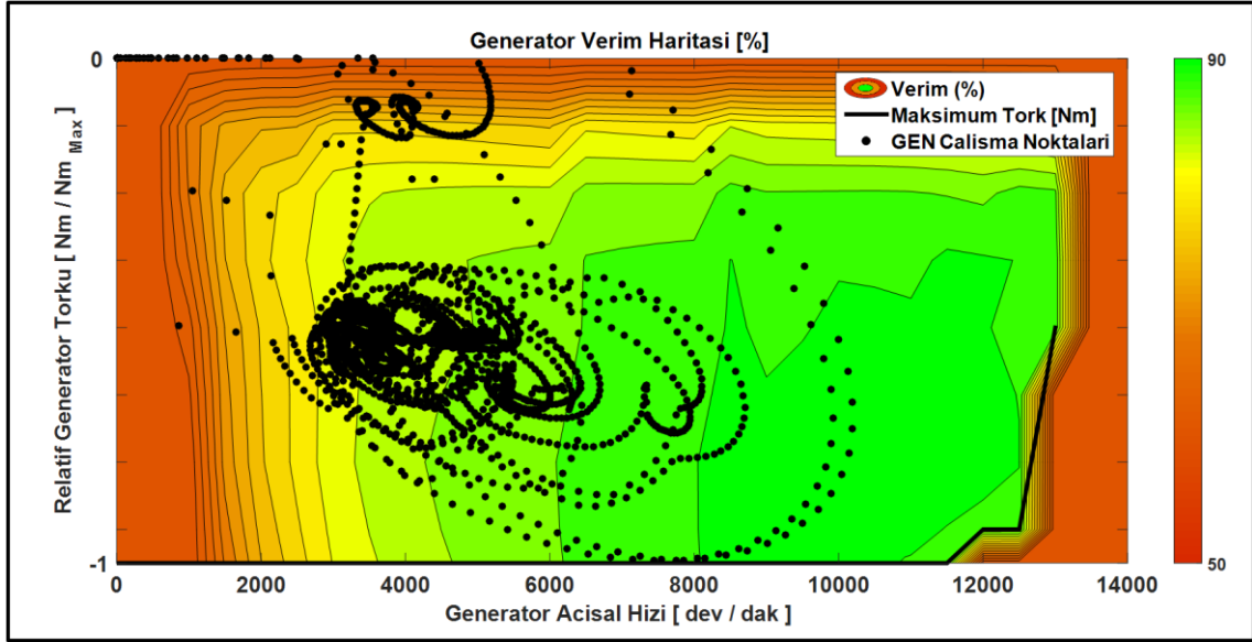
Şekil 4.48 FTP-72 çevriminde şanzımanlı tahrik sistemi kural bazlı kontrolde GEN çalışma noktaları
