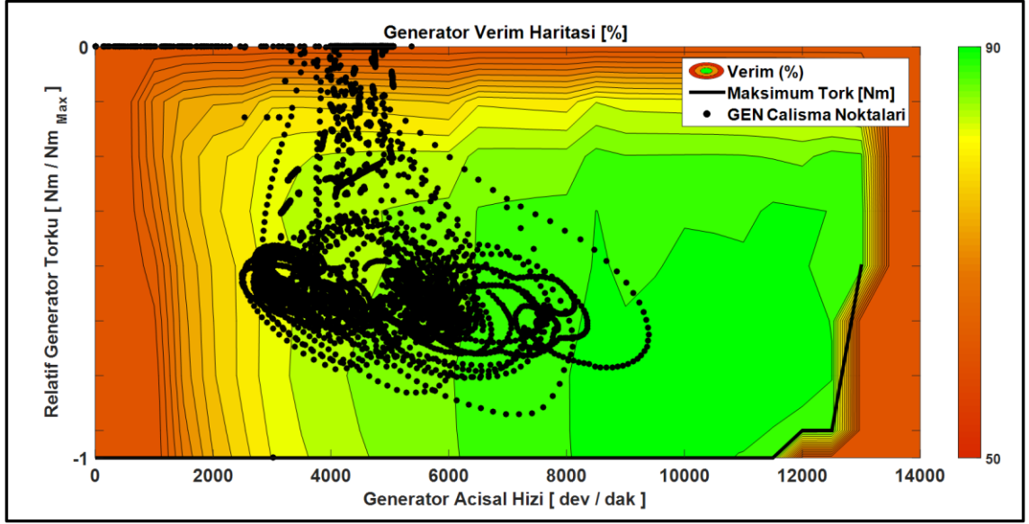
Şekil 4.31 WLTC çevriminde şanzımanlı tahrik sistemi kural bazlı kontrolde GEN çalışma noktaları
