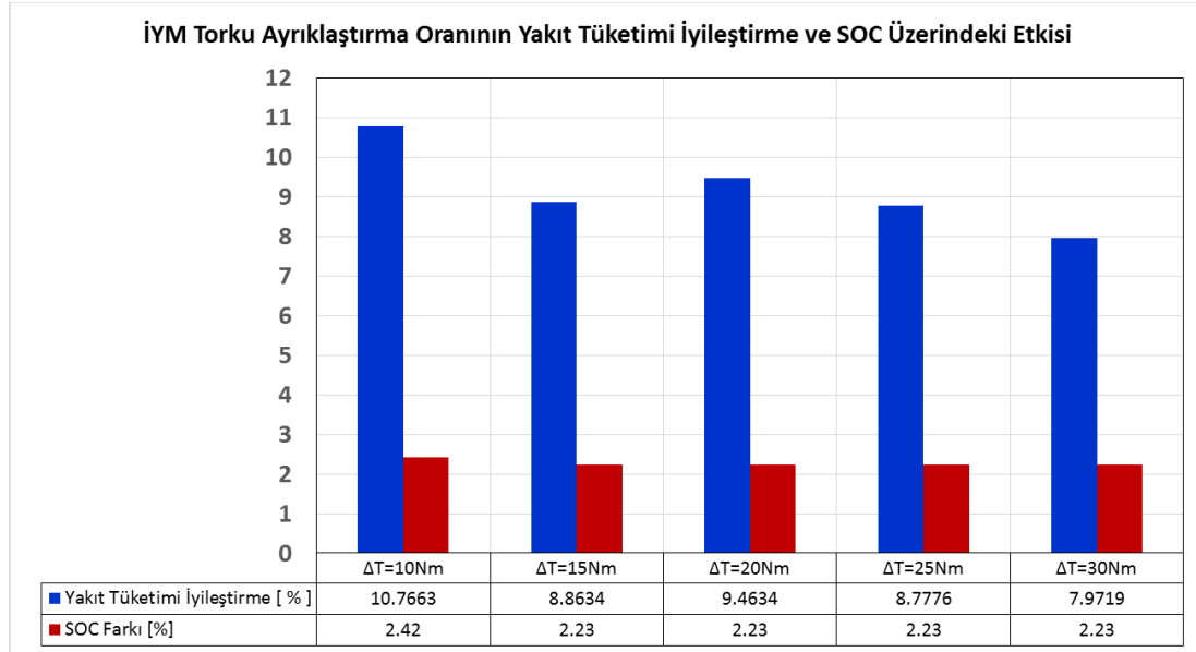
Şekil 4.53 FTP-72 çevriminde baz tahrik sistemi optimizasyon bazlı kontrolde İYM torku ayırıştırma oranının yakıt tüketimi ve son SOC üzerindeki etkisi
