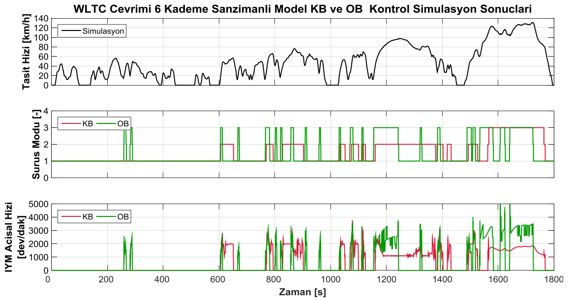
Şekil 4.26 WLTC çevriminde şanzımanlı tahrik sistemi sürüş modu ve İYM açısai hızı
