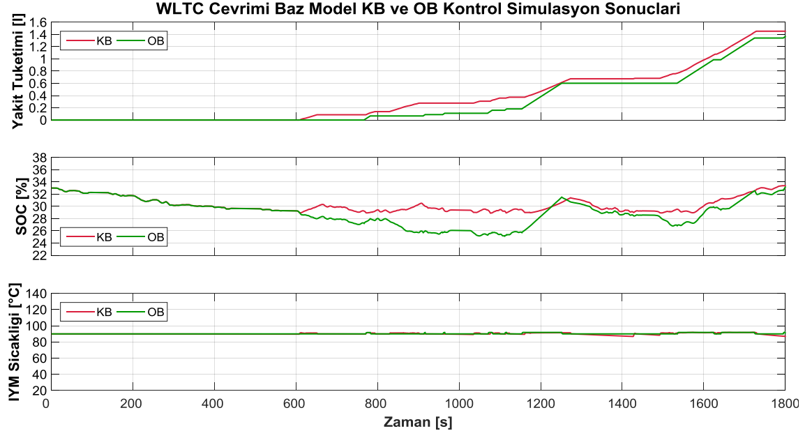
Şekil 4.19 WLTC çevriminde baz tahrik sistemi yakıt tüketimi, SOC ve İYM sıcaklığı
