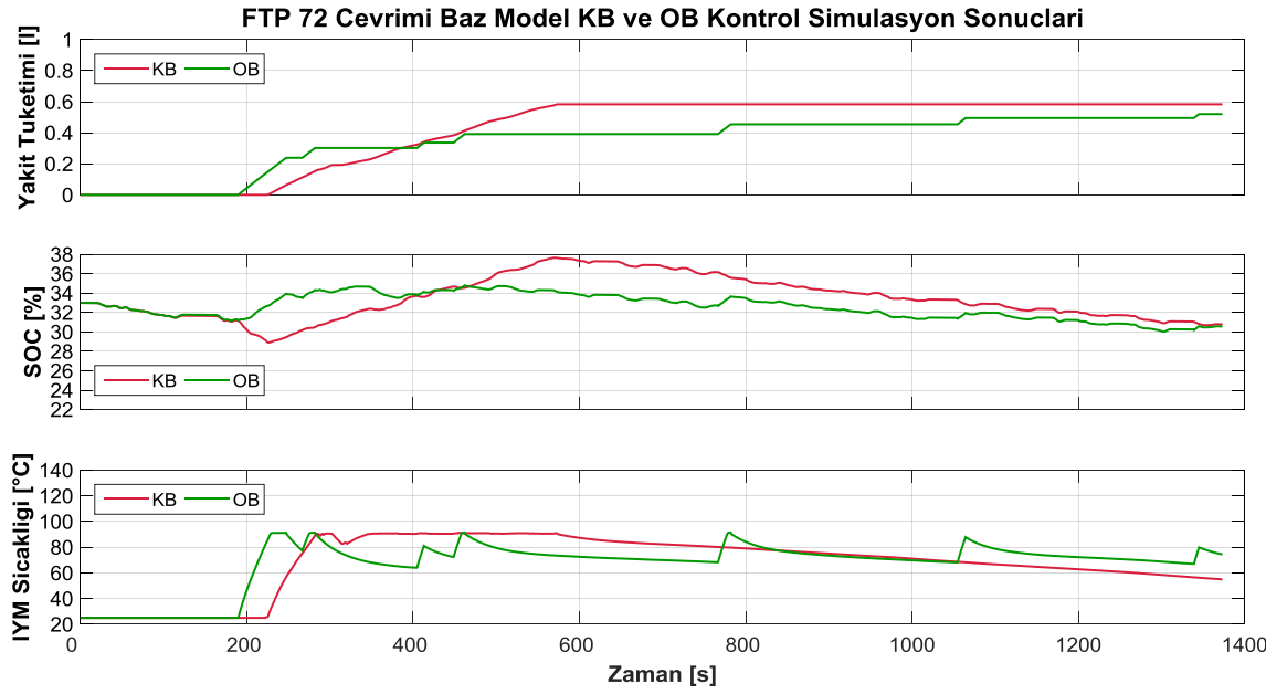
Şekil 4.36 FTP-72 çevriminde baz tahrik sistemi yakıt tüketimi, SOC ve İYM sıcaklığı
