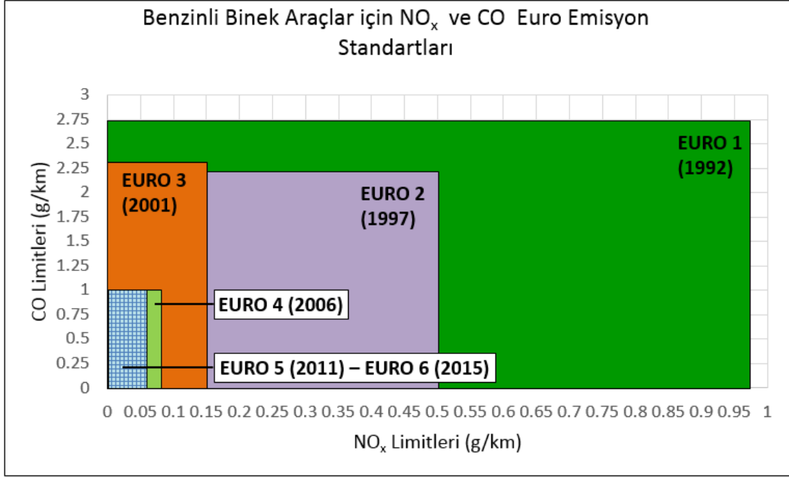
Şekil 1.4 Benzinli binek araçlarda NO x ve CO için Euro emisyon standartları 12
