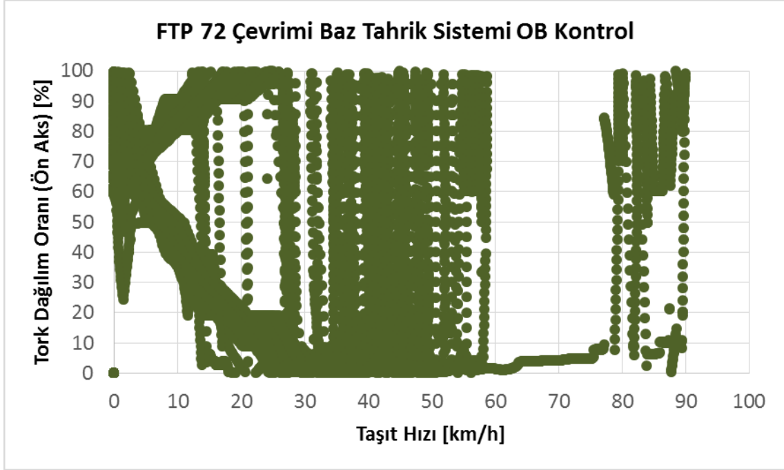
Şekil 4.40 FTP-72 çevriminde baz tahrik sistemi optimizasyon bazlı kontrolde ön aks tork dağılım oranları
