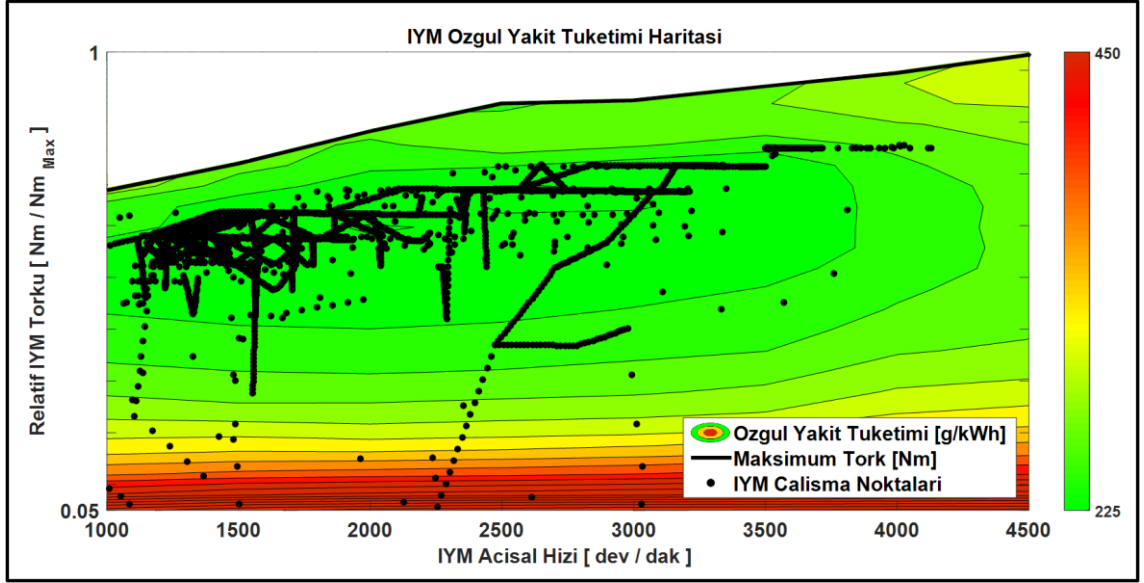
Şekil 4.50 FTP-72 çevriminde şanzımanlı tahrik sistemi optimizasyon bazlı kontrolde İYM çalışma noktaları
