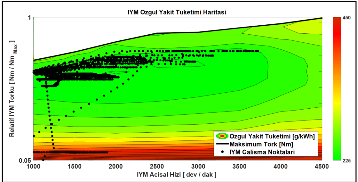
Şekil 4.47 FTP-72 çevriminde şanzımanlı tahrik sistemi kural bazlı kontrolde İYM çalışma noktaları
