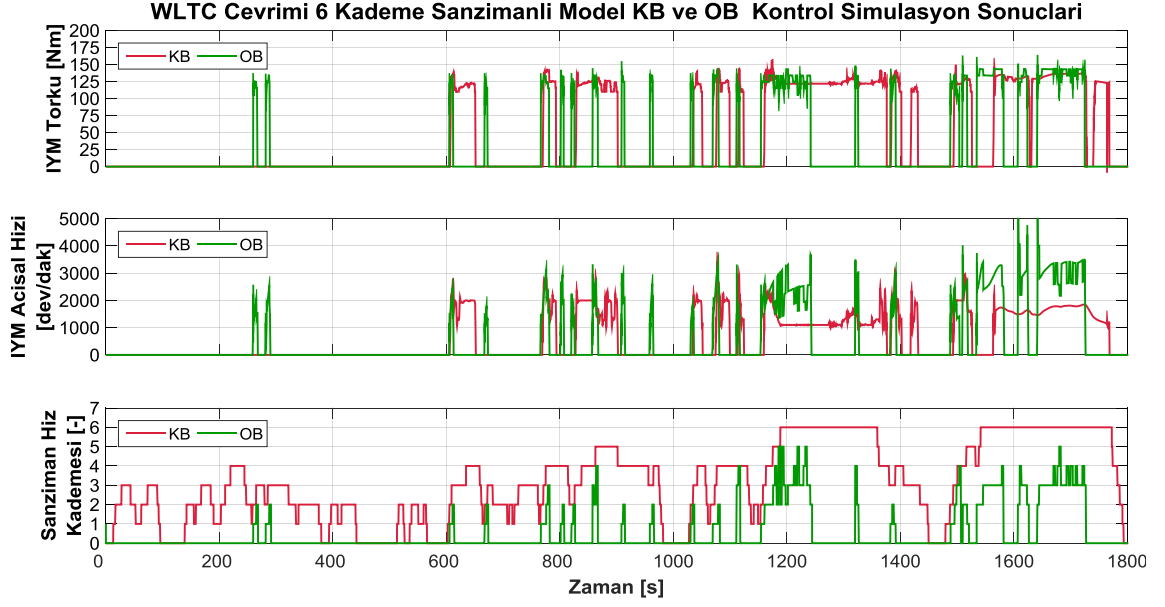
Şekil 4.27 WLTC çevriminde şanzımanlı tahrik sistemi şanzıman hız kademesi İYM açısal hızı ve torku
