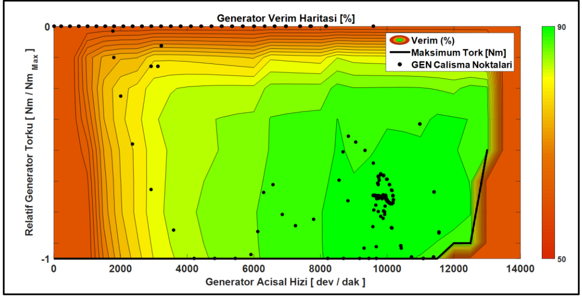
Şekil 4.8 NEDC çevriminde baz tahrik sistemi optimizasyon bazlı kontrolde GEN çalışma noktaları
