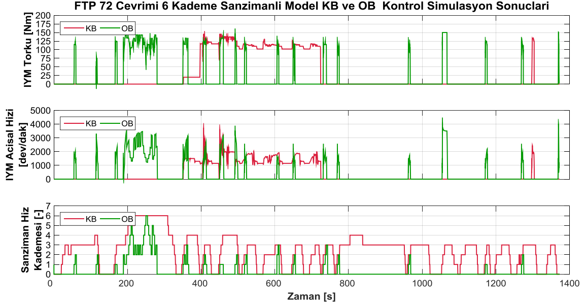
Şekil 4.45 FTP-72 çevriminde şanzımanlı tahrik sistemi şanzıman hız kademesi, İYM açısal hızı ve torku
