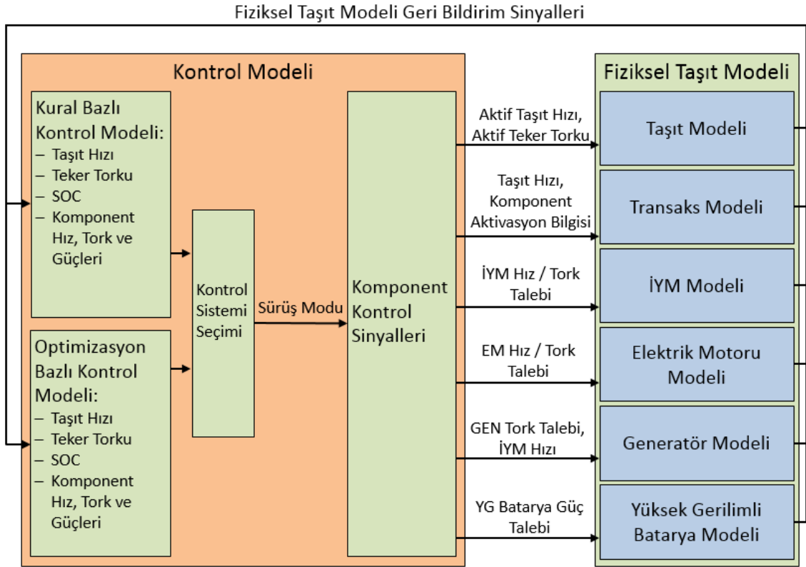
Şekil 2.6 Taşıt modeli
