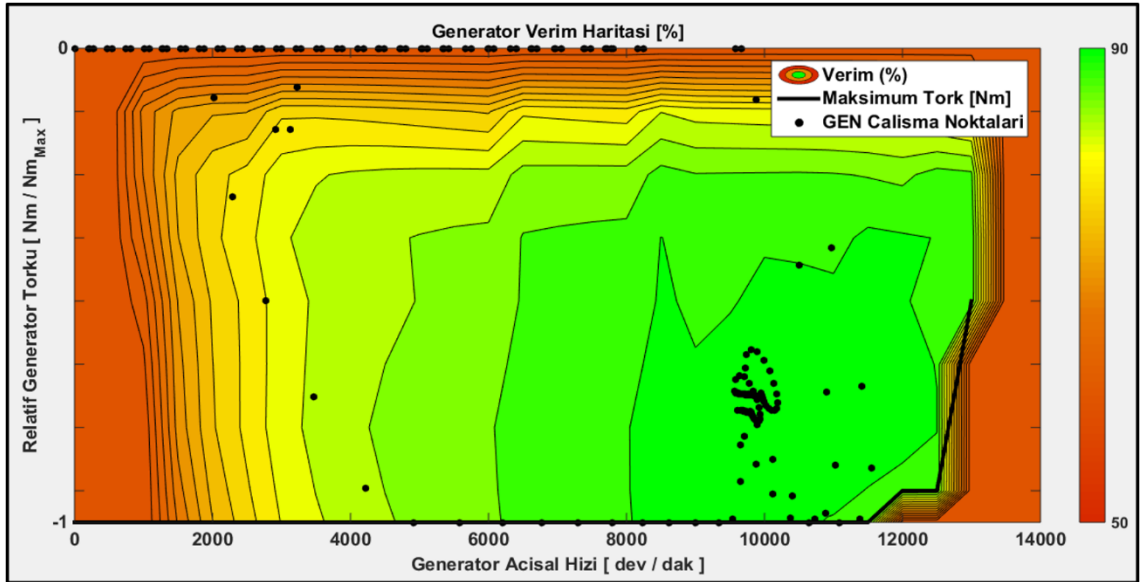
Şekil 4.25 WLTC çevriminde baz tahrik sistemi optimizasyon bazlı kontrolde GEN çalışma noktaları
