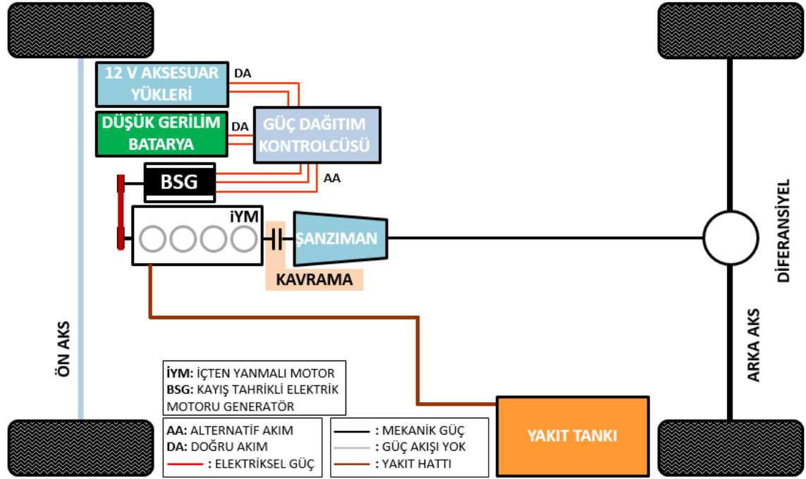
Şekil 1.12 Mikro hibrit elektrikli taşıt mimarisi
