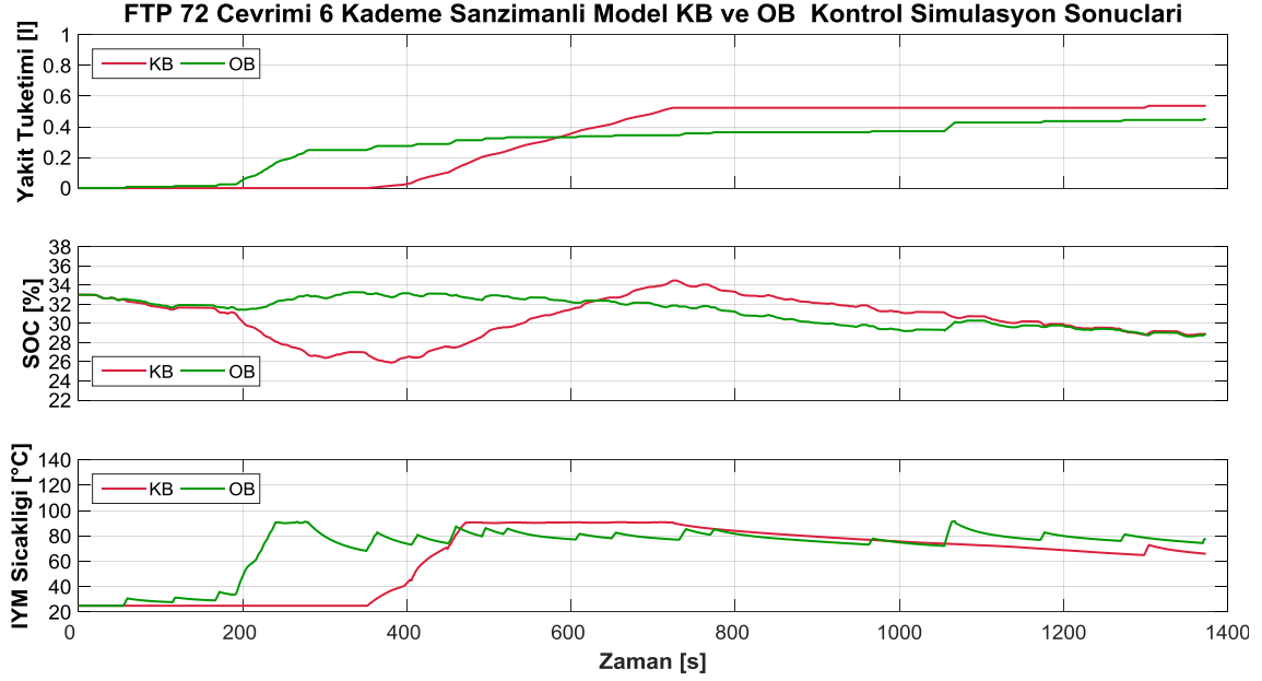
Şekil 4.44 FTP-72 çevriminde şanzımanlı tahrik sistemi yakıt tüketimi, SOC ve İYM sıcaklığı
