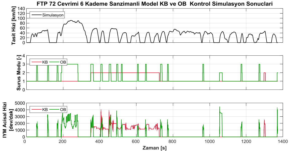
Şekil 4.43 FTP-72 çevriminde şanzımanlı tahrik sistemi sürüş modu ve İYM açısai hızı
