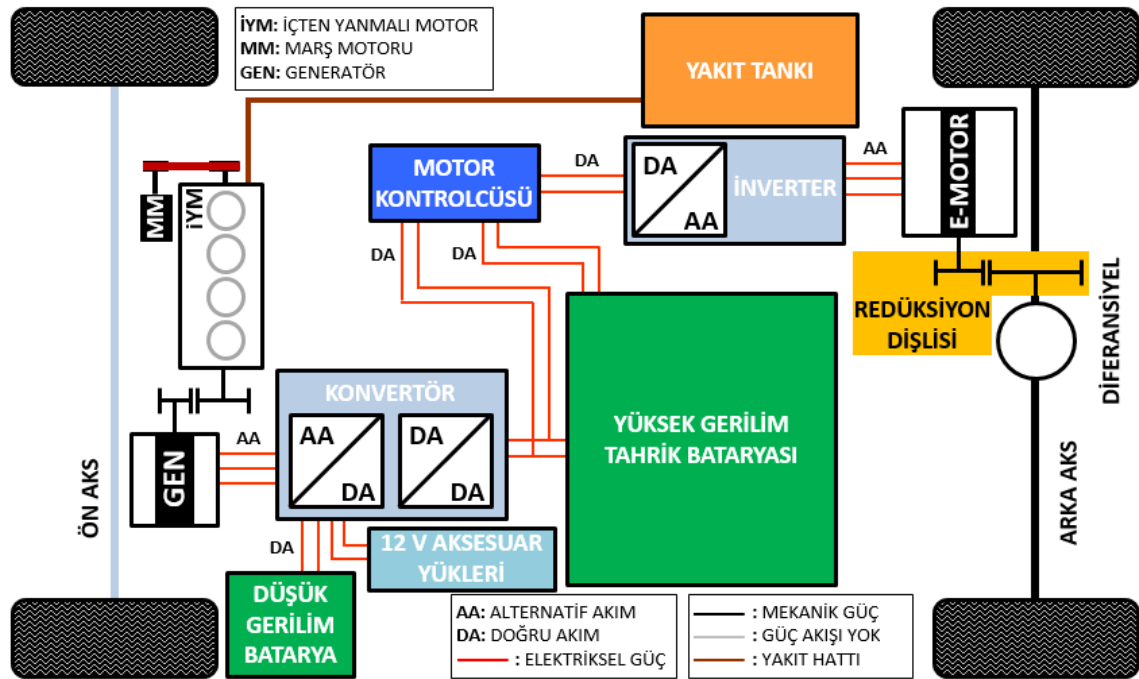
Şekil 1.9 Seri hibrit elektrikli taşıt mimarisi
