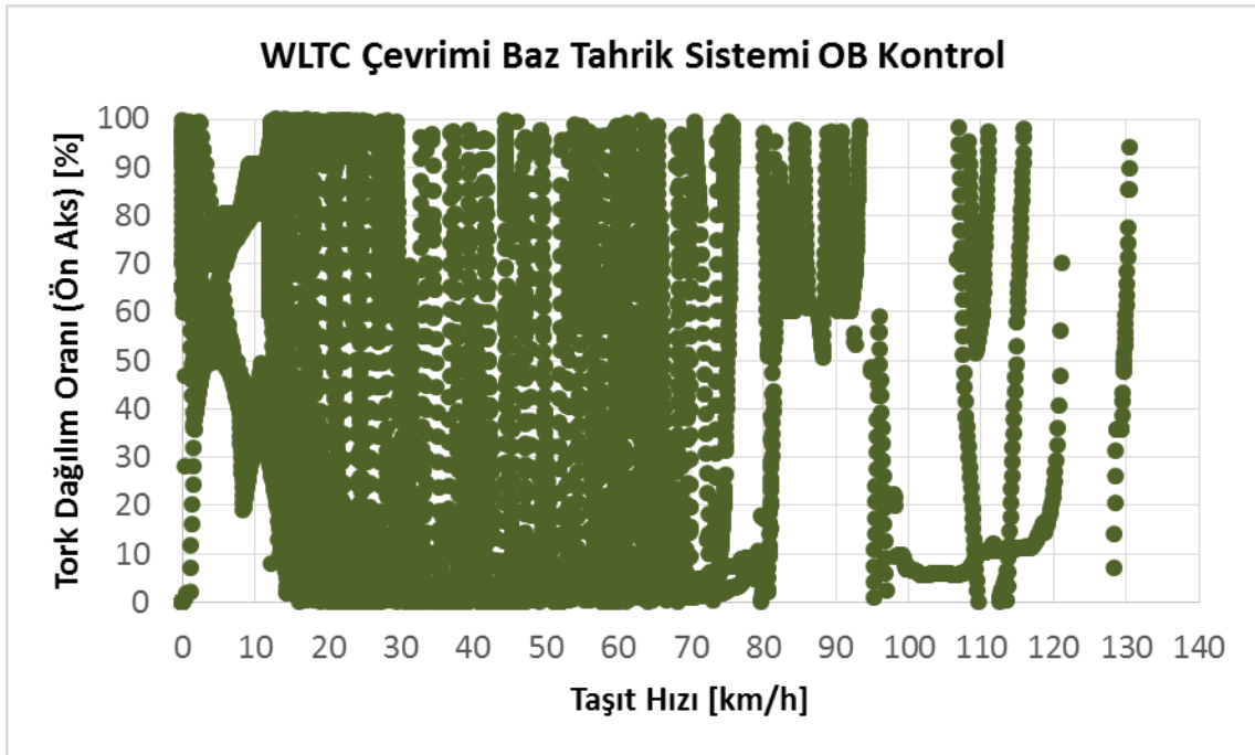
Şekil 4.23 WLTC çevriminde baz tahrik sistemi optimizasyon bazlı kontrolde ön aks tork dağılım oranları
