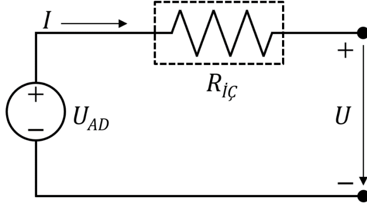
Şekil 2.8 Batarya modeli
