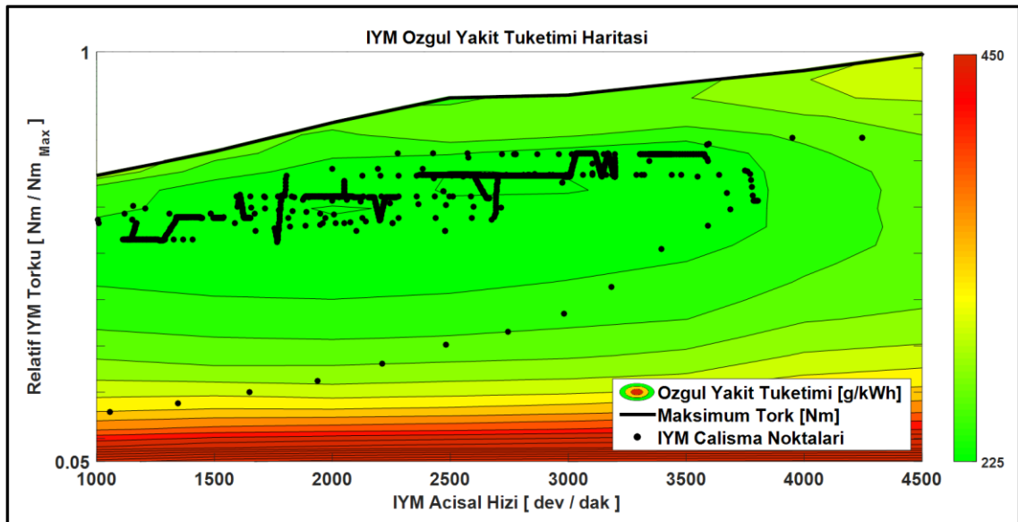
Şekil 4.16 NEDC çevriminde şanzımanlı tahrik sistemi optimizasyon bazlı kontrolde İYM çalışma noktaları
