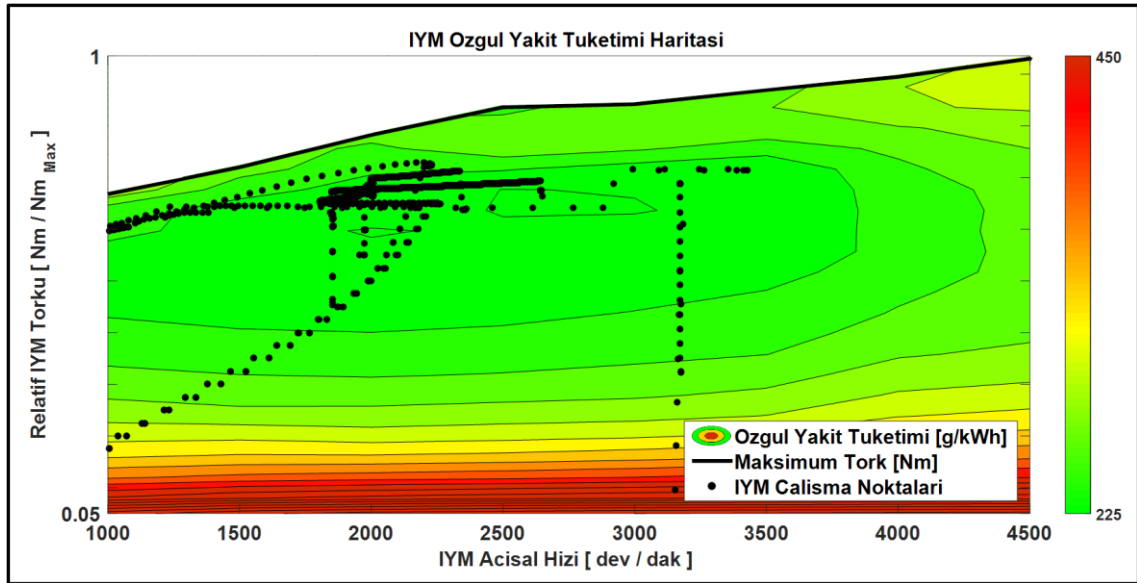
Şekil 4.4 NEDC çevriminde baz tahrik sistemi kural bazlı kontrolde İYM çalışma noktaları
