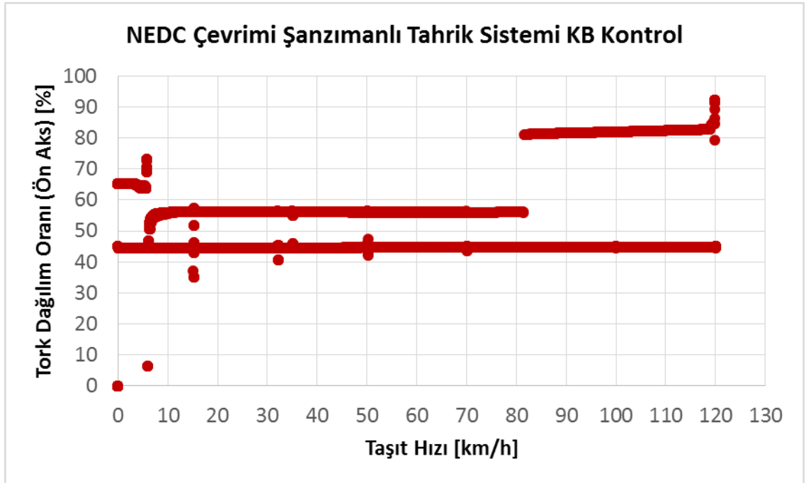
Şekil 4.12 NEDC çevriminde şanzımanlı tahrik sistemi kural bazlı kontrolde ön aks tork dağılım oranı
