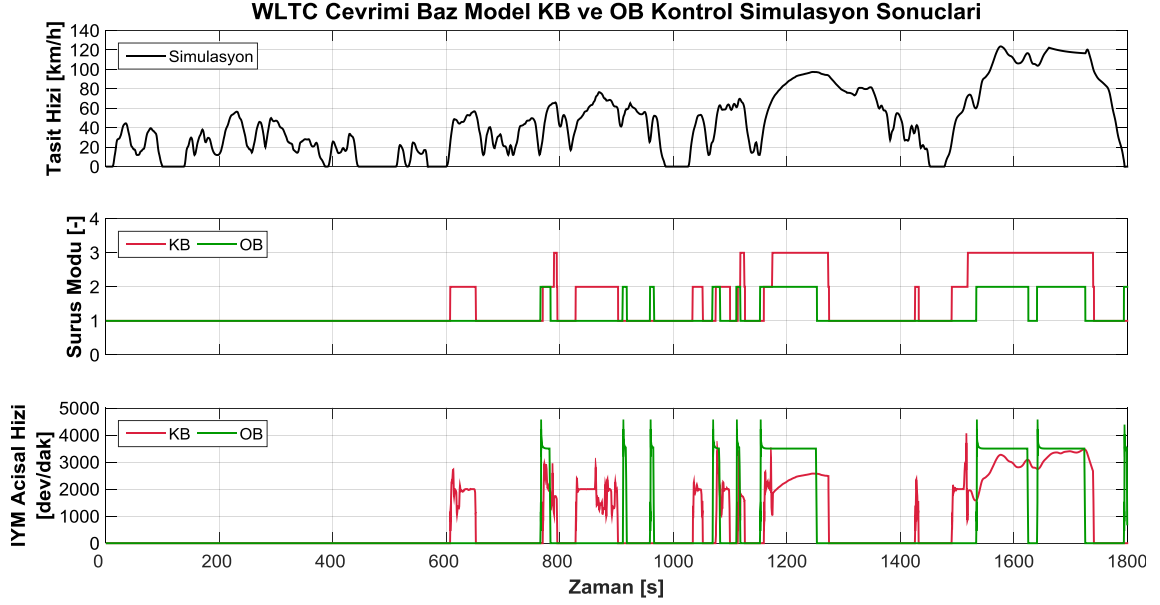
Şekil 4.18 WLTC çevriminde baz tahrik sistemi sürüş modu ve İYM açıl hızı
