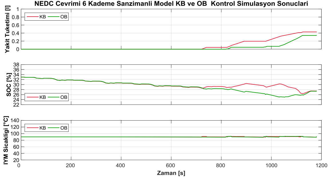
Şekil 4.11 NEDC çevriminde şanzımanlı tahrik sistemi yakıt tüketimi, SOC ve İYM sıcaklığı
