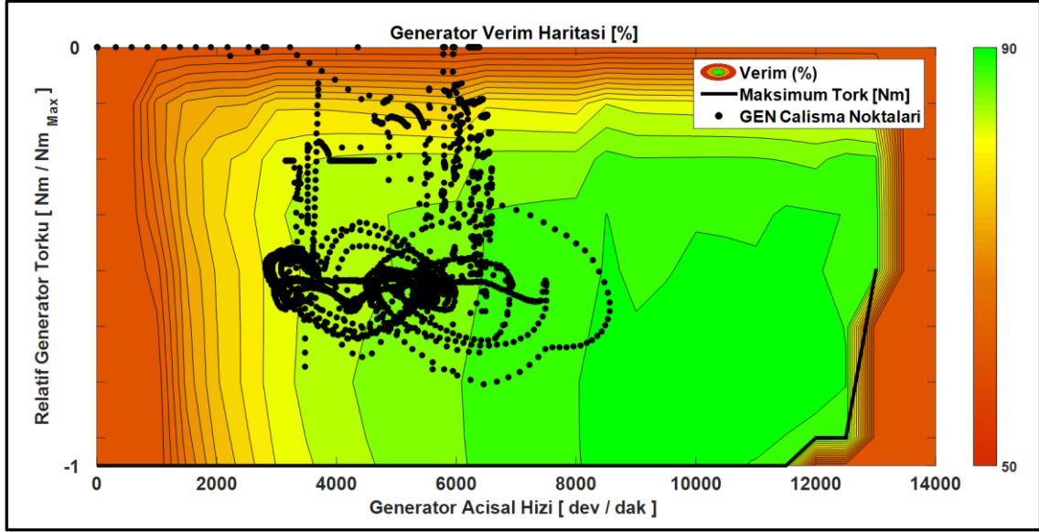
Şekil 4.39 FTP-72 çevriminde baz tahrik sistemi kural bazlı kontrolde GEN çalışma noktaları
