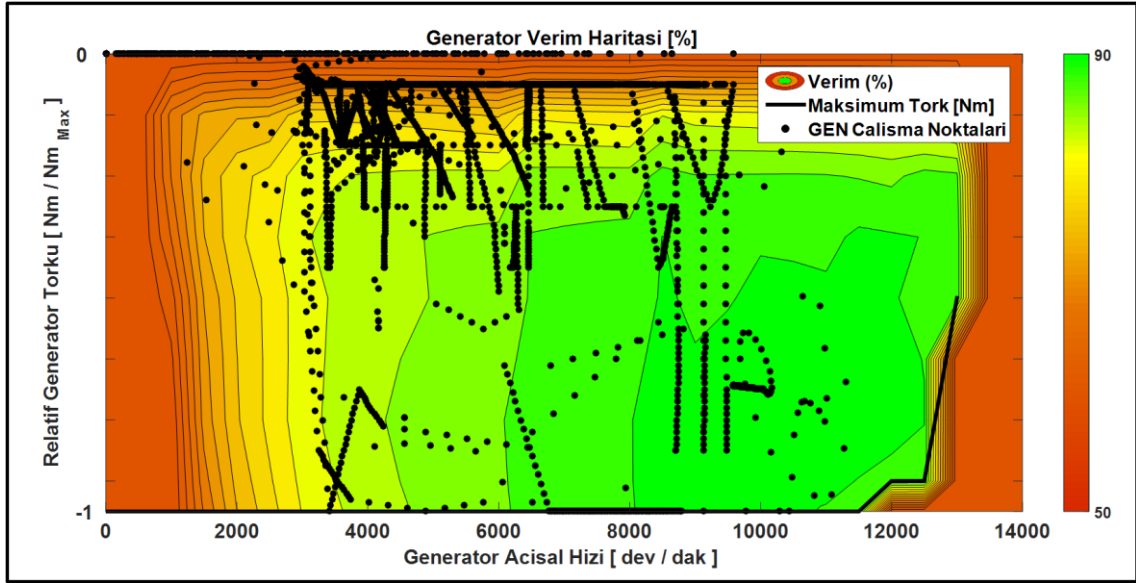
Şekil 4.51 FTP-72 çevriminde şanzımanlı tahrik sistemi optimizasyon bazlı kontrolde İYM çalışma noktaları
