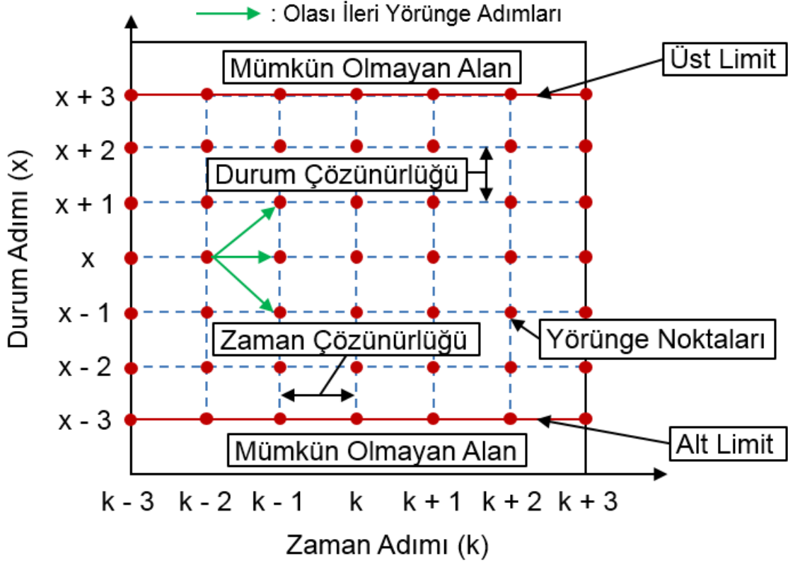
Şekil 3.3 Ayrılaştırılmış durum zaman uzayı
