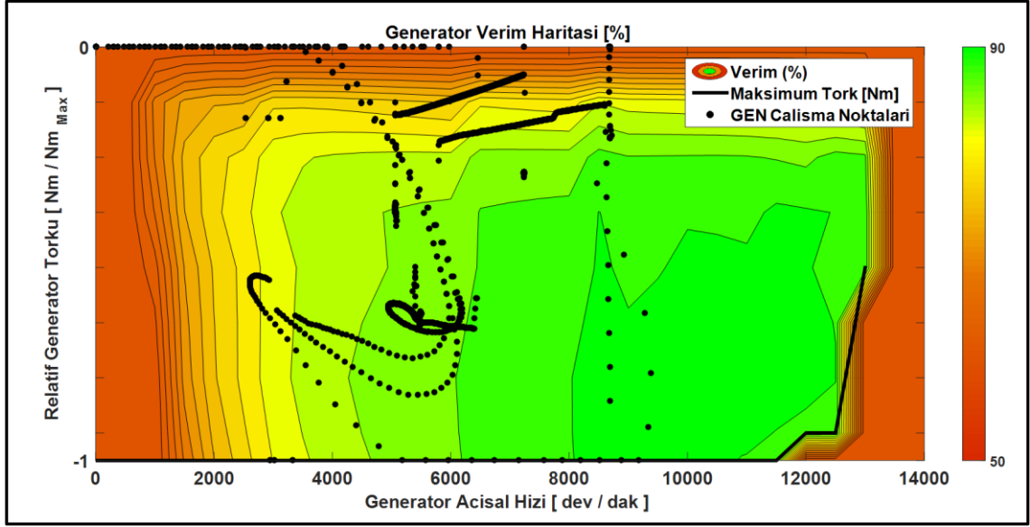
Şekil 4.5 NEDC çevriminde baz tahrik sistemi kural bazlı kontrolde GEN çalışma noktaları
