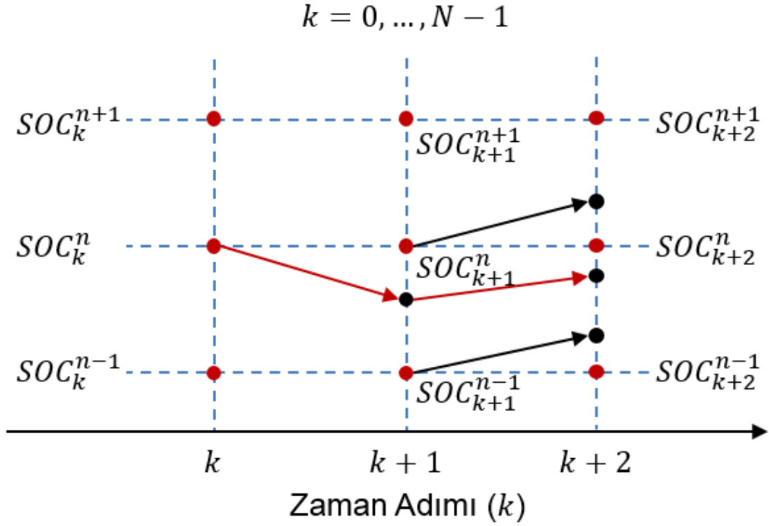
Şekil 3.6 İleriye dönük hesaplamada kullanılan interpolasyon
