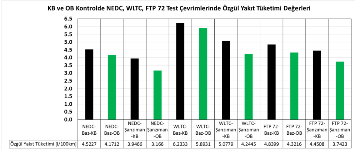
Şekil 4.57 Kural bazlı ve optimizasyon bazlı kontrolde NEDC, WLTC, FTP-72 test çevrimlerinde özgül yakıt tüketimi değerleri
