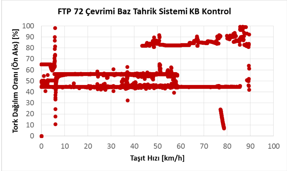
Şekil 4.37 FTP-72 çevriminde baz tahrik sistemi kural bazlı kontrolde ön aks tork dağılım oranları
