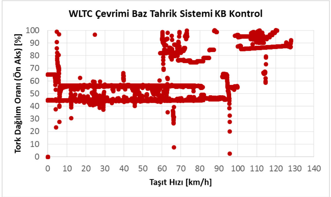
Şekil 4.20 WLTC çevriminde baz tahrik sistemi kural bazlı kontrolde ön aks tork dağılım oranı
