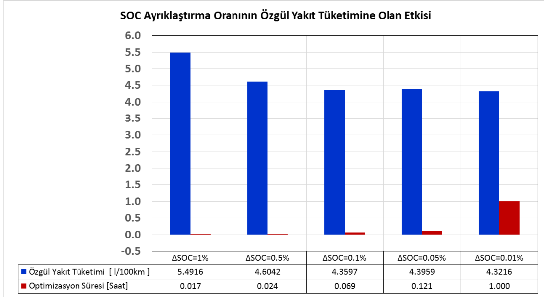
Şekil 4.56 FTP-72 çevriminde baz tahrik sistemi optimizasyon bazlı kontrolde SOC ayırıklaştırma oranının özgöl yakıt tüketimi ve optimizasyon süresi üzerindeki etkisi
