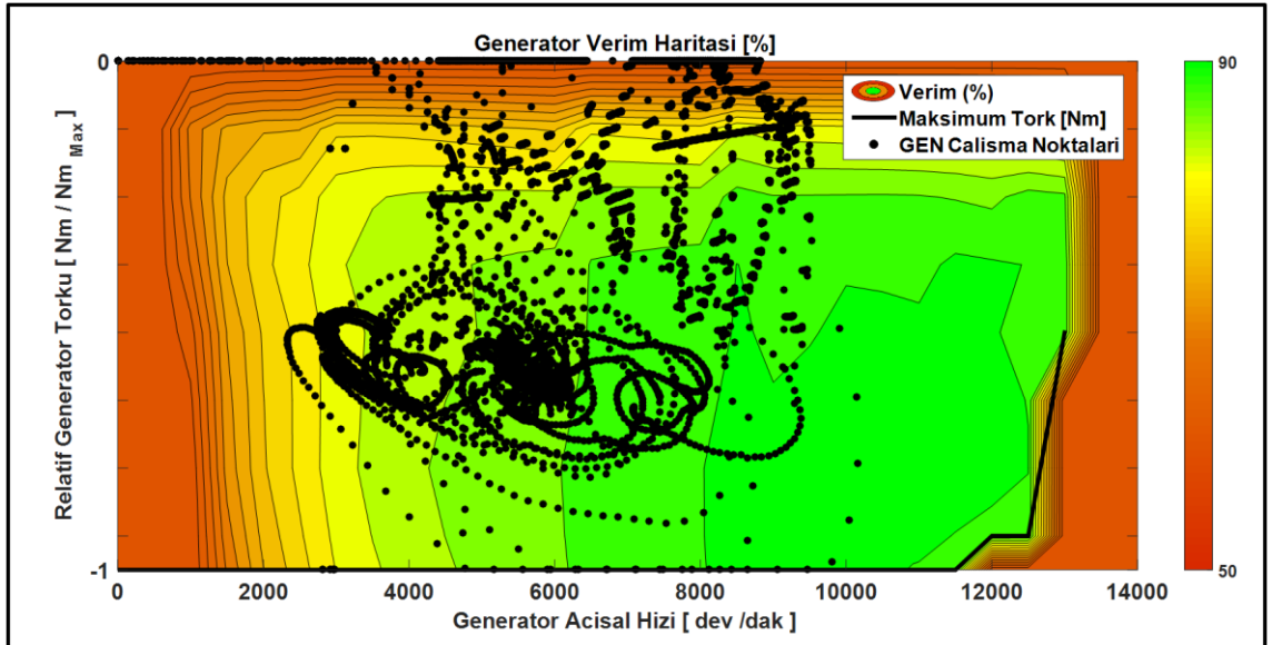
Şekil 4.22 WLTC çevriminde baz tahrik sistemi kural bazlı kontrolde GEN çalışma noktaları
