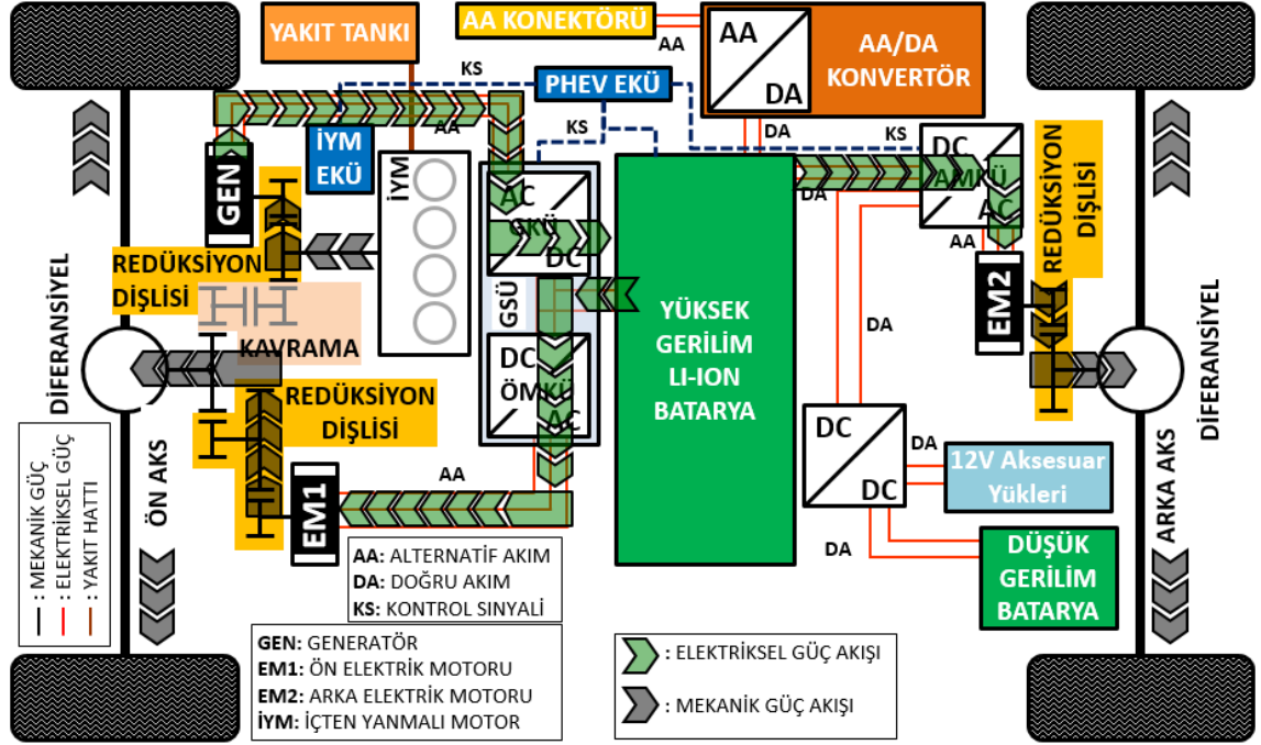
Şekil 2.4 Seri hibrit sürüş modunda güç akışı
