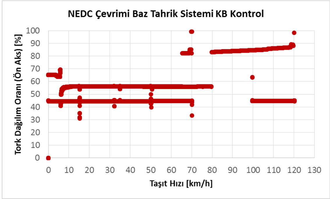
Şekil 4.3 NEDC çevriminde baz tahrik sistemi kural bazlı kontrolde ön aks tork dağılım oranı
