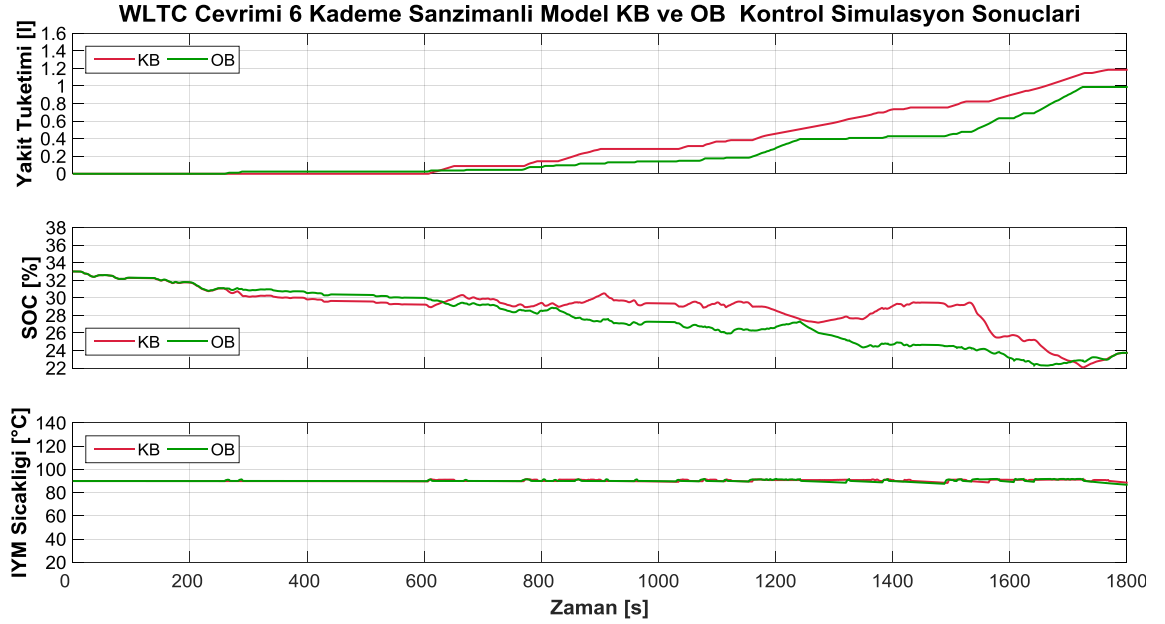
Şekil 4.28 WLTC çevriminde şanzımanlı tahrik sistemi yakıt tüketimi, SOC ve İYM sıcaklığı
