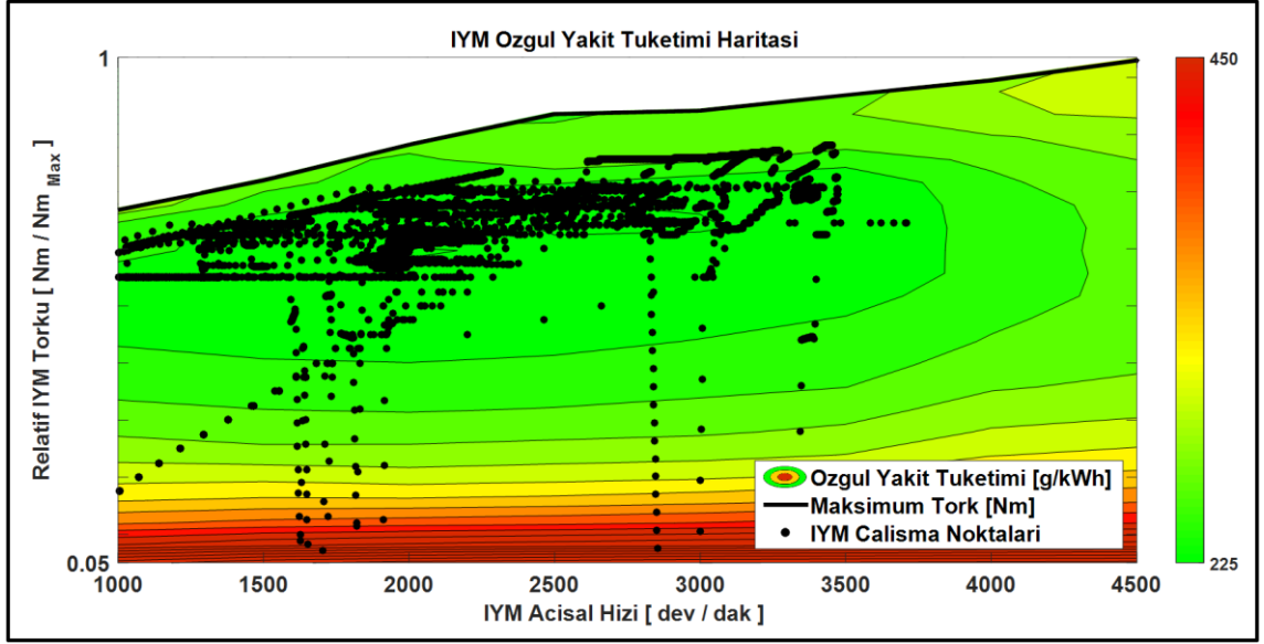
Şekil 4.21 WLTC çevriminde baz tahrik sistemi kural bazlı kontrolde İYM çalışma noktaları
