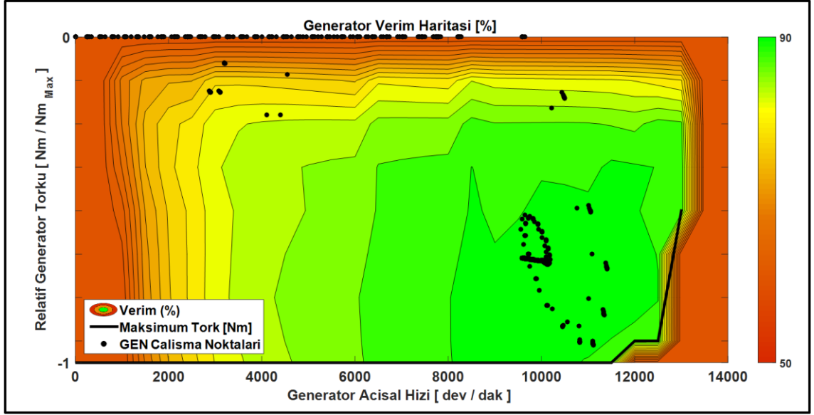
Şekil 4.42 FTP-72 çevriminde baz tahrik sistemi optimizasyon bazlı kontrolde GEN çalışma noktaları
