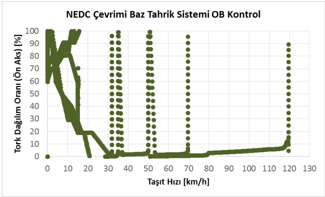
Şekil 4.6 NEDC çevriminde baz tahrik sistemi optimizasyon bazlı kontrolde ön aks tork dağılım oranları
