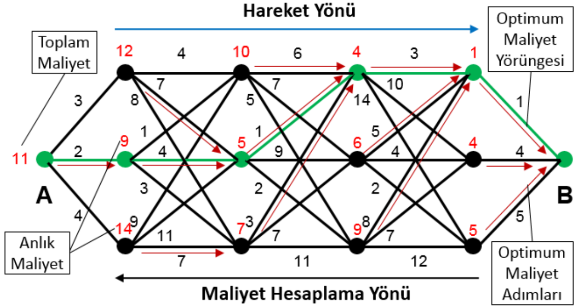
Şekil 3.2 Dinamik programlama optimum yörünge maliyeti
