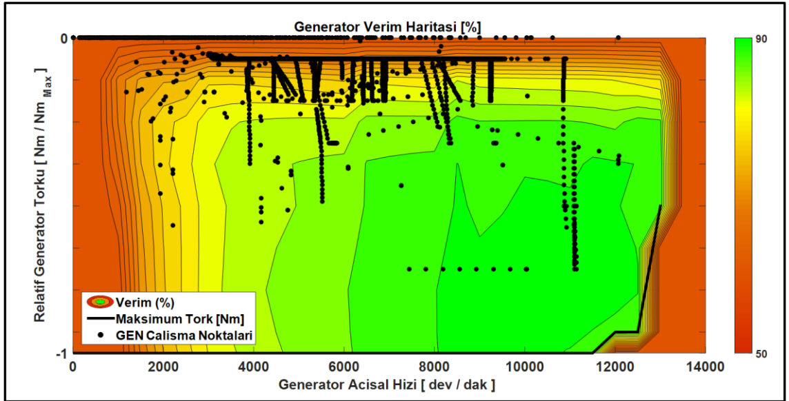
Şekil 4.34 WLTC çevriminde şanzımanlı tahrik sistemi optimizasyon bazlı kontrolde GEN çalışma noktaları
