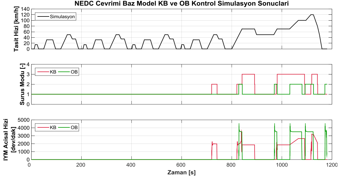
Şekil 4.1 NEDC çevriminde baz tahrik sistemi sürüş modu ve İYM açısal hızı
