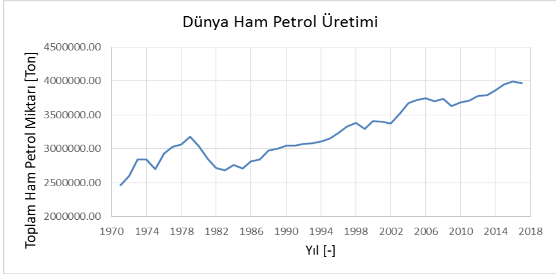
Şekil 1.1 Dünya ham petrol üretimi (1970 – 2018)
