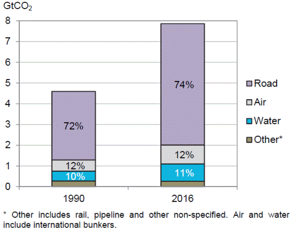
Şekil 1.3 Taşımacılık sektörü alt sektörlere göre CO 2 salınım miktarları (1990,2016)[15]
