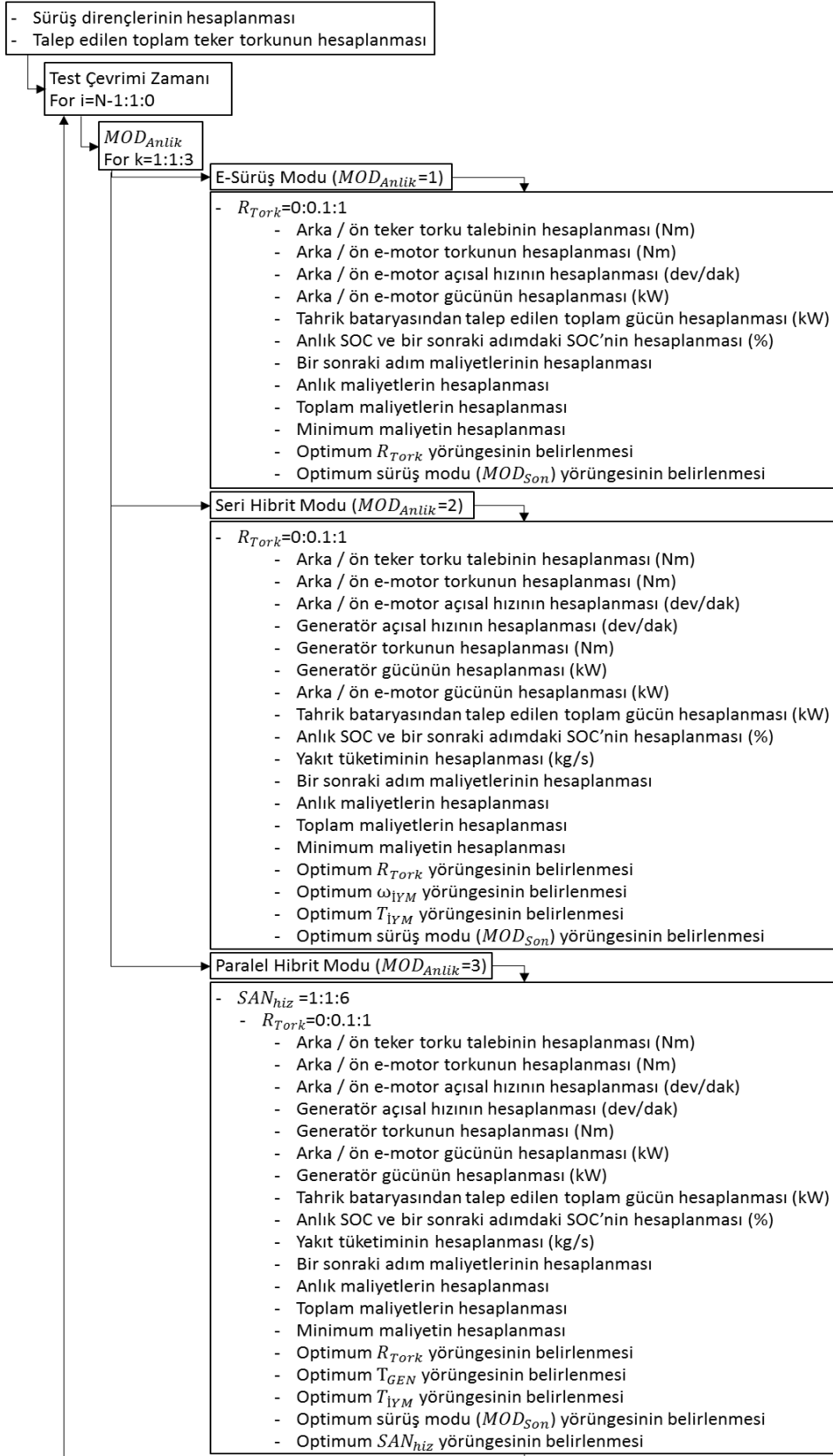
Şekil 3.10 Şanzımanlı tahrik sisteminde optimizasyon kodu algoritması
