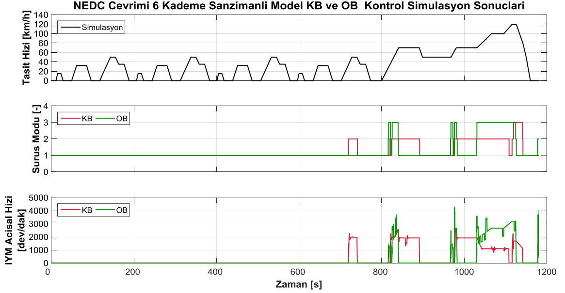
Şekil 4.9 NEDC çevriminde şanzımanlı tahrik sistemi sürüş modu ve İYM açısal hızı
