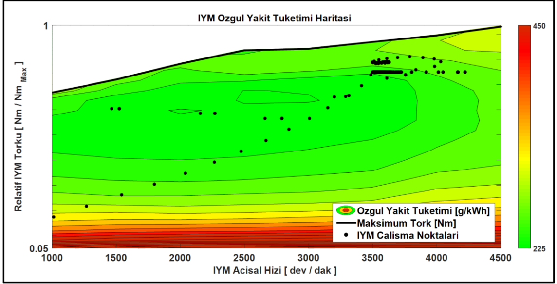
Şekil 4.24 WLTC çevriminde baz tahrik sistemi optimizasyon bazlı kontrolde İYM çalışma noktaları
