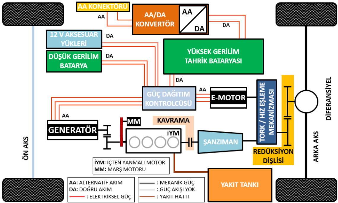
Şekil 1.14 Seri - paralel hibrit elektrikli taşıt mimarisi
