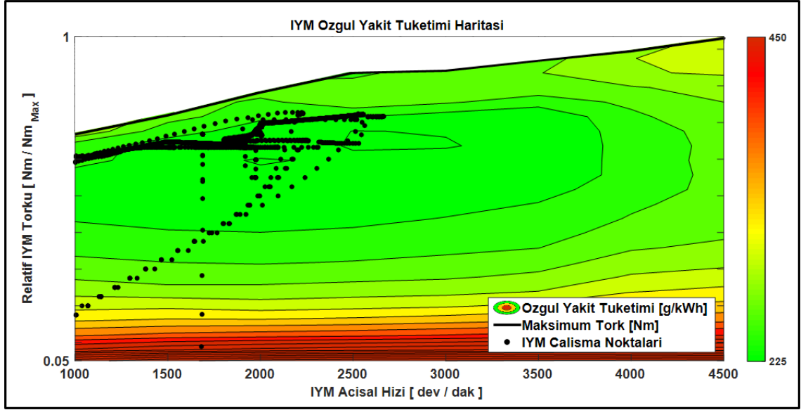
Şekil 4.13 NEDC çevriminde şanzımanlı tahrik sistemi kural bazlı kontrolde İYM çalışma noktaları
