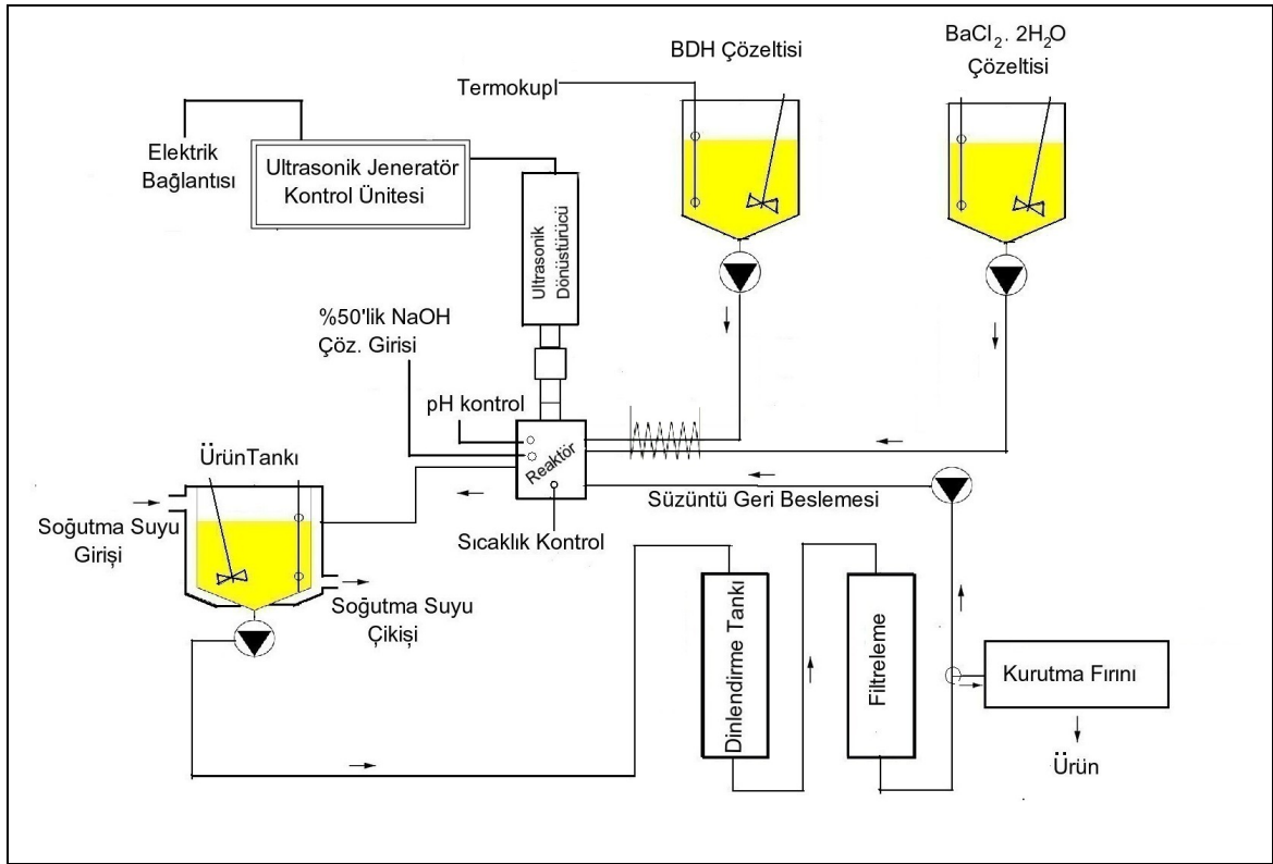
Şekil 6. 5 BDH kullanılan ultrasonik destekli sürekli üretim sistemi
