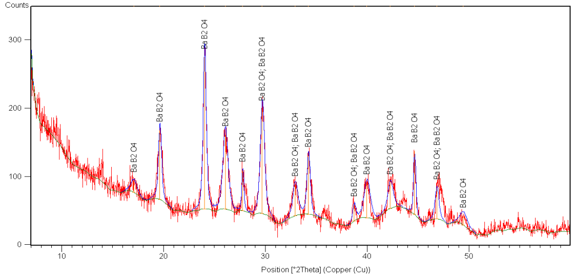
Şekil 7. 93 80 °C’de elde edilen ürünün XRD paterni (BK: SMT)
