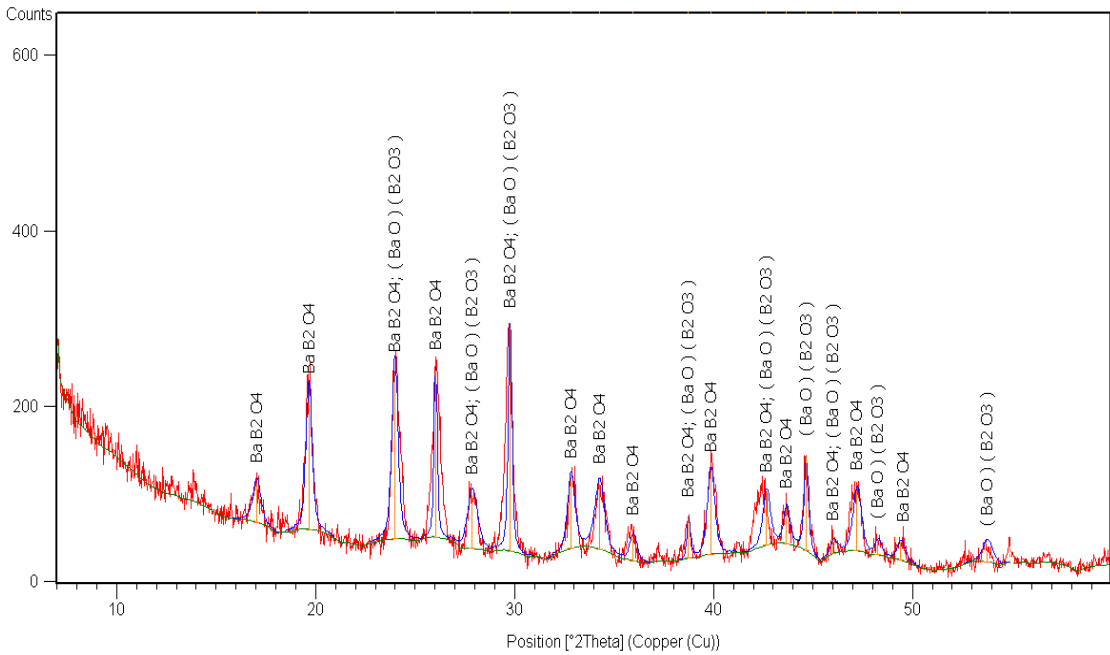
Şekil 7.47 pH 13 değerinde elde edilen ürünün XRD paterni (BK: BDH)
