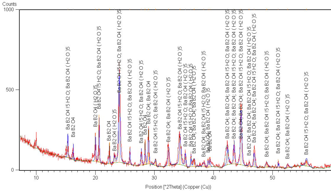
Şekil 7. 91 50 °C’de elde edilen ürünün XRD paterni (BK: SMT)
