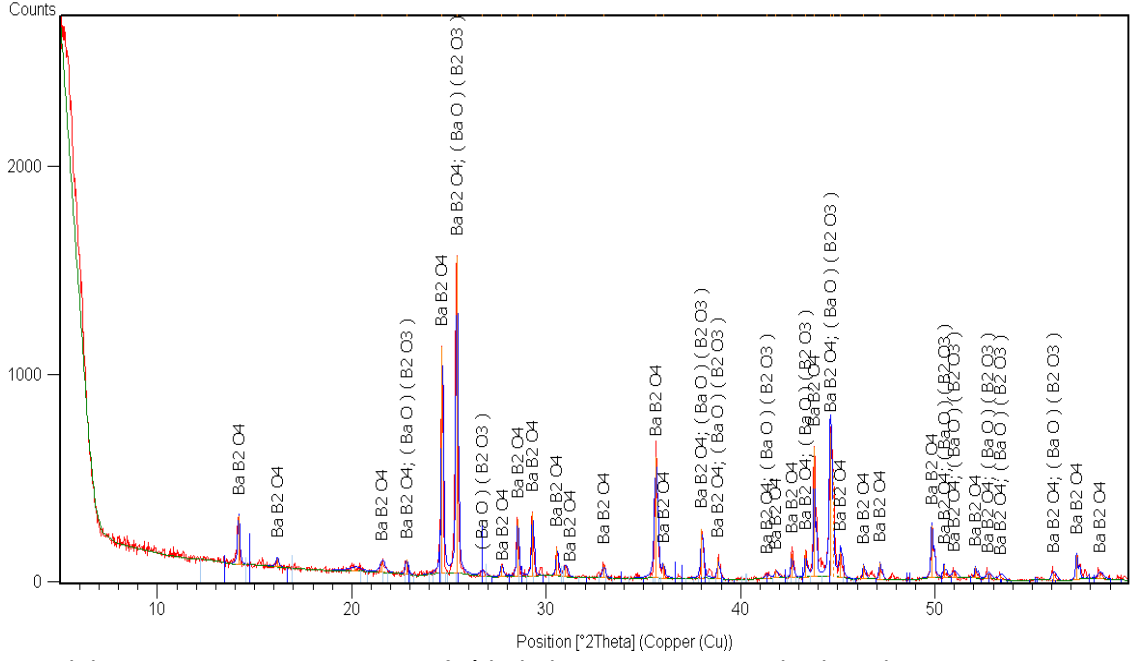
Şekil 7.40 D142 ürününün 630 °C’de kalsinasyonunun ardından alınan XRD paterni
