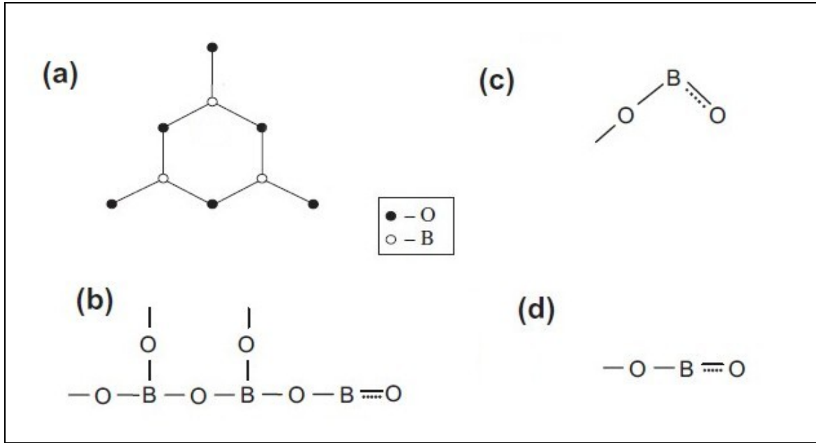
Şekil 2. 13 Çeşitli metaborat formları. Serbest \text{B}_3\text{O}_6^{3-} iyonu / metaborat halkası (a), üç elemanlı (\text{BO}_2)_3^{3-} anyonu zinciri (b), 'V' formundaki (c) ve düzlemsel yapıdaki(d) \text{BO}_2^{-1} anyonu [46]
