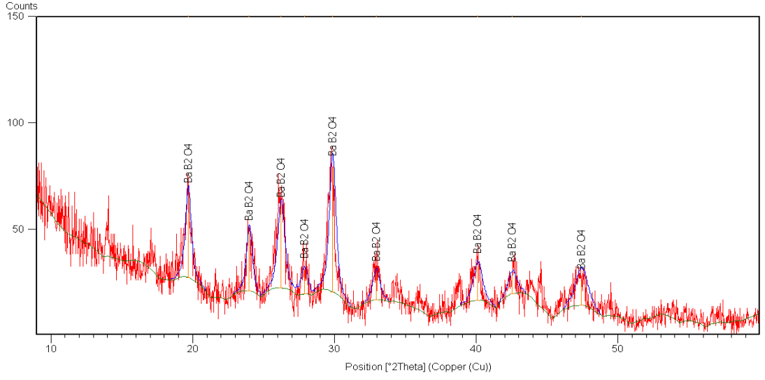
Şekil 7. 9 65 °C’de elde edilen ürünün XRD paterni (BK: H 3 BO 3 )
