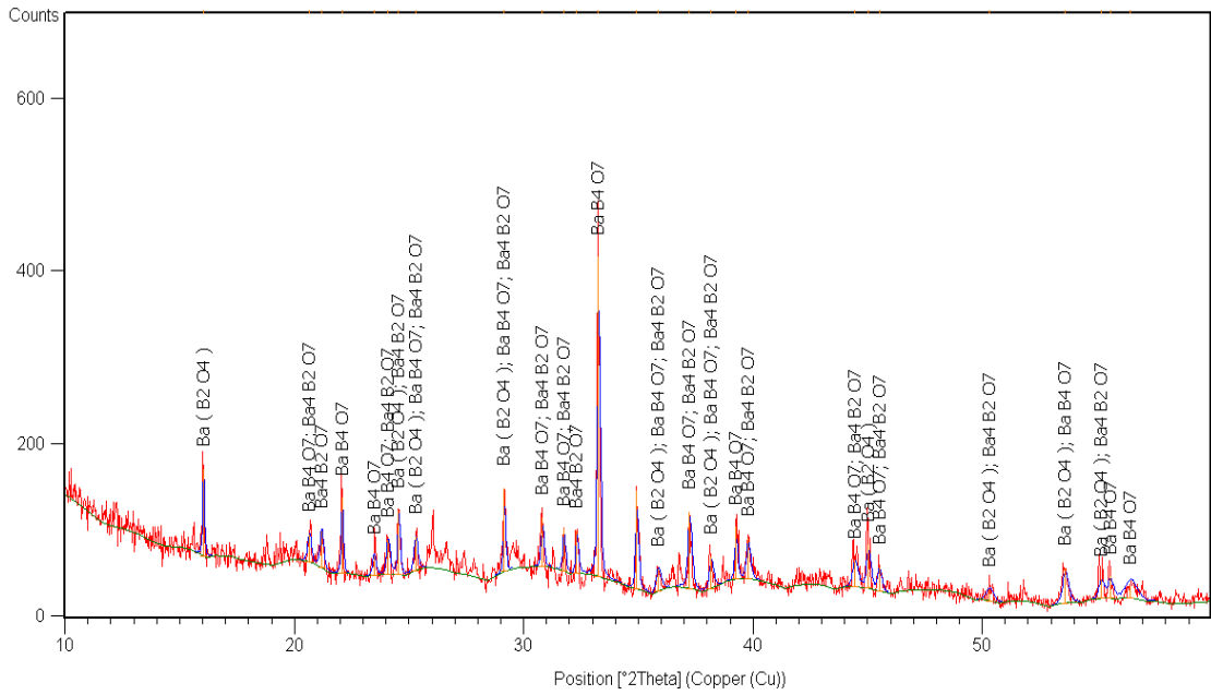
Şekil 7.135 270W ve 3dk'da elde edilen numunenin XRD paterni (BK:H 3 BO 3 )
