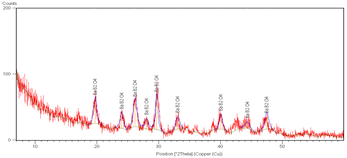
Şekil 7.58 5 dk.’da elde edilen ürünün XRD paterni (BK: BDH)
