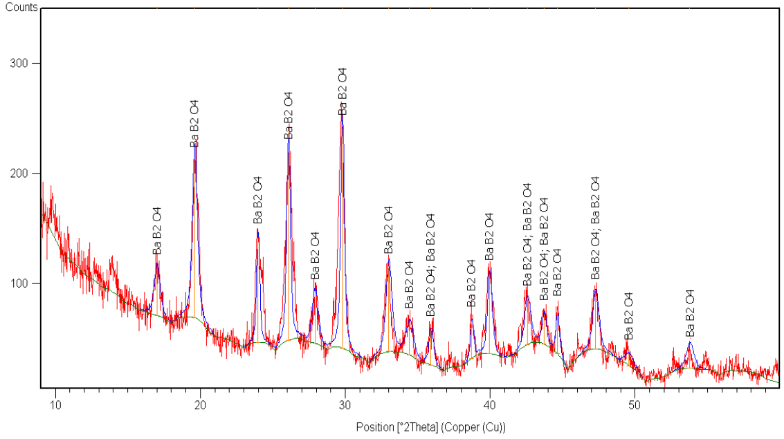
Şekil 7. 12 95 °C’de elde edilen ürünün XRD paterni (BK: H 3 BO 3 )
