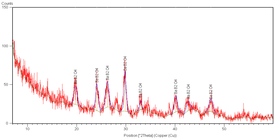
Şekil 7.25 5 sa. KS neticesinde elde edilen ürünün XRD paterni (BK: H 3 BO 3 )
