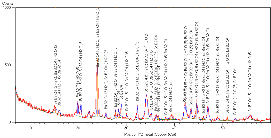
Şekil 7. 90 45 °C’de elde edilen ürünün XRD paterni (BK: SMT)
