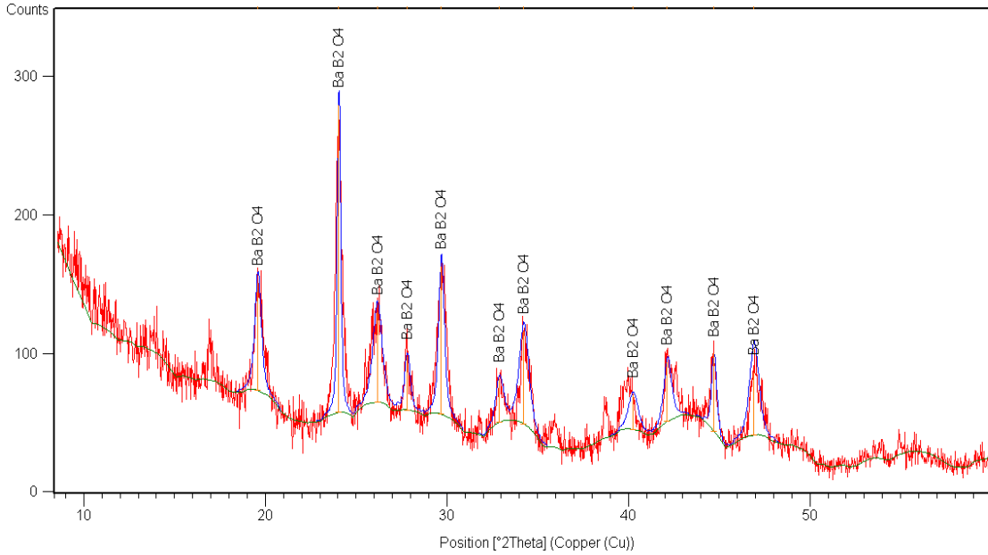
Şekil 7. 102 25 dk.'da elde edilen ürünün XRD paterni (BK: SMT)
