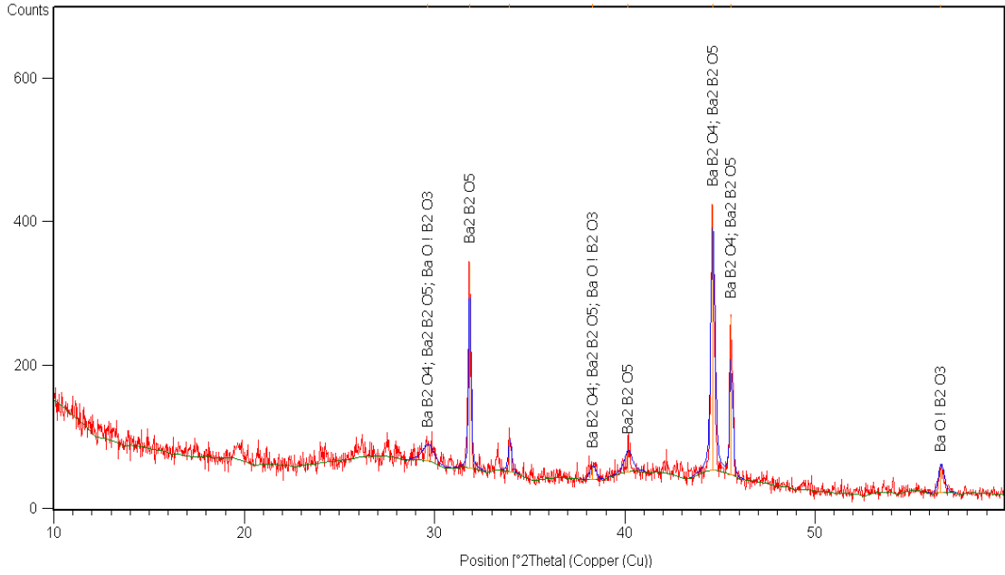
Şekil 7. 134 270W ve 2dk'da elde edilen numunenin XRD paterni (BK:H 3 BO 3 )
