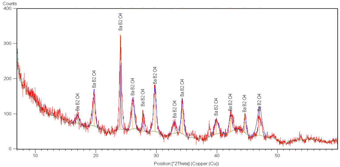
Şekil 7. 94 90 °C’de elde edilen ürünün XRD paterni (BK: SMT)
