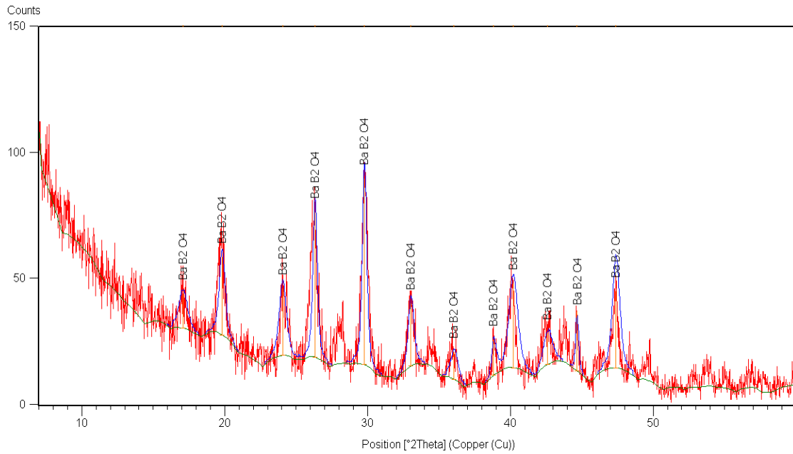
Şekil 7.28 2,5:1 H 3 BO 3 :BKD molar oranlı reaksiyon ürününün XRD paterni
