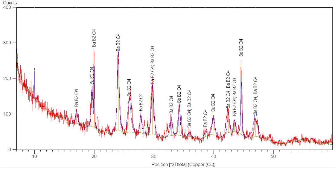
Şekil 7. 92 65 °C’de elde edilen ürünün XRD paterni (BK: SMT)
