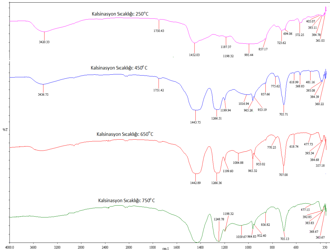
Şekil 7. 122 Farklı sıcaklıklarda kalsine edilmiş D156 numunesinin FTIR sonucu
