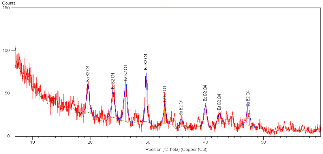
Şekil 7.24 4 sa. KS neticesinde elde edilen ürünün XRD paterni (BK: H 3 BO 3 )
