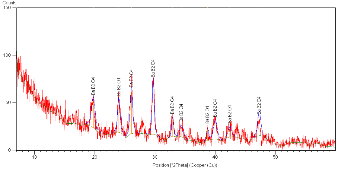
Şekil 7. 23 3 sa. KS neticesinde elde edilen ürünün XRD paterni (BK: H 3 BO 3 )
