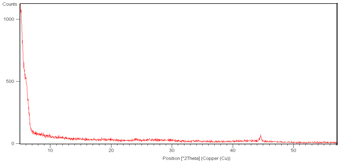
Şekil 7. 44 pH 10 değ rinde elde edilen  r n n XRD paterni (BK: BDH)
