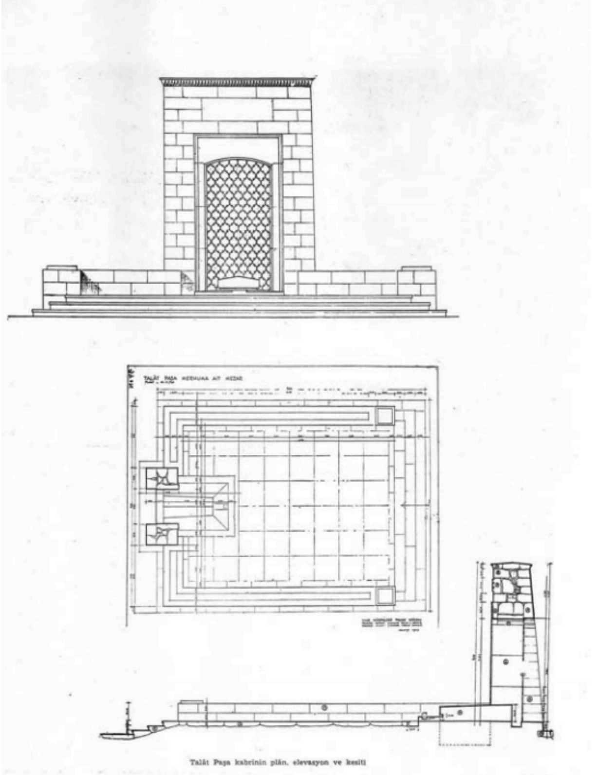
Şekil 3.111 Sadrazam Talat Paşa'nın Mezarı [280]
