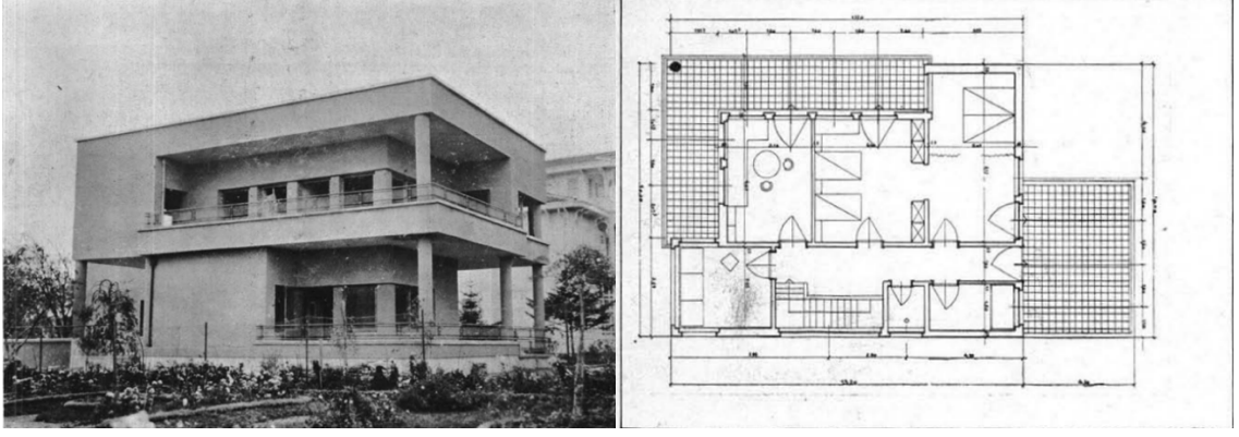
Şekil 3.76 İstanbul Suadiye Doktor İhsan Sami Garan Evi [239]
