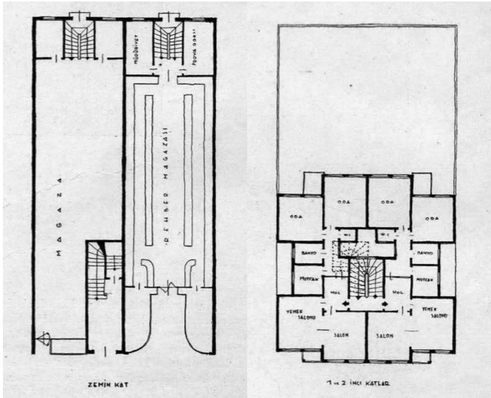
Şekil 3.134 Anafartalar Caddesinde bir Kira Evi [317]
