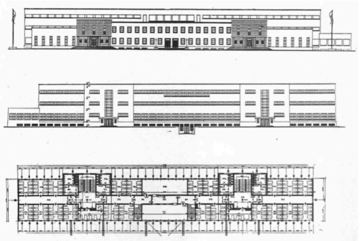
Şekil 3.139 Ankara Polis Jandarma Mektebi [321]
