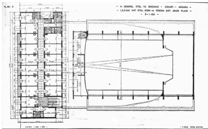
Şekil 3.42 Ankara Nur Sinema ve Oteli [167]
