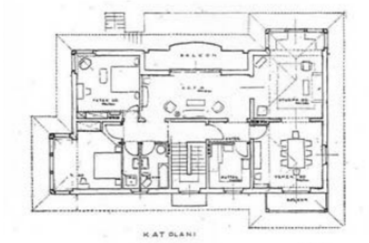
Şekil 3.242 Çifte Evler Projesi Evi [446]
