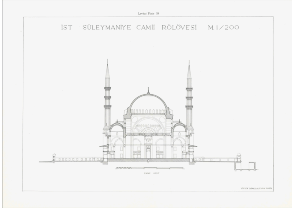
Şekil 3.235 İstanbul Süleymaniye Cami Rölövesi [442]
