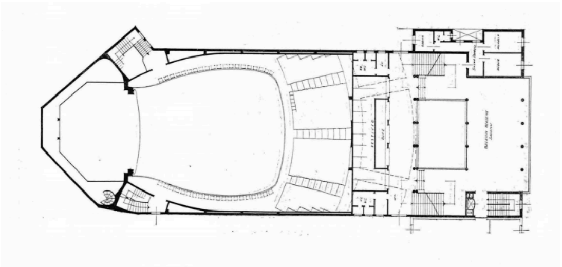
Şekil 3.40 Ankara Büyük Sinema [165]
