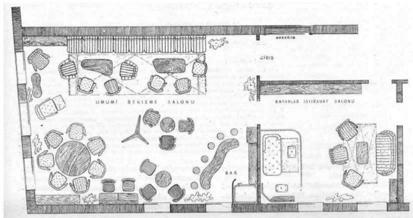
Şekil 3.223 Antaş Havacılık uçak yolcu bekleme salonu [426]
