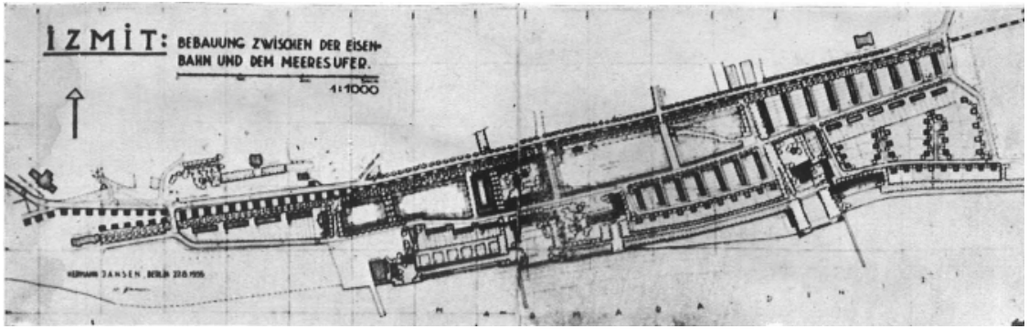
Şekil 3.46 İzmit İmar Planı [180]
