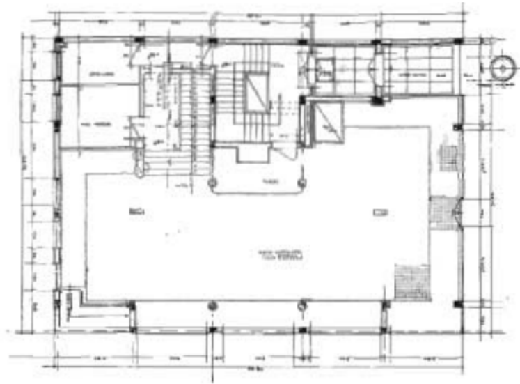
Şekil 3.68 Ankara Koç Hanı [223]
