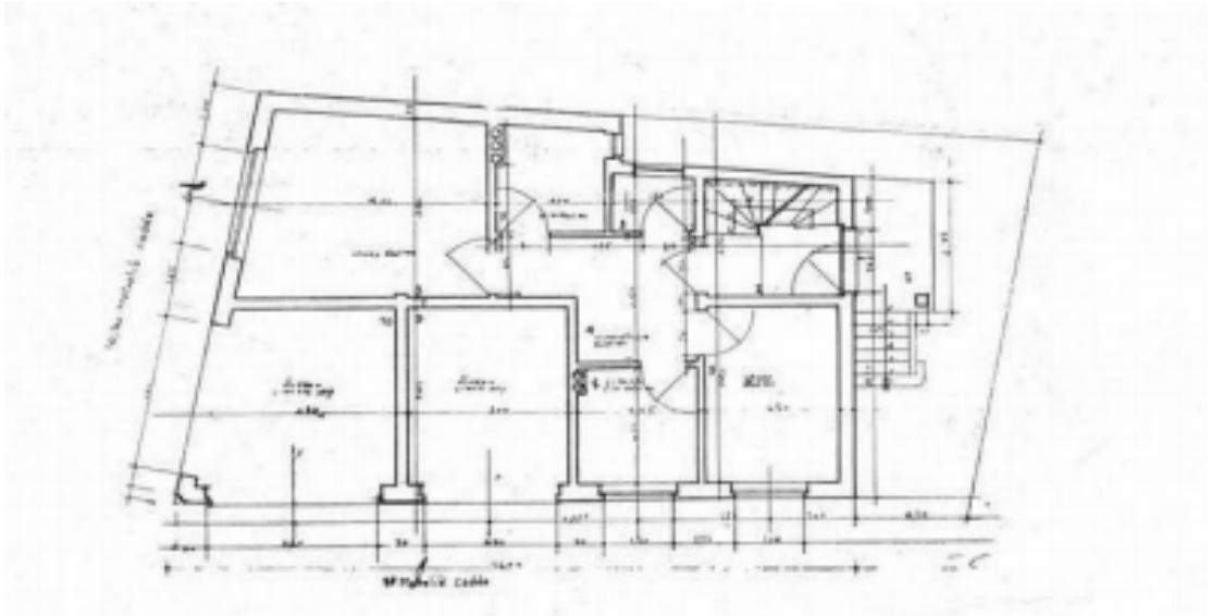
Şekil 3.91 Muhittin Bey Evi-Kadıköy [258]
