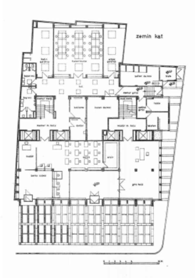
Şekil 3.73 Akbank Genel Müdürlük Binası [235]
