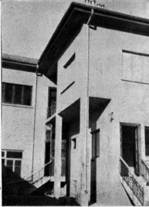
Şekil 3.123 Eskişehir’de Bay Salahattin Evi [292]
