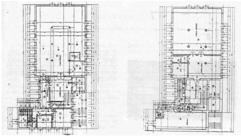
Şekil 3.50 İstanbul Maliye Binası Mercan Şubesi [189]
