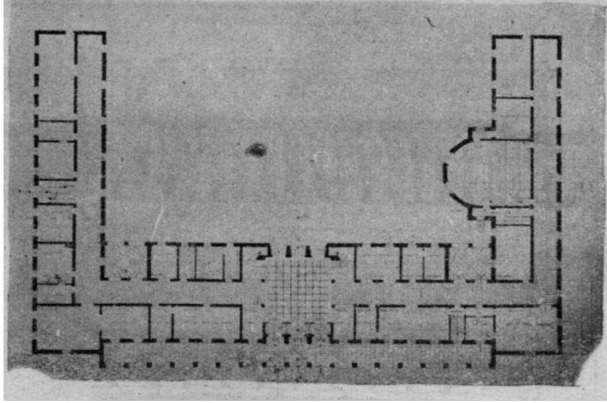
Şekil 3.37 Adana Adalet Sarayı Binası Müsabakası [161]
