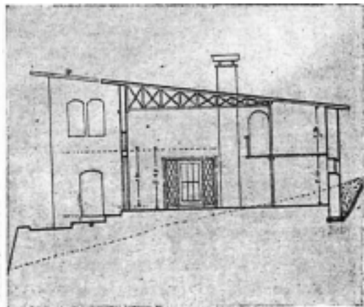
Şekil 3.214 Elmadag kayakevi (Hidayet Nejat Erer ile) [417]
