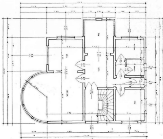
Şekil 3.164 İstanbul Kadıköy'de Ev [351]
