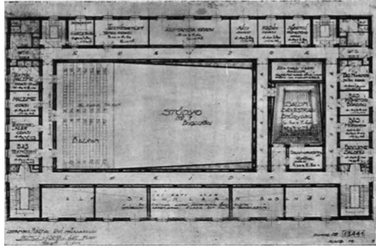
Şekil 3.13 İstanbul Radyoevi Proje Müsabakası Paftaları [114]
