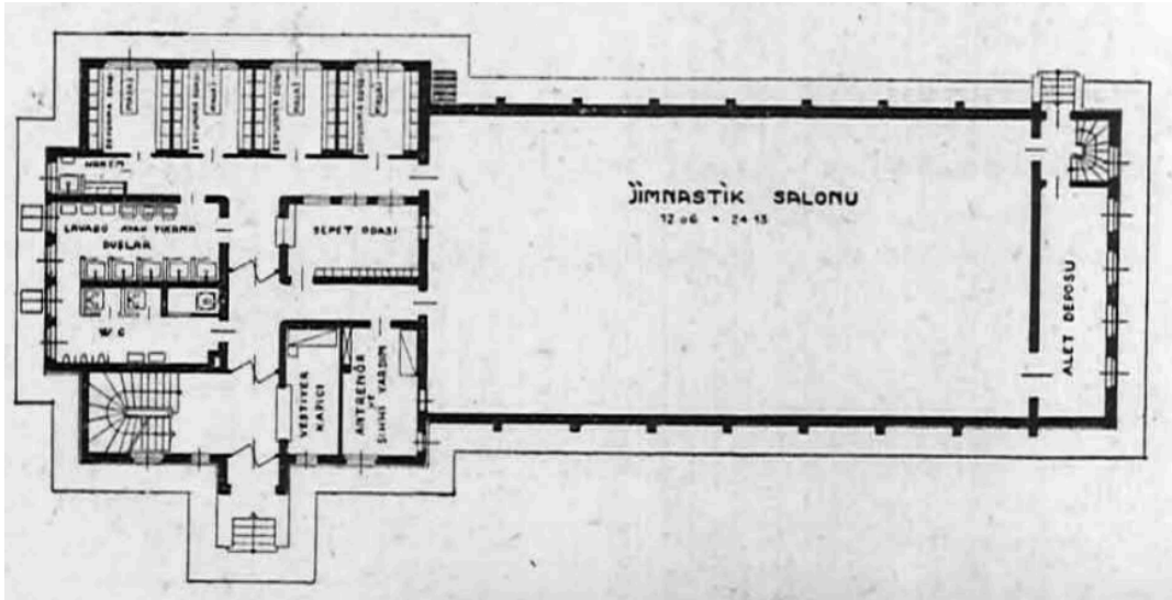
Şekil 3.127 İstanbul Karag mr k Kapalı Jimnastik Salonu [305]
