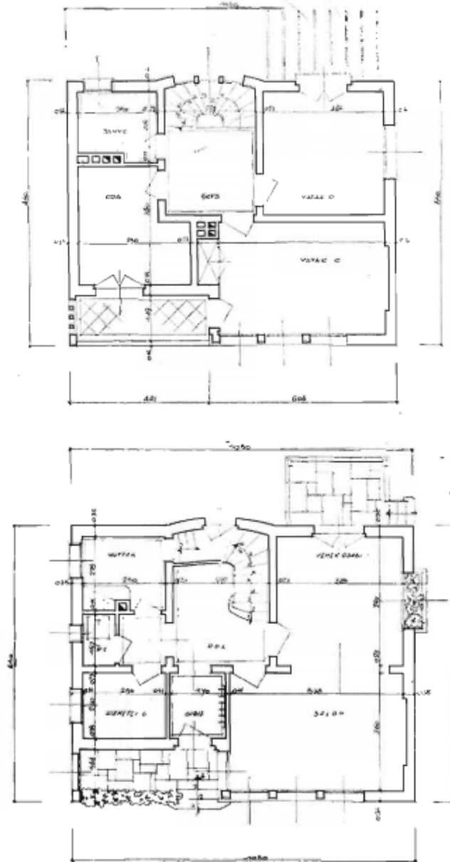
Şekil 3.39 Ankara İş Bankası Piyango Evi [164]
