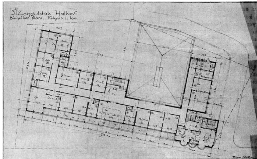
Şekil 3.87 Zonguldak Halk Evi Binası [254]
