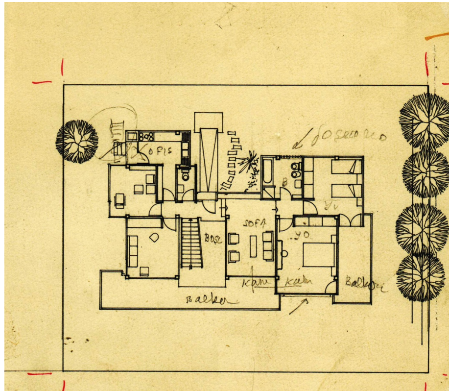
Şekil 3.208 Pendik Adnan Kunt Evi çizimleri [412]
