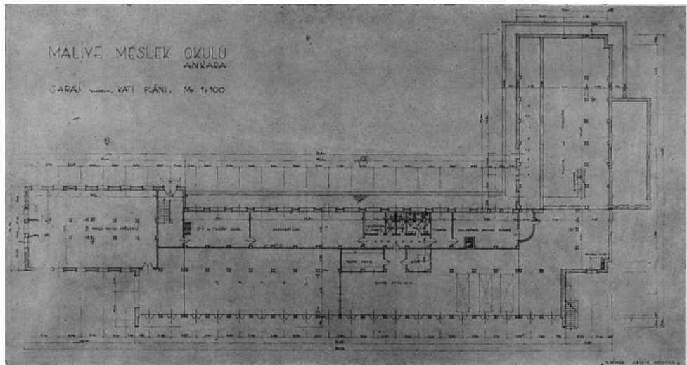
Şekil 3.41 Ankara Maliye Meslek Okulu [166]
