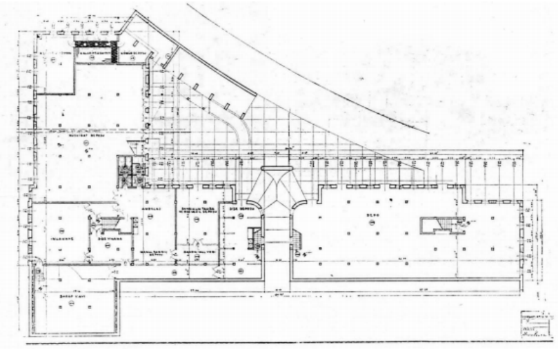
Şekil 3.204 İnhisarlar Umum Müdürlüğü depo ve imalathanesi [405]
