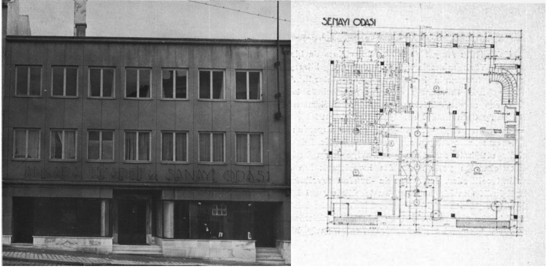
Şekil 3.65 Ankara Sanayi ve Ticaret Odası Binası [220]
