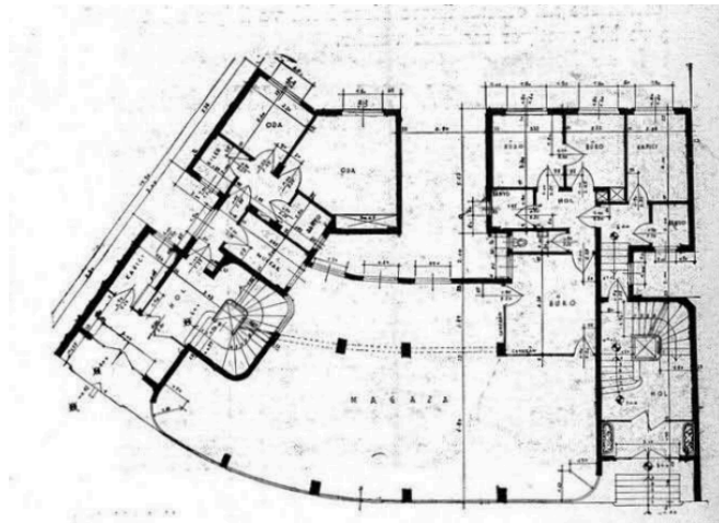
Şekil 3.167 İstanbul Taksim, Doğu Apartmanı (Mustafa Can ile)[353]
