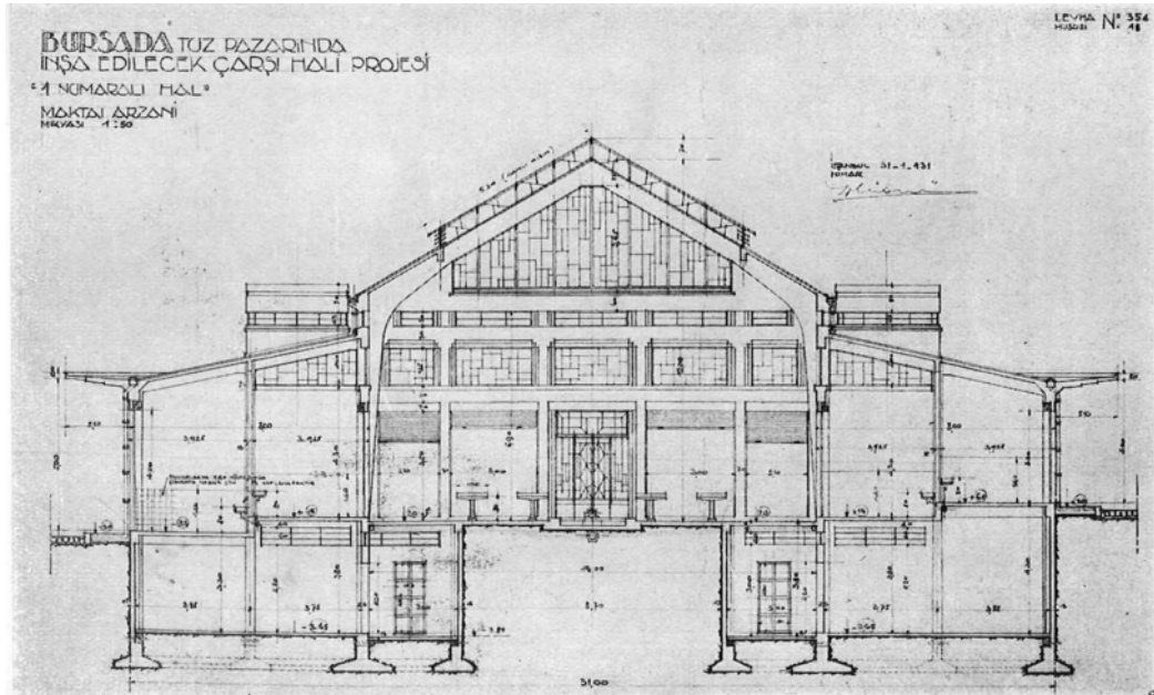
Şekil 3.24 Bursa'da İnşa Edilecek Hal Binası Projesi [125]
