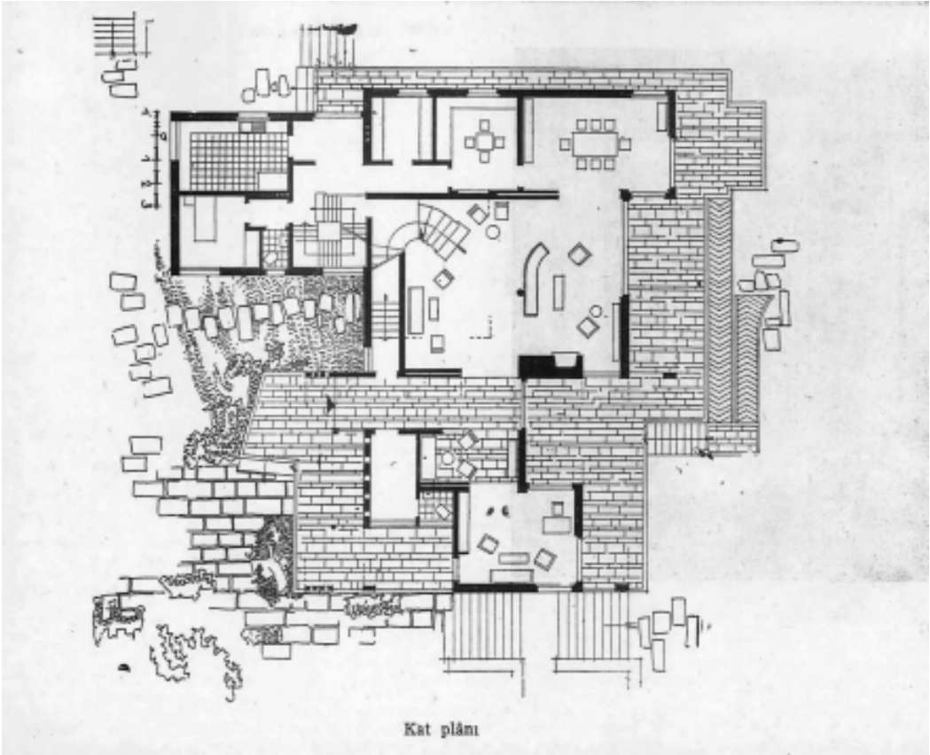
Şekil 3.186 Büyük Adada Sadıkoğlu Villâsı [379]
