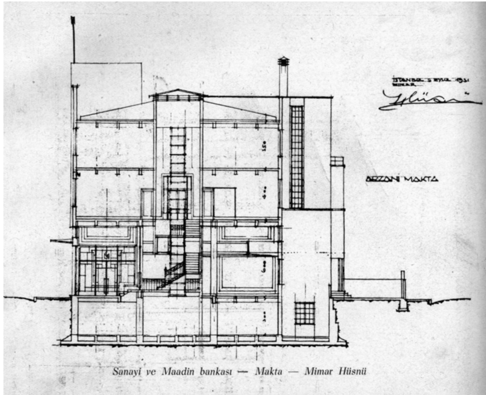
Şekil 3.22 Ankara Sanayi ve Maadin Bankası Müsabaka Paftaları [124]
