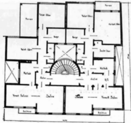
Şekil 3.150 Ankara'da bir Kira Evi [336]
