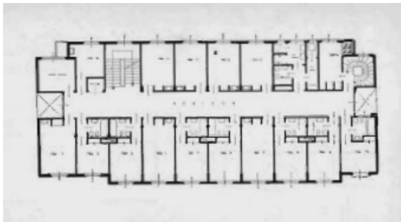
Şekil 3.131 Ankara Yeni Şehir oteli [310]
