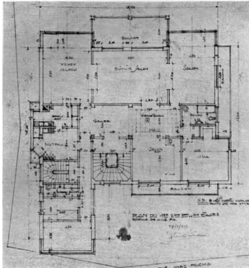
Şekil 3.25 Ayazpaşa Mühendis İbrahim Galip B. Apartmanı [126]
