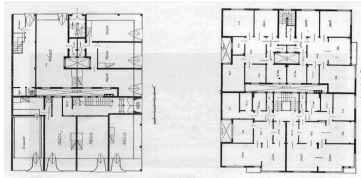
Şekil 3.150 Ankara'da bir Kira Evi [336]
