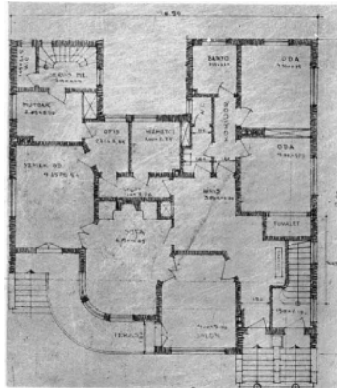
Şekil 3.121 Ankara'da Bir Ev [291]
