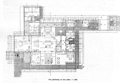
Şekil 3.80 Makbule Atadan Köşkü [243]
