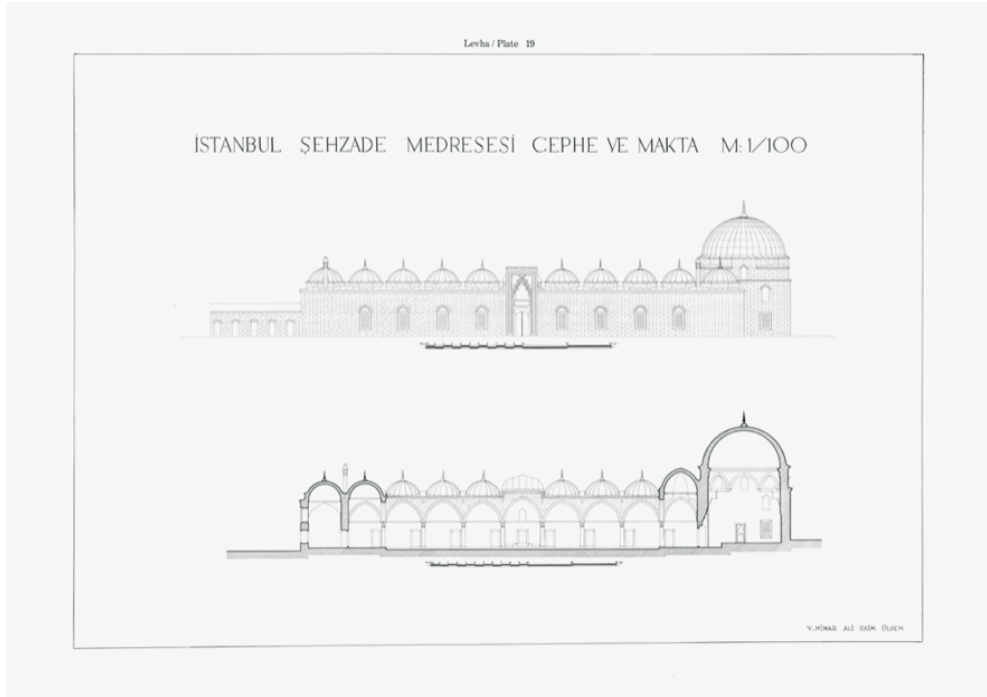
Şekil 3.236 İstanbul Şehzade Medresesi Rölövesi [443]
