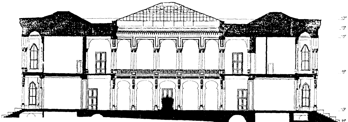
Şekil : 2.21- Divanhane Binası Kesit ve Görünüşler (Merkez,...)
