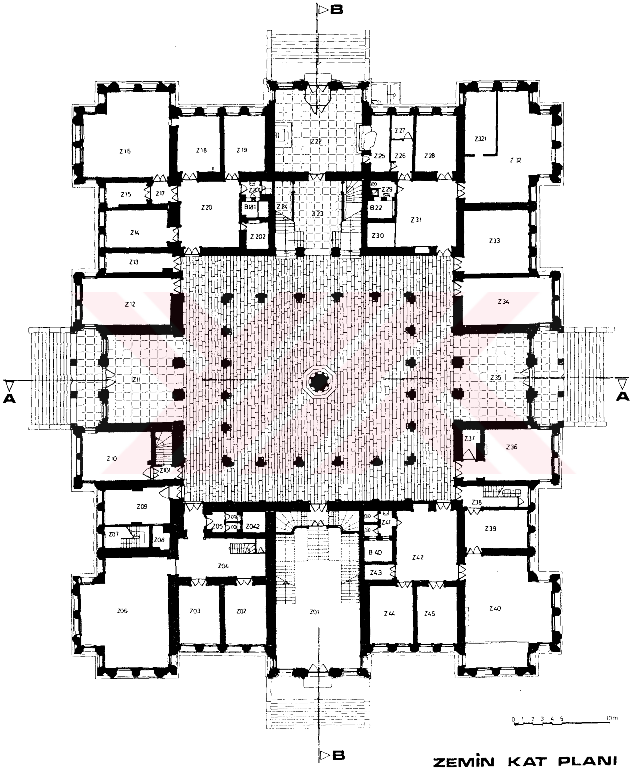
Şekil : 2.19- Divanhane Binası, Zemin Kat Planı, (Merey,...)
