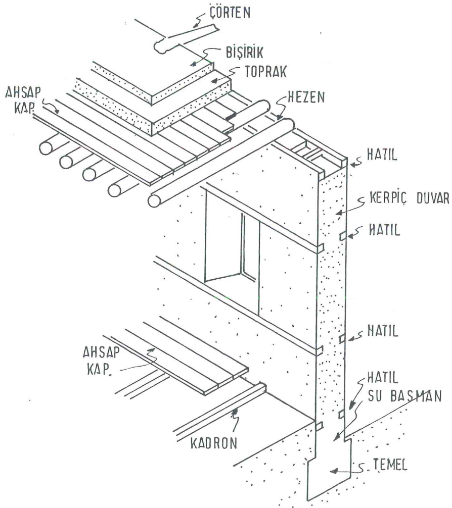
Resim 8. Sistem Detayı
